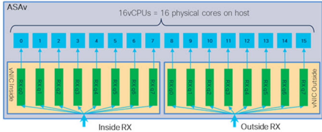
图 4: 16 核 ASA 的 RSS RX 队列
