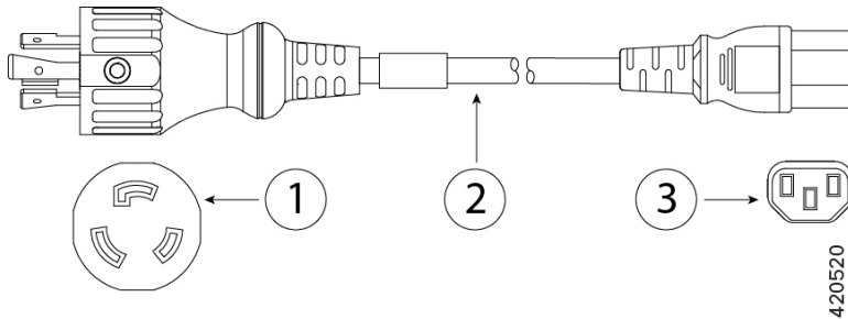
图 27: 日本 CAB-L620P-C13-JPN
