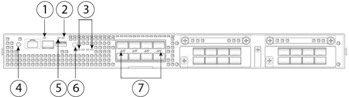
图 6: 前面板 LED
