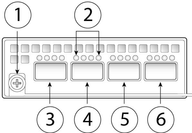
图 9: FPR4K-NM-4X40G
