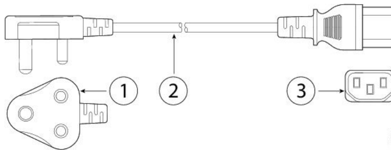
图 23: 印度 CAB-250V-10A-ID
