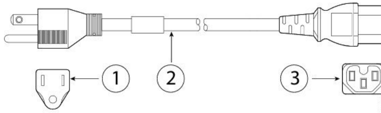
图 29: 北美 CAB-TA-NA
