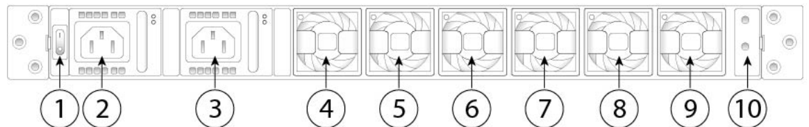
图 7: Firepower 4100 后面板
