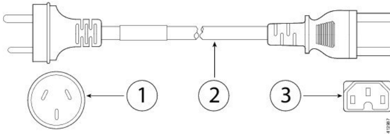
图 20: 中国 CAB-9K10A-CH
