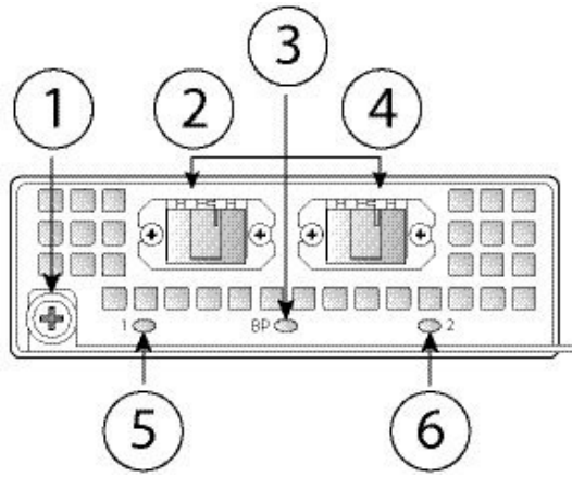
图 11: FPR4K-NM-2X40G-F
