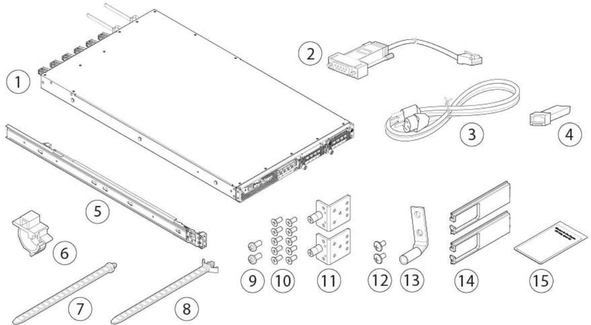
图 2: Firepower 4100 装箱单
