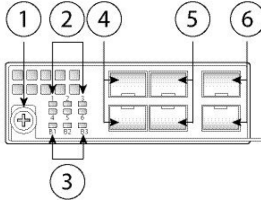
图 12: FPR4K-NM-6X1SX-F、FPR4K-NM-6X10SR-F、FPR4K-NM-6X10LR-F
