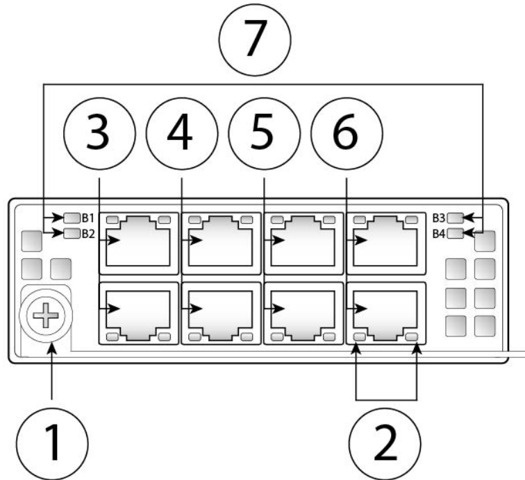
图 10: FPR-NM-8X1G-F
