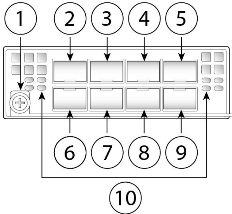
图 8: FPR4K-NM-8X10G
