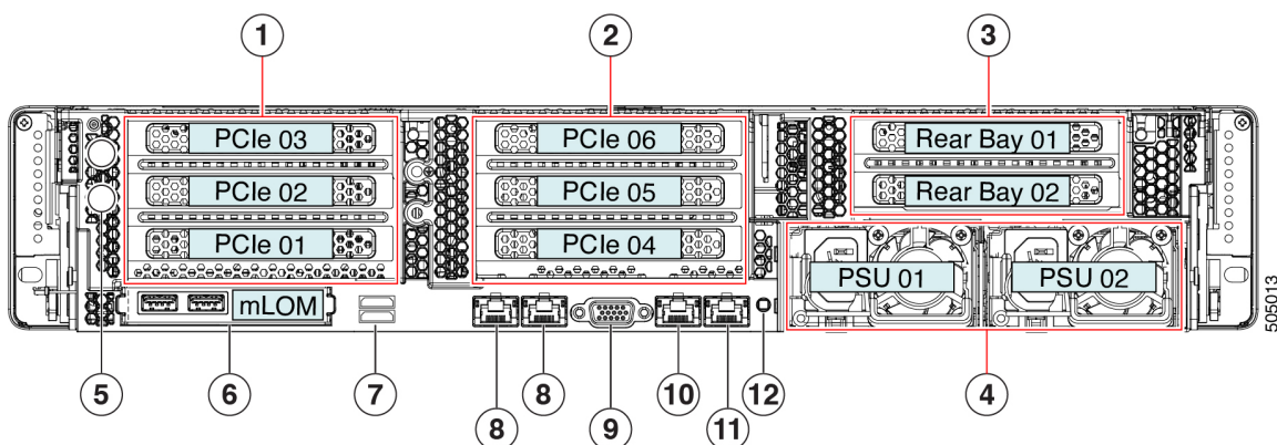
图 6: 后面板
