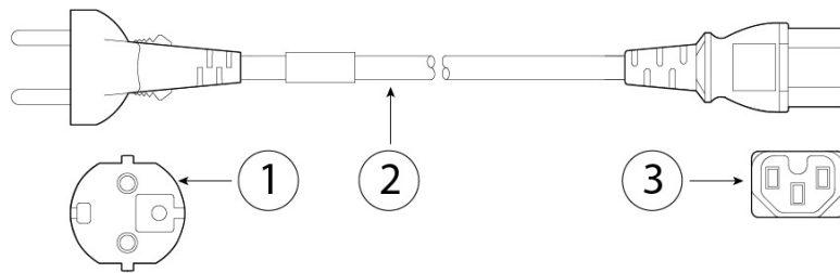
图 15: 欧洲 (CAB-9K10A-EU)
