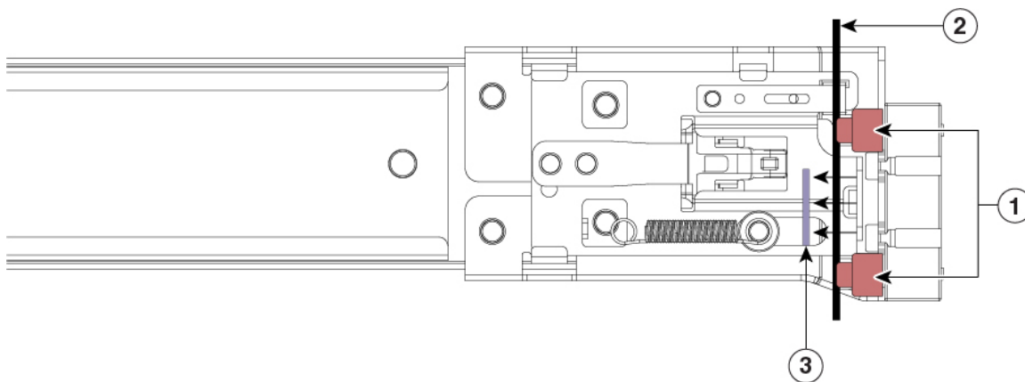
图 29: 前紧固装置，前端内侧
