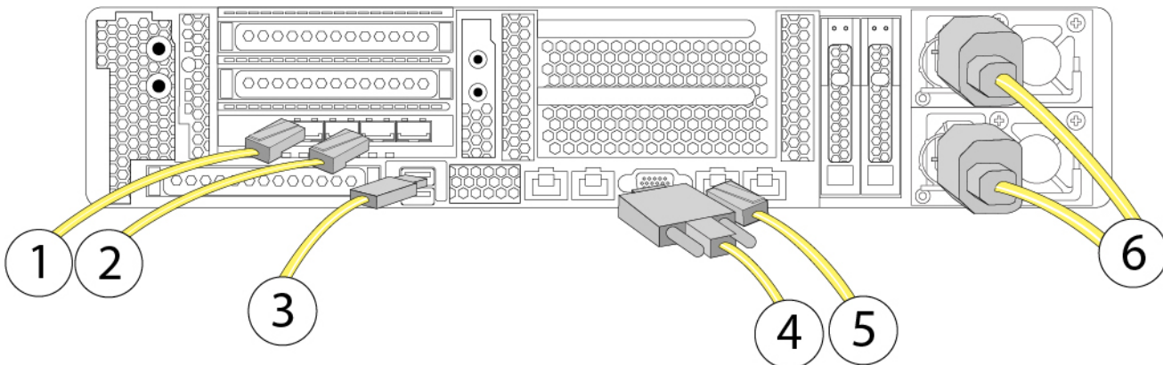
图 31: 电缆连接
