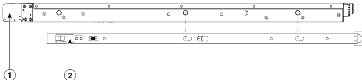
图 28: 将内滑轨固定到机箱的侧面
