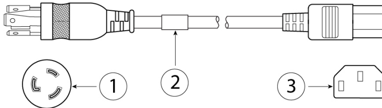
图 24: 北美 (CAB-AC-L620-C13)
