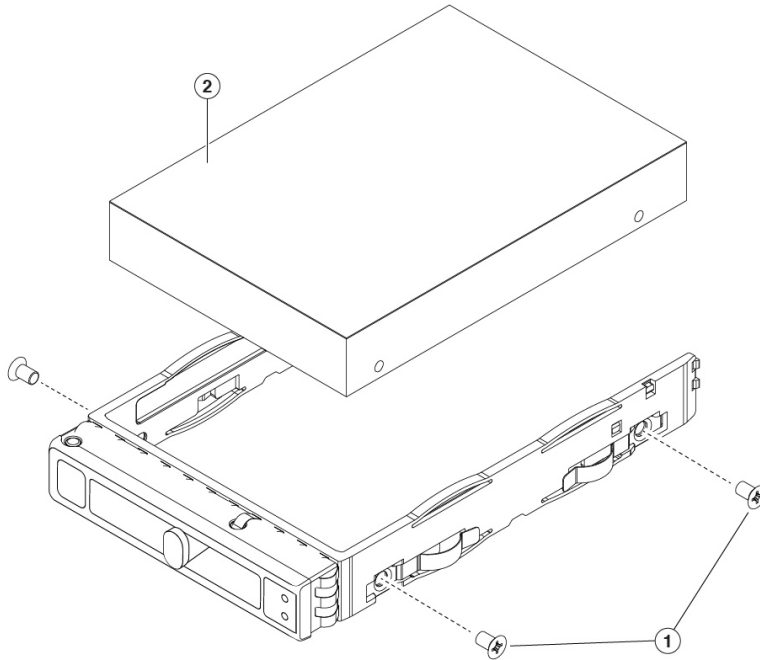
图 33: 拆卸驱动器托架
