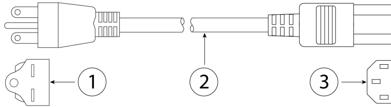
图 23: 北美 (CAB-N5K6A-NA)
