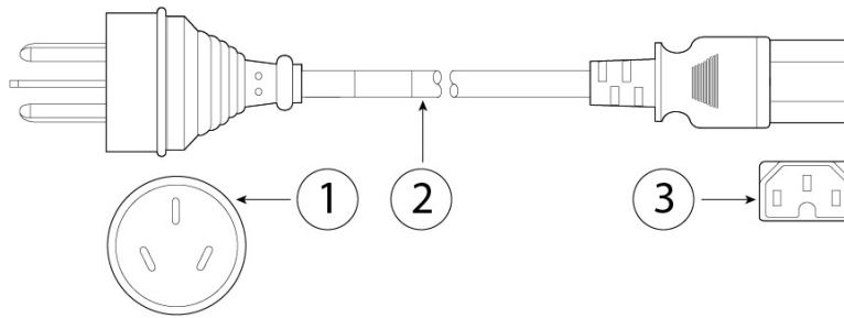
图 9: 澳大利亚 (CAB-9K10A-AU)
