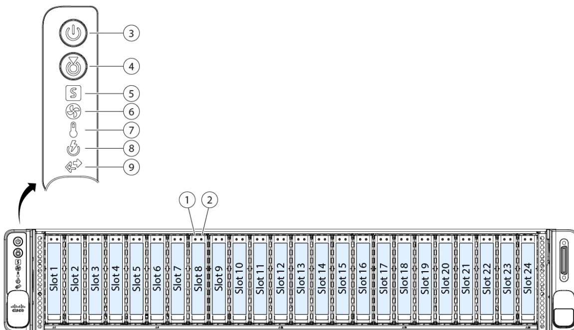
图 5: 前面板 LED 及其状态
