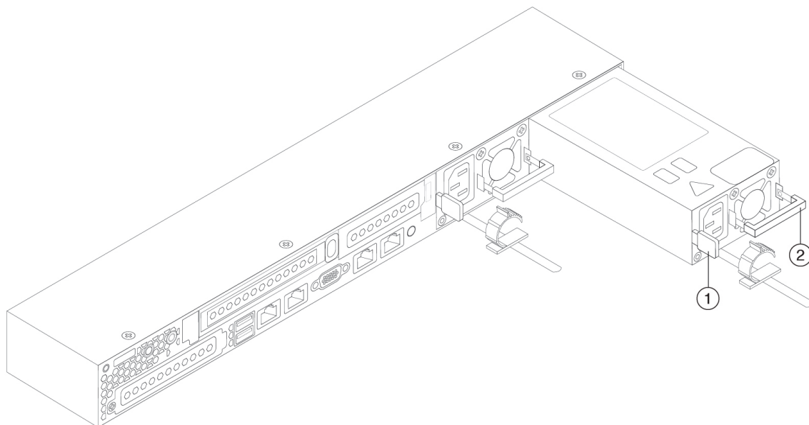
图 34: 拆卸和更换交流电源
