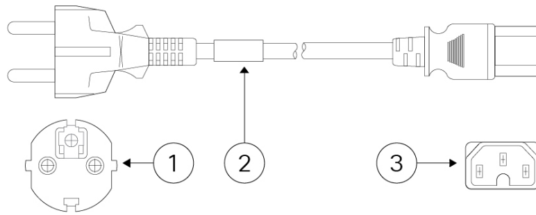
图 21: 韩国 (CAB-9K10S-KOR)
