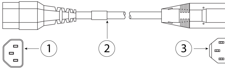
图 11: 机柜跳线 (CAB-C13-C14-2M)
