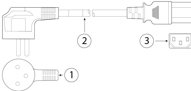
图 17: 以色列 (CAB-250V-10A-IS)
