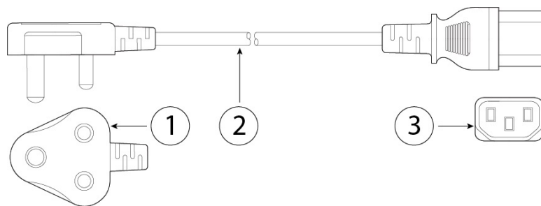
图 16: 印度 (CAB-250V-10A-ID)
