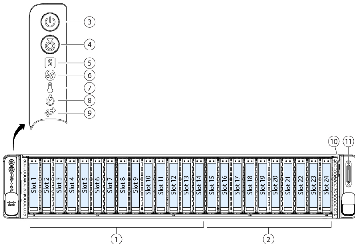
图 4: Cisco Secure Endpoint PC4000 前面板
