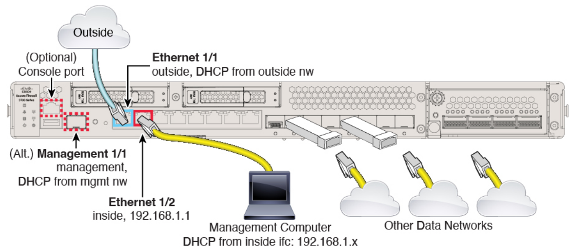
图 2: Secure Firewall 3100 的布线
