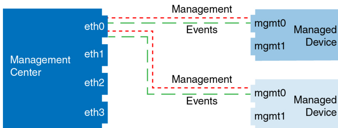
图 4: Cisco Secure Firewall Management Center 上的单个管理接口
