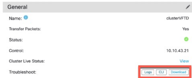
图 6: 故障排除
