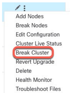
图 18: 中断集群
