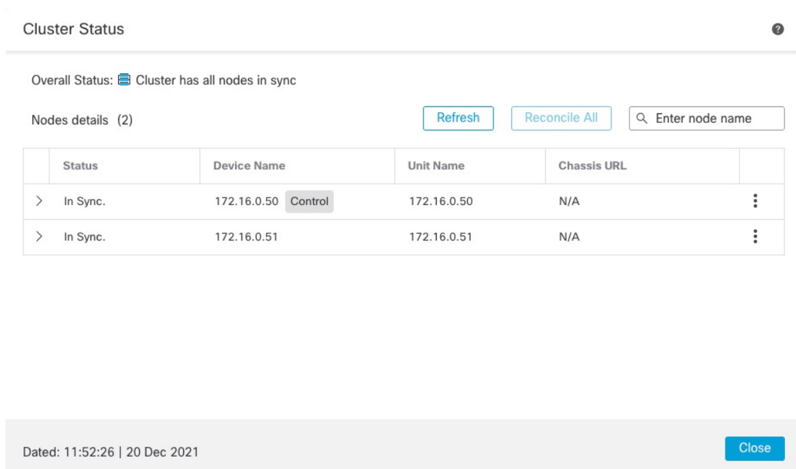
图 21: 集群状态
