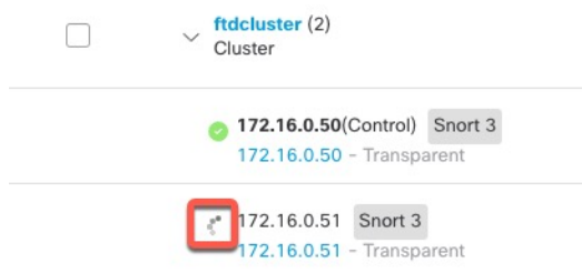
图 15: 节点注册
