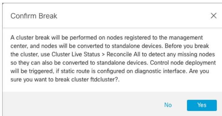
图 19: 确认中断
