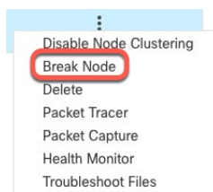
图 16: 中断节点
