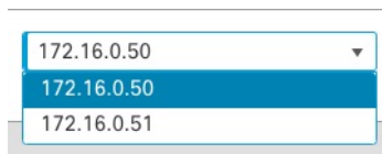
图 8: 选择节点
