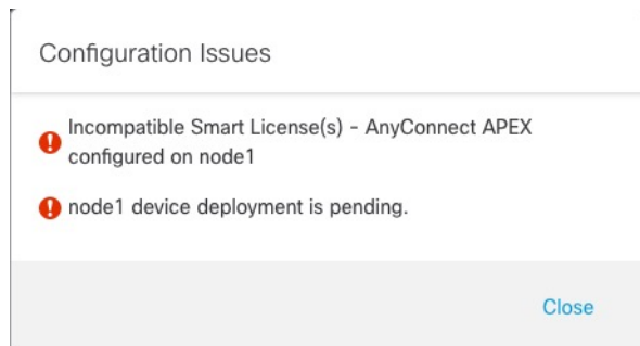
图 2: 配置问题
