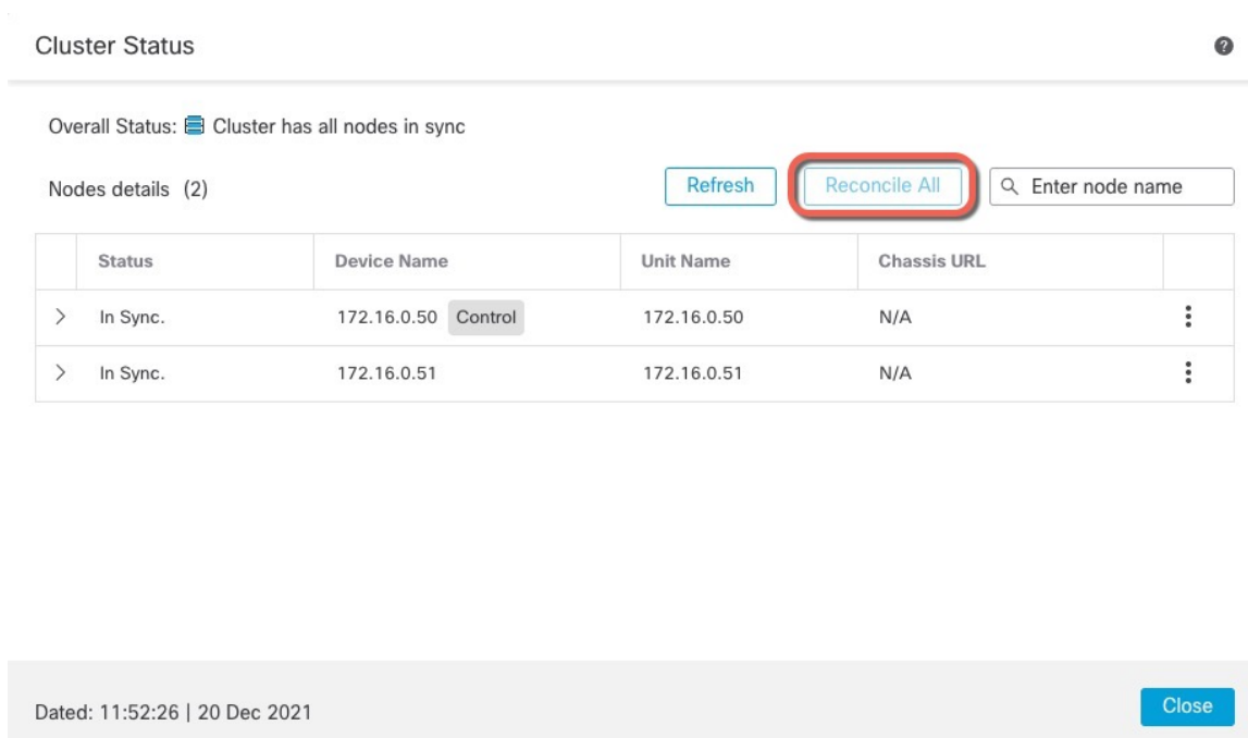
图 25: 协调全部
