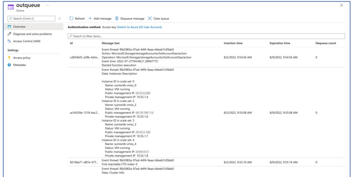
图 13: 出站队列
