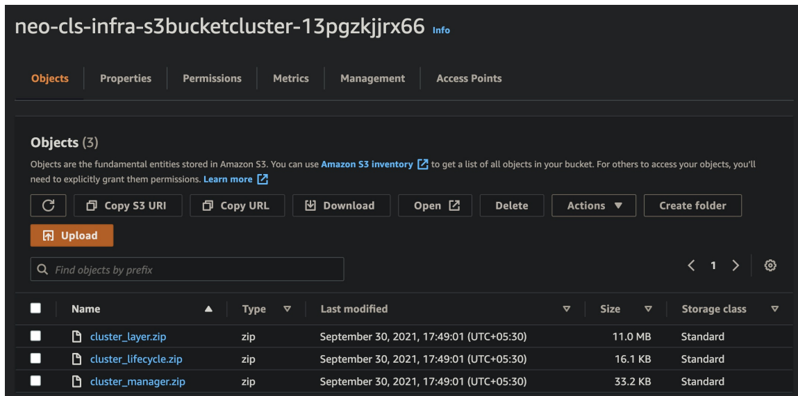
图 3. S3 桶
