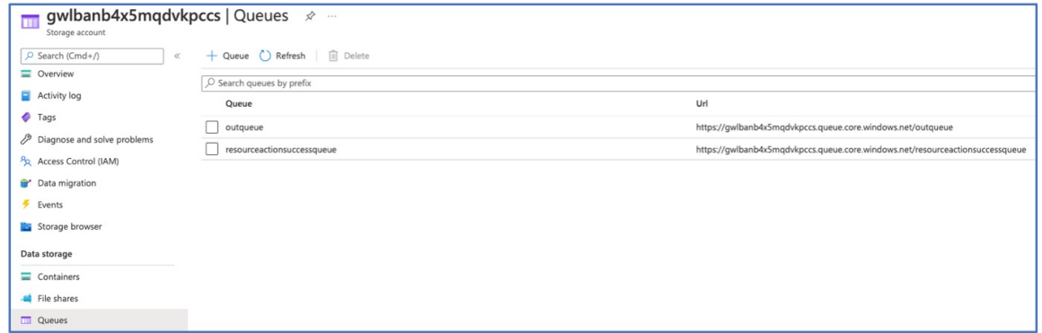
图 13: 出站队列
