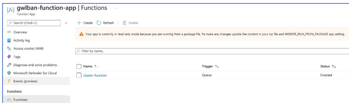
图 11: 功能
