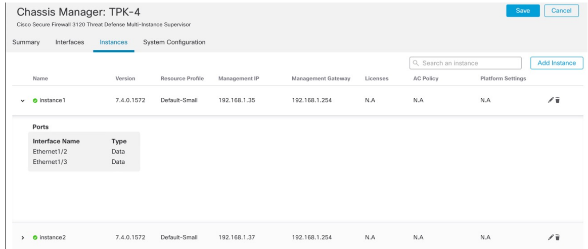
图 59: 实例 (Instances)
