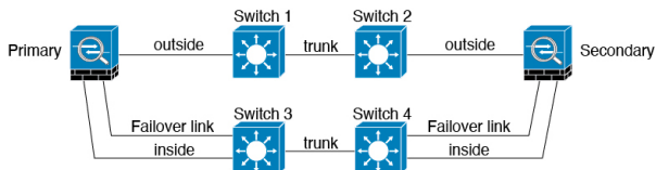
图 5: 使用安全交换机连接
