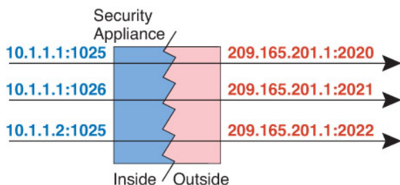
图 7: 动态 PAT
