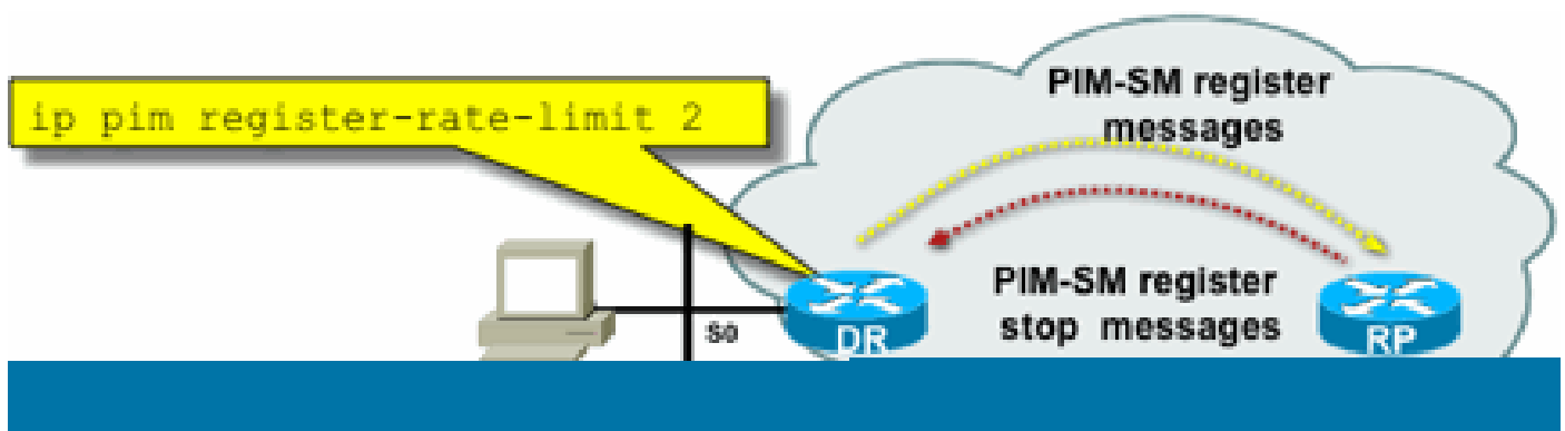
圖8: PIM-SM暫存器隧道控制
