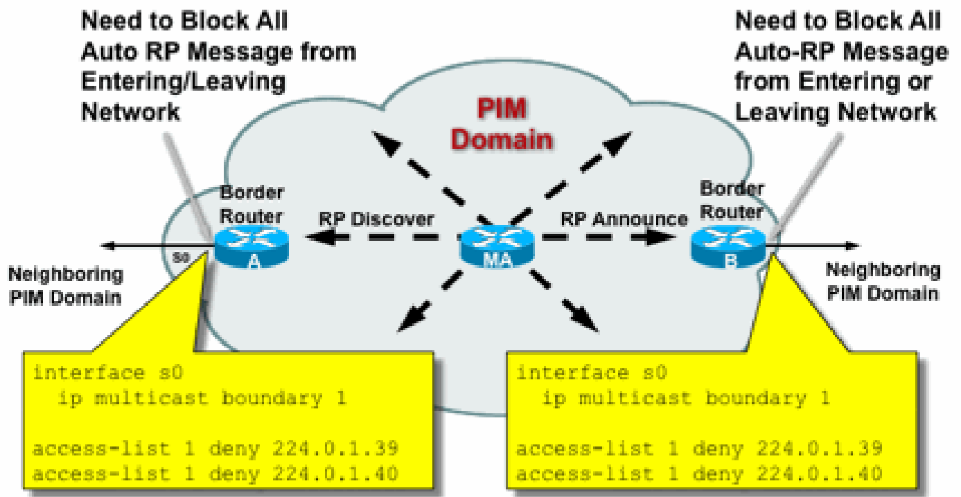
圖10：組播邊界命令
