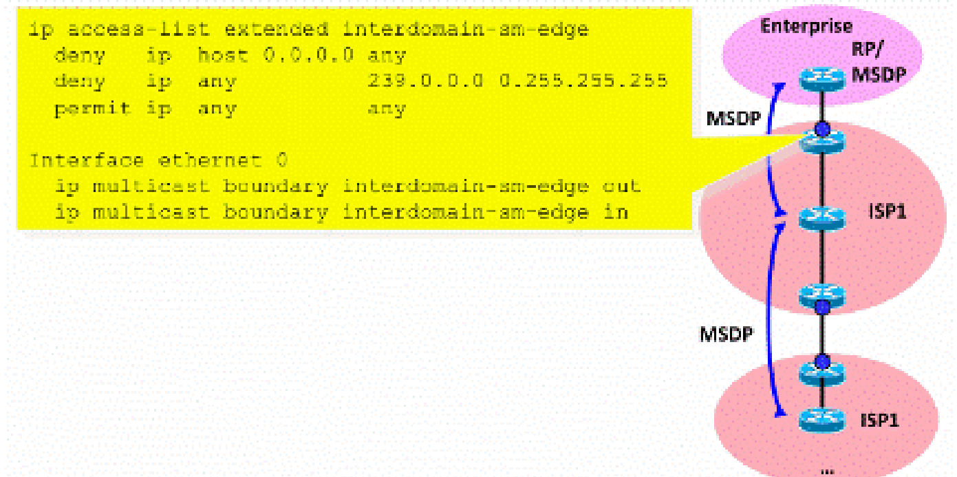
圖13：域間(*,G)過濾器
