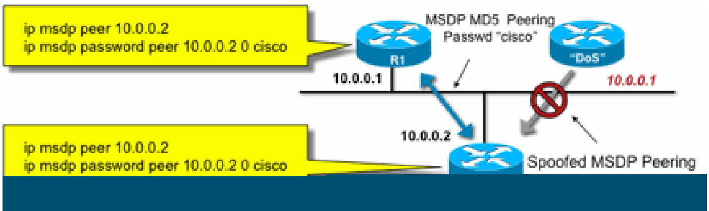
圖15: MSDP MD5鄰居身份驗證
