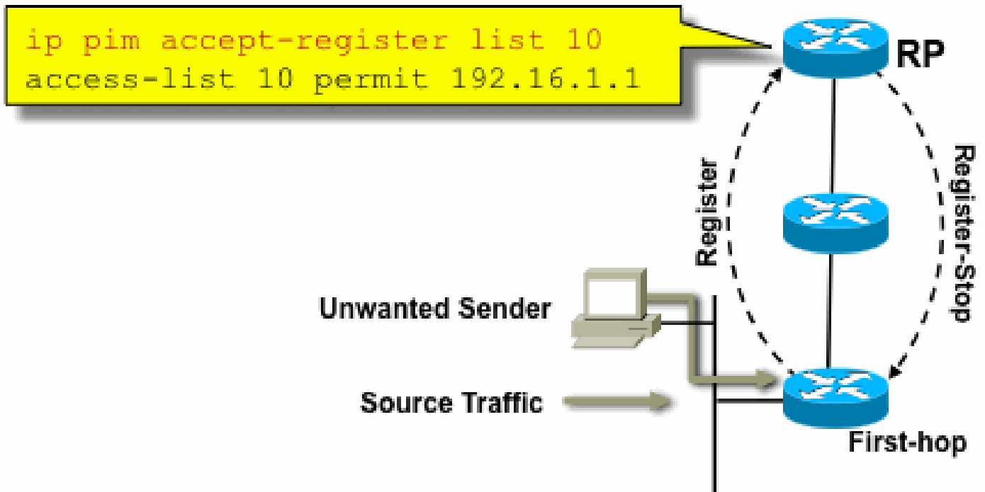
圖17:PIM-SM源控制
