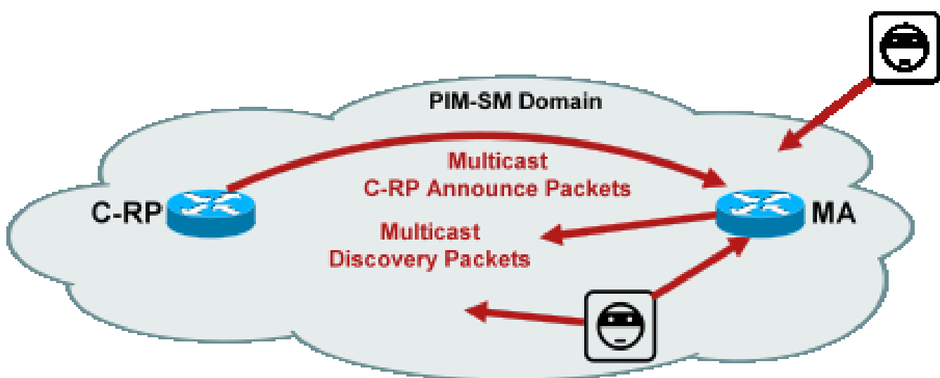
圖2：自動RP資料包
