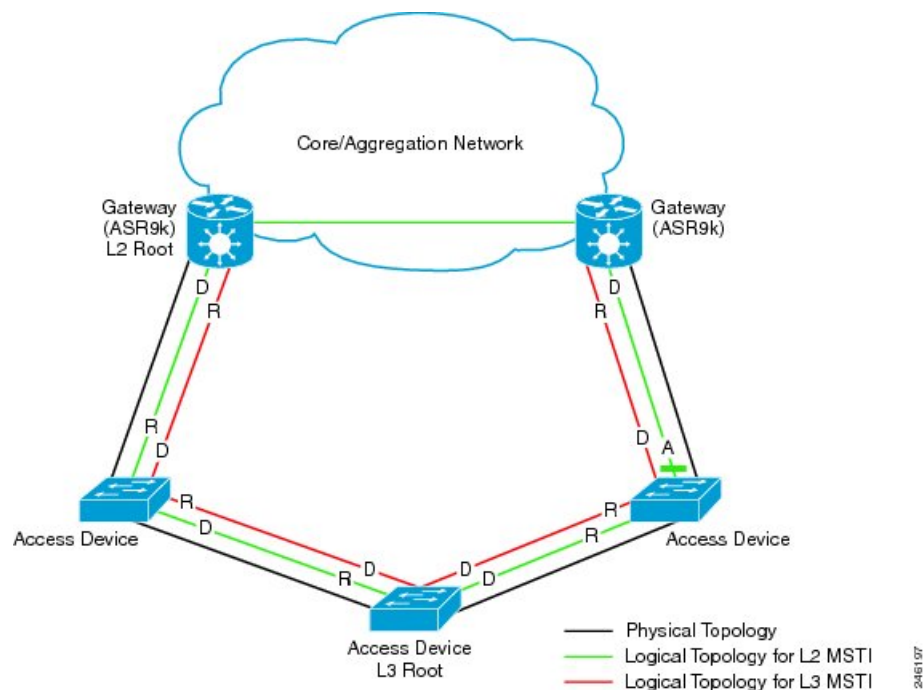
Figure 62: MSTAG Edge Mode scenario
