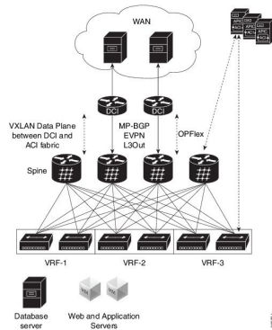
Figure 34: OpFlex Topology
