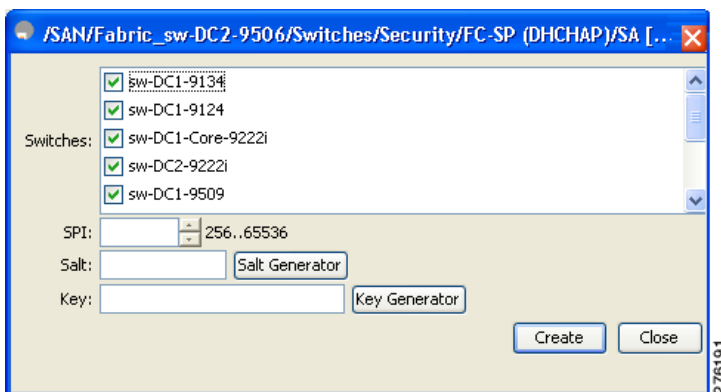
Figure 15-3 Create SA Parameters
