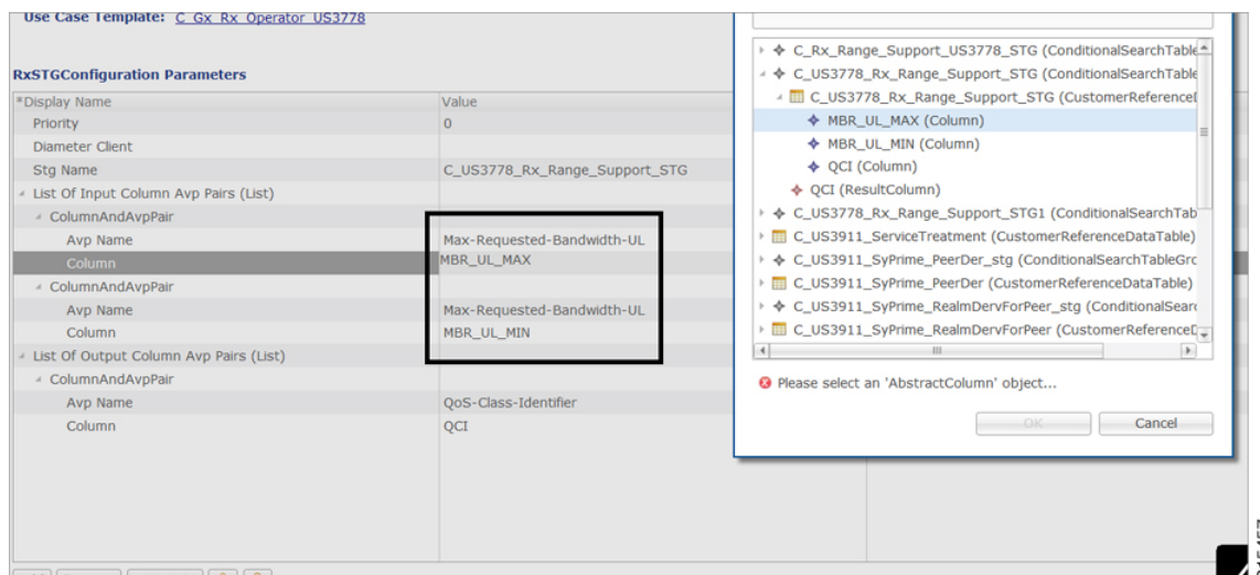
Figure 156: RxSTGconfiguration Column Parameter
