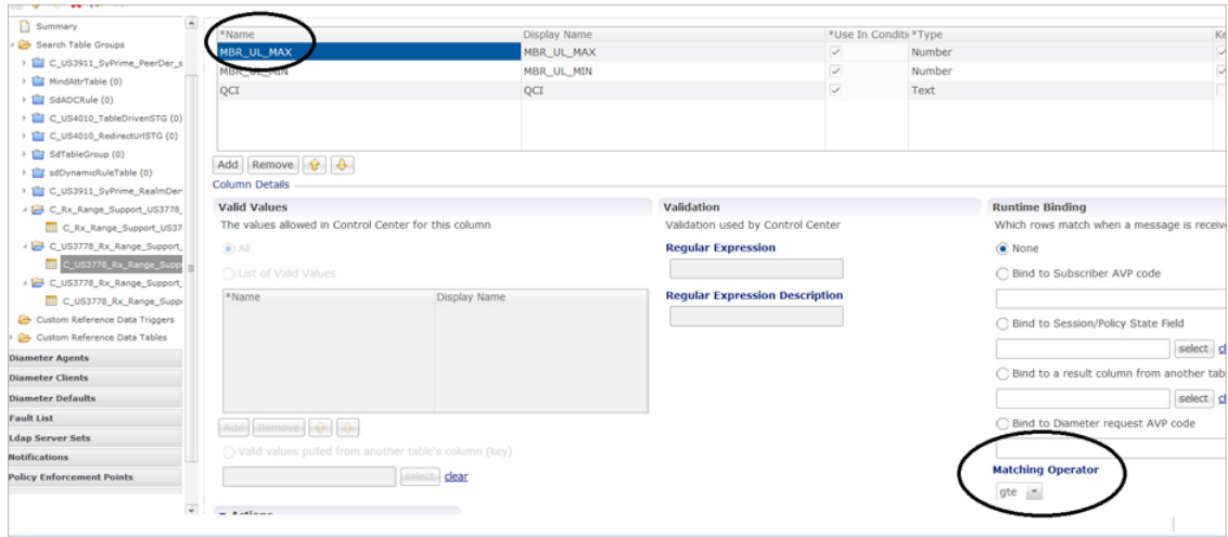
Figure 154: MBR_UL_MAX Input Column
