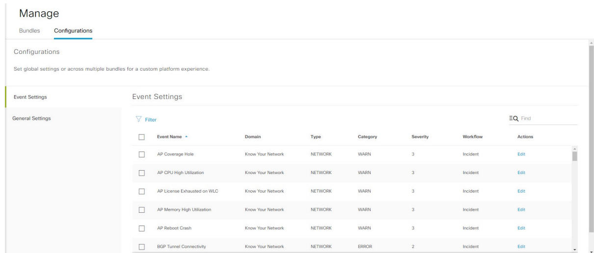
図 18 : [Event Settings] ウィンドウ
