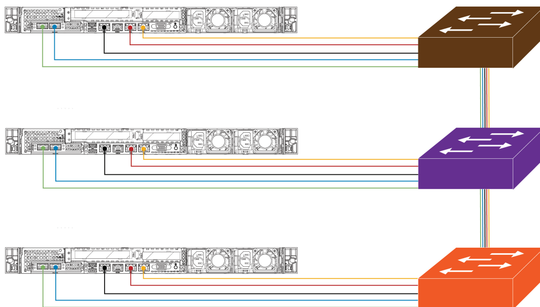
図 2: 3 ノードクラスタの推奨される配線
