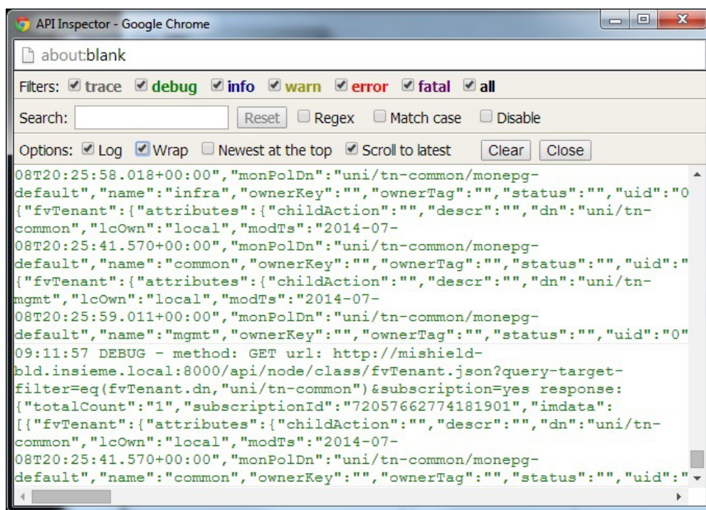
図 113: API インスペクタ
