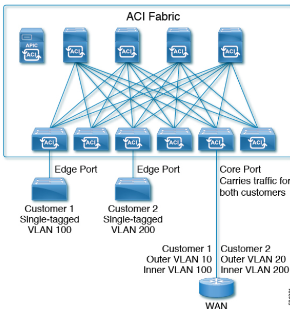
図 33: ACI 802.1 q トンネル
