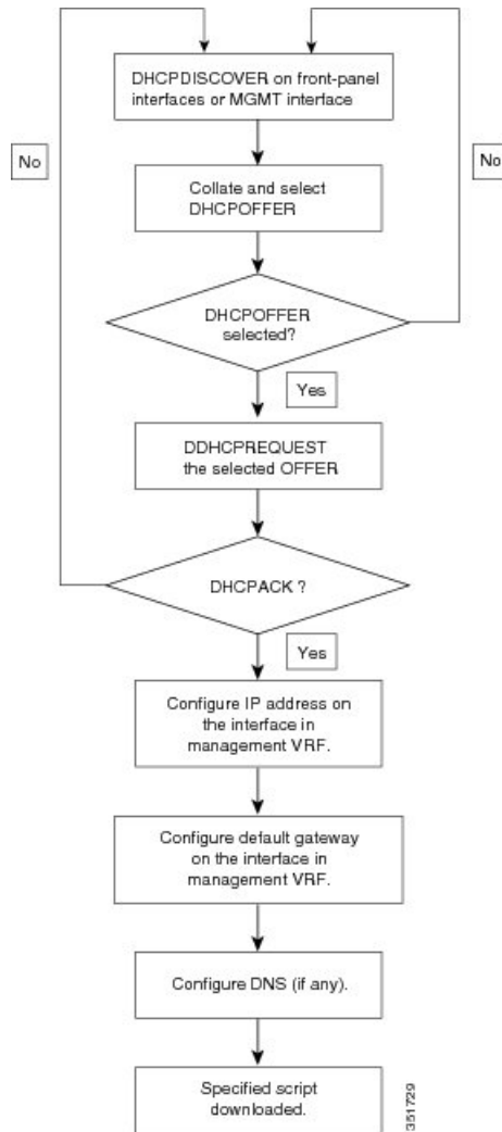
図 3: DHCP 検出プロセス
