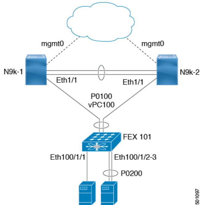
図 3: デュアルホーム FEX トポロジ
