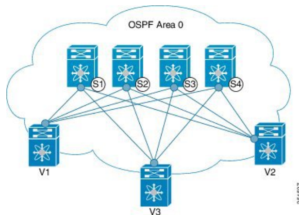
図 46: アンダーレイ ルーティング プロトコルとしての OSPF
