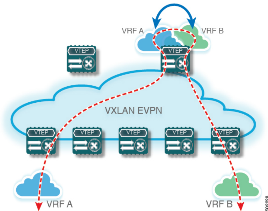
図 11: 中央集中型 VRF ルートリーク：カスタム VRF による共有インターネット
