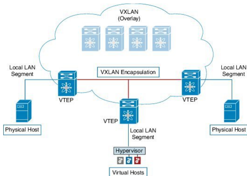
図 44: オーバーレイの概要
