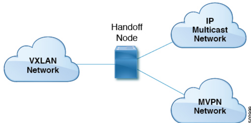
図 42: VXLAN : MVPN ハンドオフ ネットワーク
