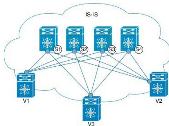
図 47: アンダーレイ ルーティング プロトコルとしての IS-IS
