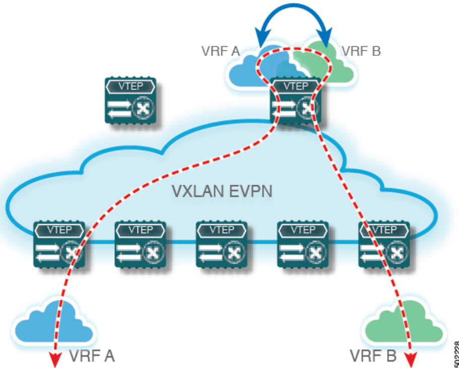
図 10: 中央集中型 VRF ルート リーク : カスタム VRF による特定のプレフィックス
