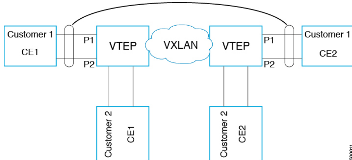
図 22: VXLAN P2P トンネルを通じた LACP トンネリング
