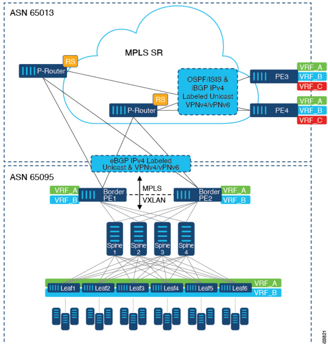
図 37: DCからコアネットワークドメインへの分離を使用したトポロジ
