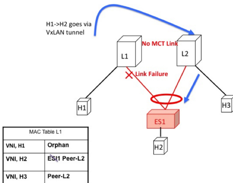
図 60: L1 での ES1 障害。H1->H2 が VxLAN トンネル経由でブリッジされます。
