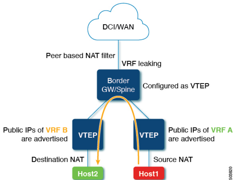
図 13: EVPN分散NAT設定トポロジ
