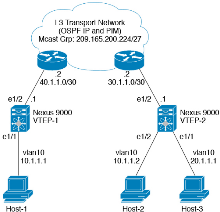
図 30: VXLAN デキャップスイッチでの出力の SVI でのルーテッド ACL
