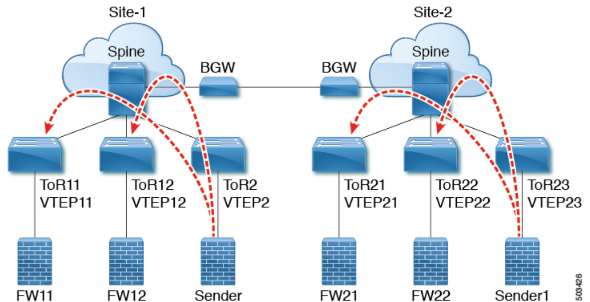
図 76: マルチサイトトポロジの VNF
