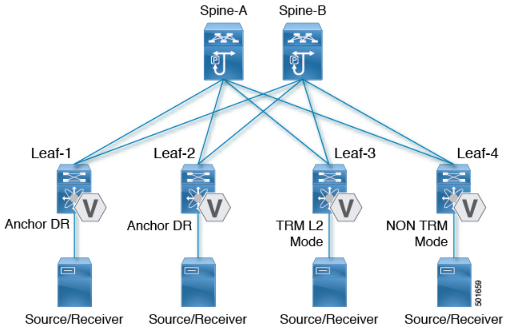
図 21: TRM レイヤ 2/レイヤ 3 混合モード
