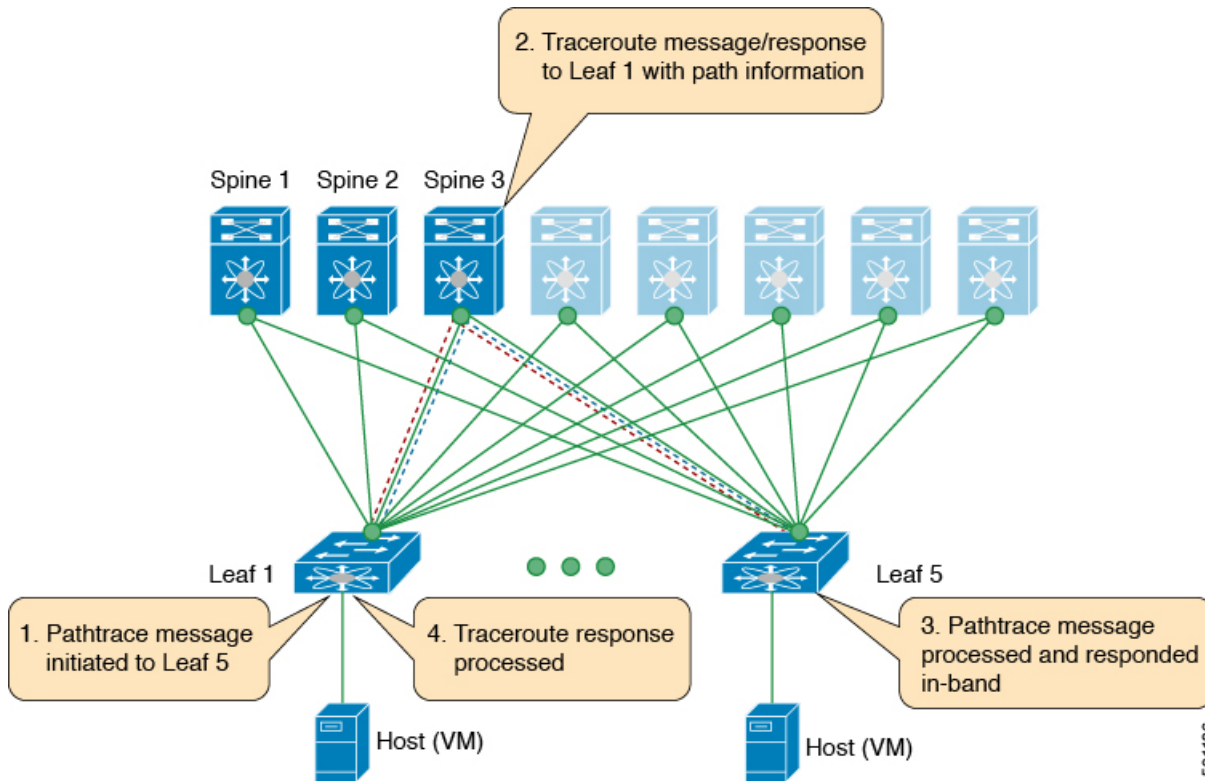
図 15: Traceroute メッセージ
