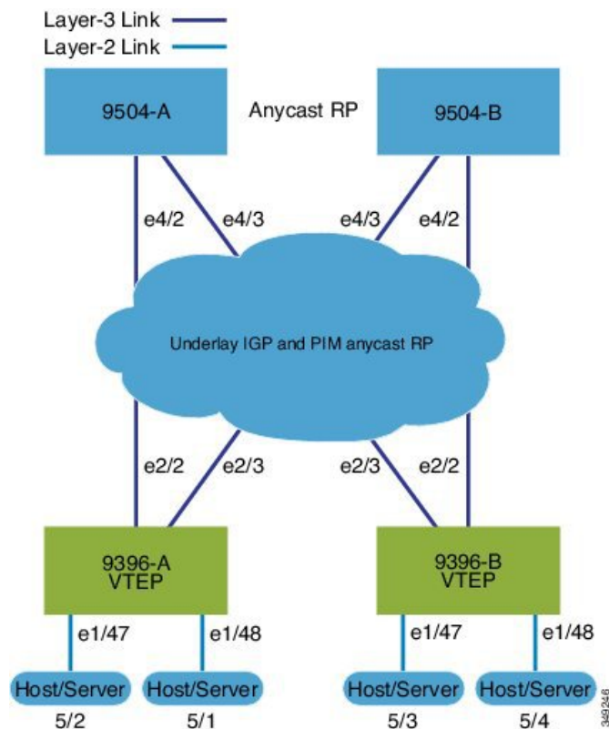
図 7: VXLAN BGP EVPN のトポロジ (IBGP)
