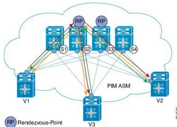
図 49: IP マルチキャストルーティング プロトコルとしての PIM ASM
