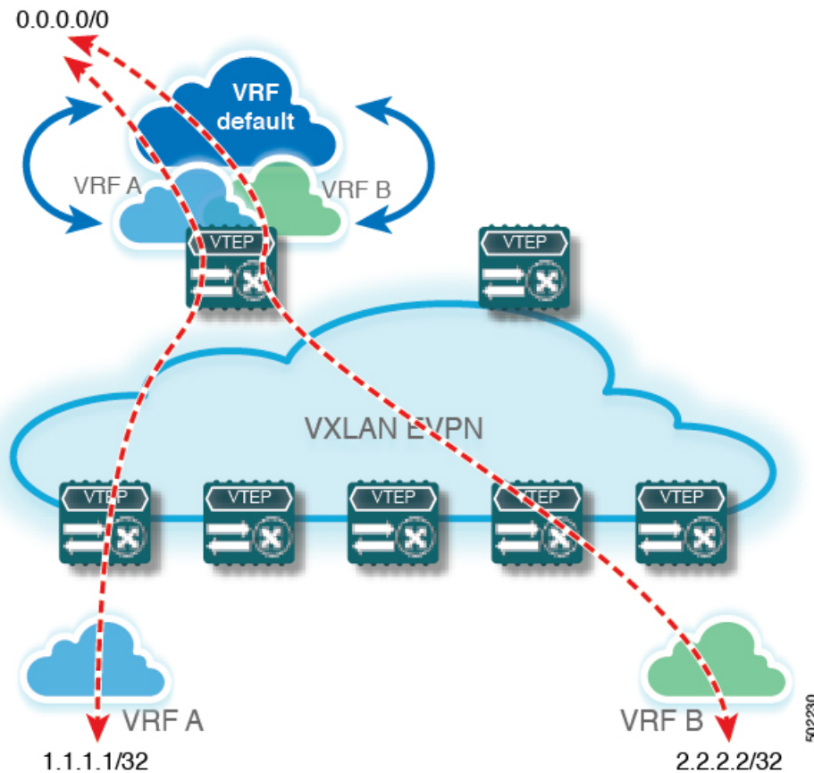
図 12: 中央集中型 VRF ルート リーク : VRF デフォルトでの共有インターネット
