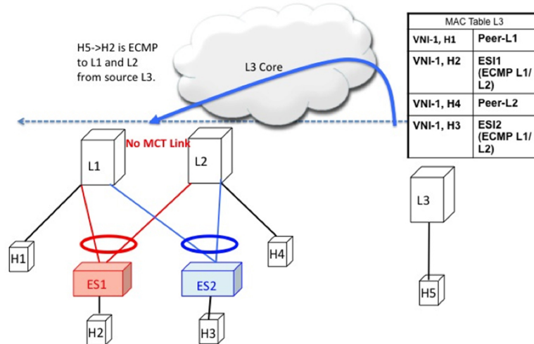
図 65: レイヤ 2 VXLAN ゲートウェイ。L3は MAC ECMP を L1/L2 に実行します。
