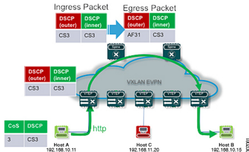
図 34: VXLAN トンネル内部のマーキング
