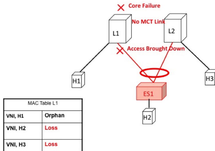
図 61: L1 のコア障害。MCTがないため、H1->H2はすべての接続を失います。
