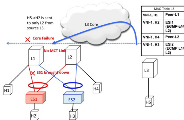
図 67: レイヤ 2 VXLAN ゲートウェイ。L1 でコア障害が発生しました。L3 は MAC ECMP リストから L1 を削除します。これは、L1 へのルート到達可能性が L3 でなくなるために発生します。
