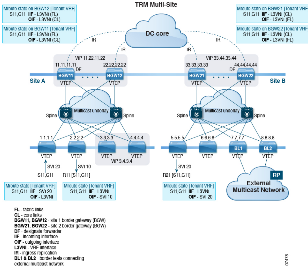
図 18: マルチサイトトポロジの TRM、BL 外部マルチキャスト接続
