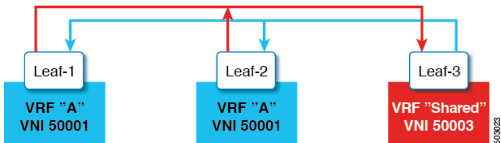
図 5: 共有サービス VRF
