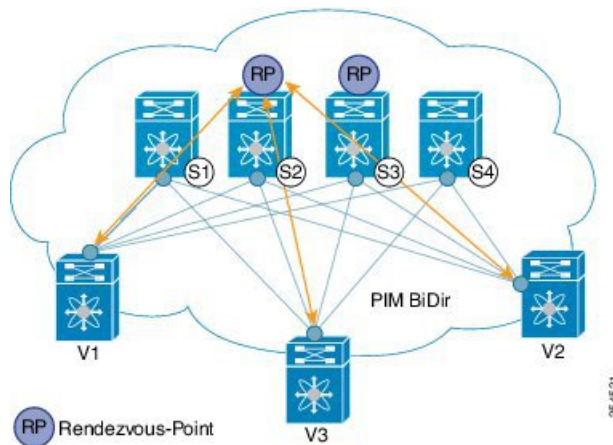
図 50: IP マルチキャスト ルーティング プロトコルとしての PIM BiDir
