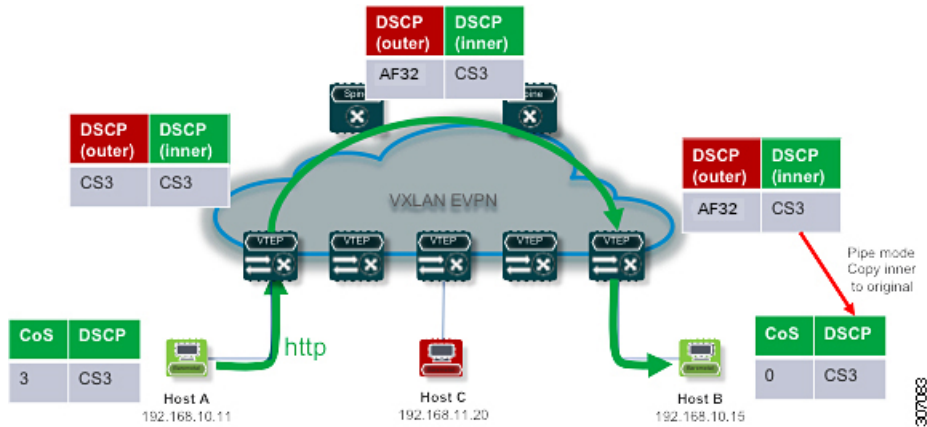
図 36: パイプモードの内部 DSCP 値がレイヤ 3 パケットのカプセル化解除されたパケット DSCP 値にコピーされる
