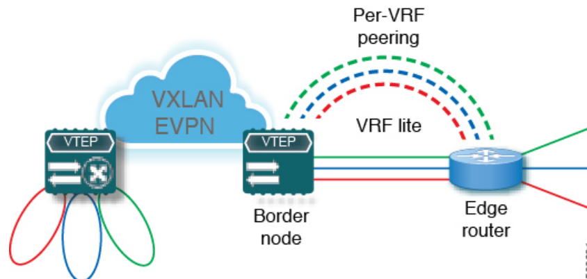
図 9: VRF-Lite を使用したレイヤ 3 外部接続
