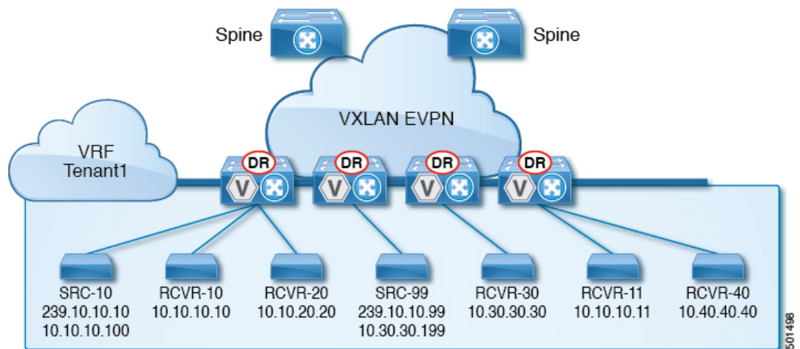
図 20: VXLAN EVPN TRM
