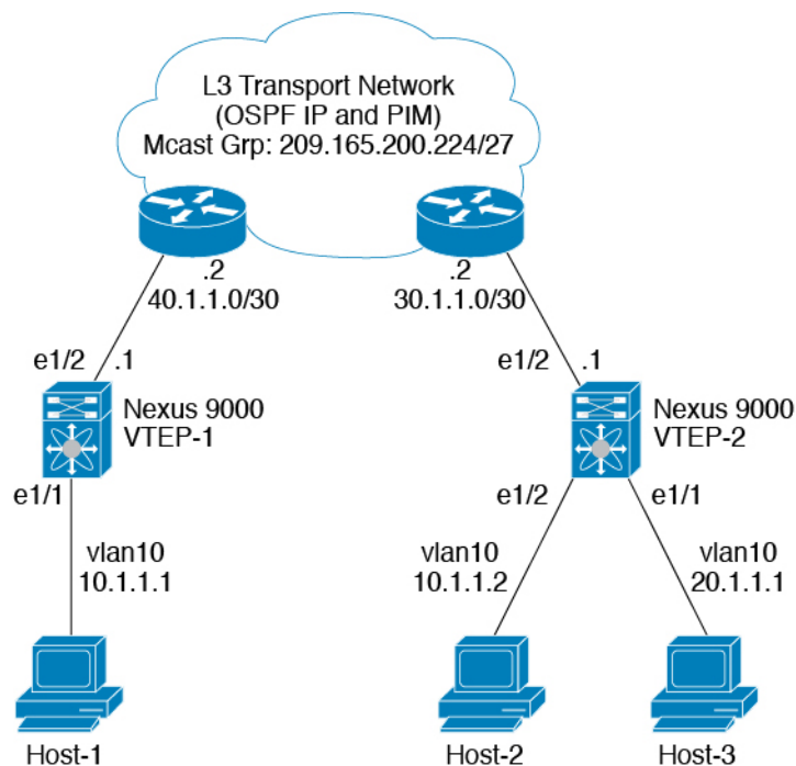
図 27: VXLAN Encap スイッチでの入力の SVI でのルーテッド ACL
