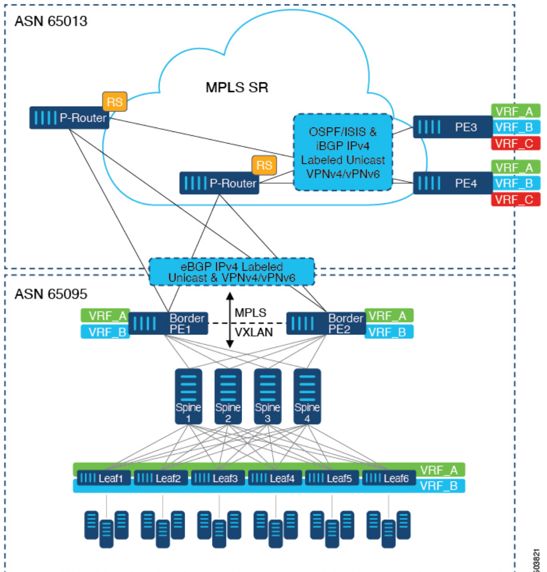
図 39: DCからコアネットワークドメインへの分離を使用したトポロジ
