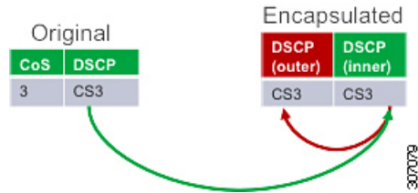
図 32: レイヤ 3 パケットから VXLAN 外部ヘッダーへの優先順位のコピー
