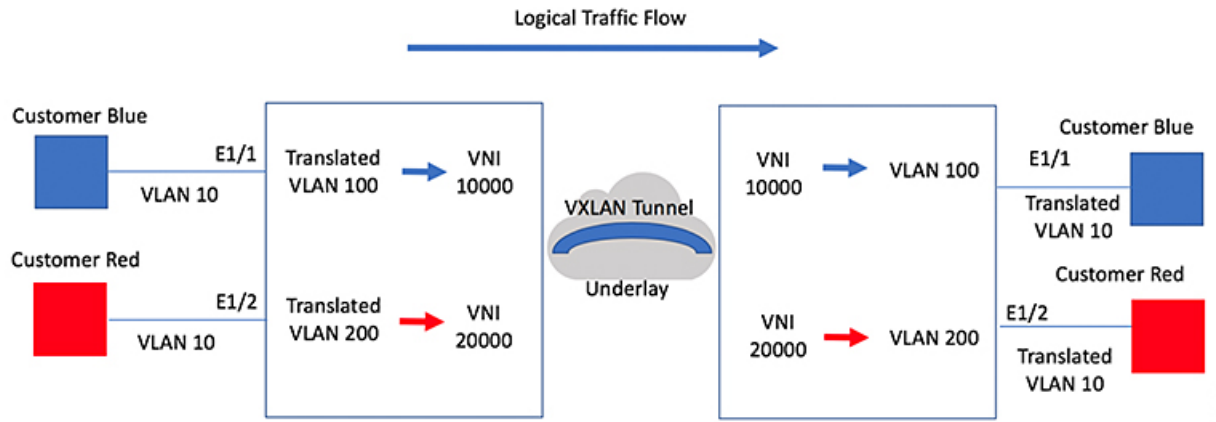
図 23:論理的トラフィック フロー
