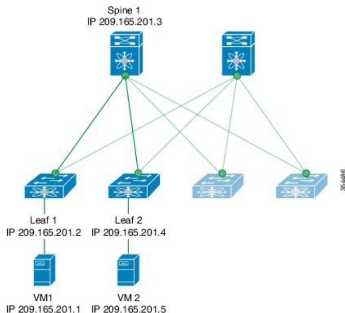
図 17: VXLAN ネットワーク
