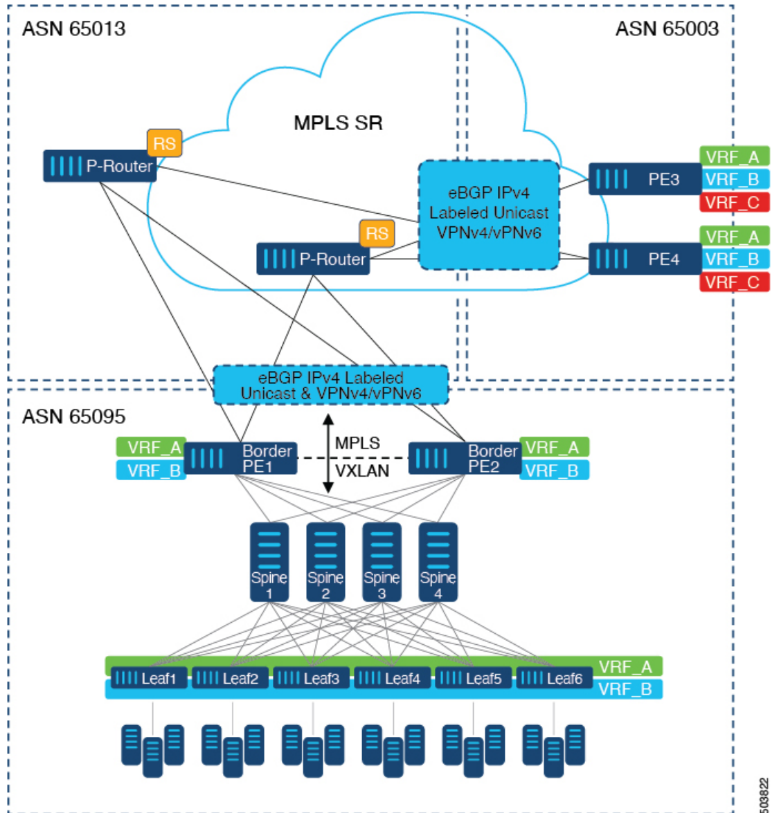
図 40: コアネットワーク内の複数の管理ドメイン
