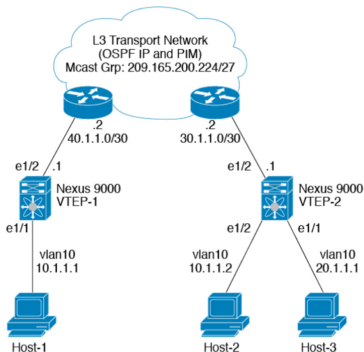
図 26: VXLAN Encap スイッチの VLAN ACL
