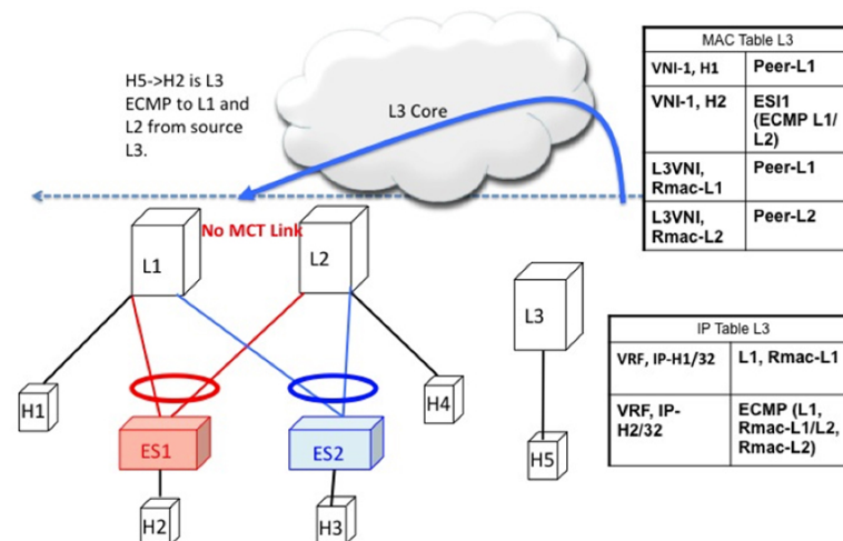
図 68: レイヤ 3 VXLAN ゲートウェイ。L3 は、サブネット間トラフィックの L1/L2 に対して IP ECMP を実行します。
