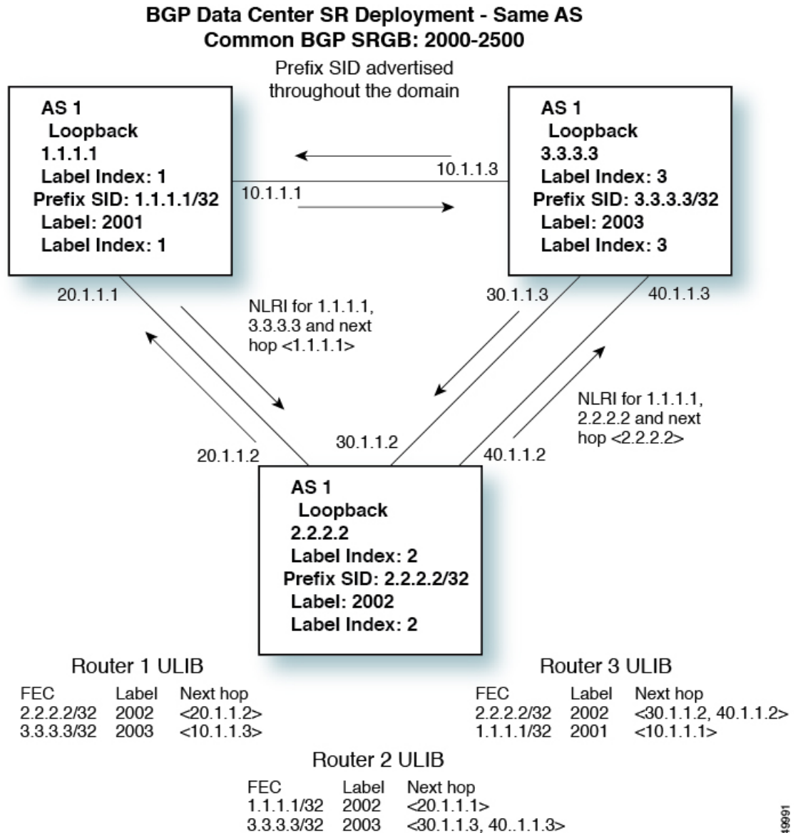
図 12: BGP プレフィックス SID の簡単な例
