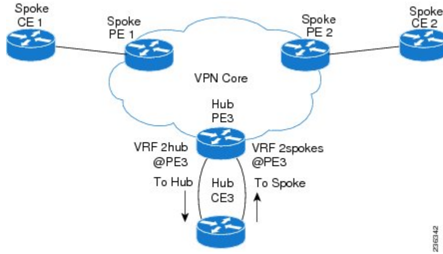
図 3: ハブアンドスポーク トポロジ
