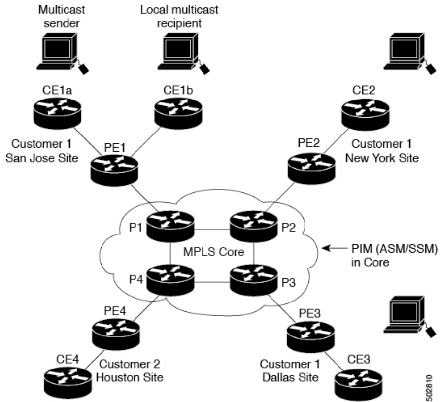
図 15: デフォルト マルチキャスト配信ツリーの概要
