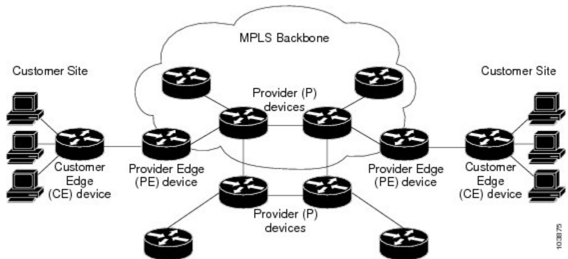
図 2: MPLS レイヤ 3 VPN の基本用語
