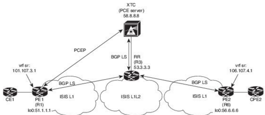
図 9: 参照トポロジ
