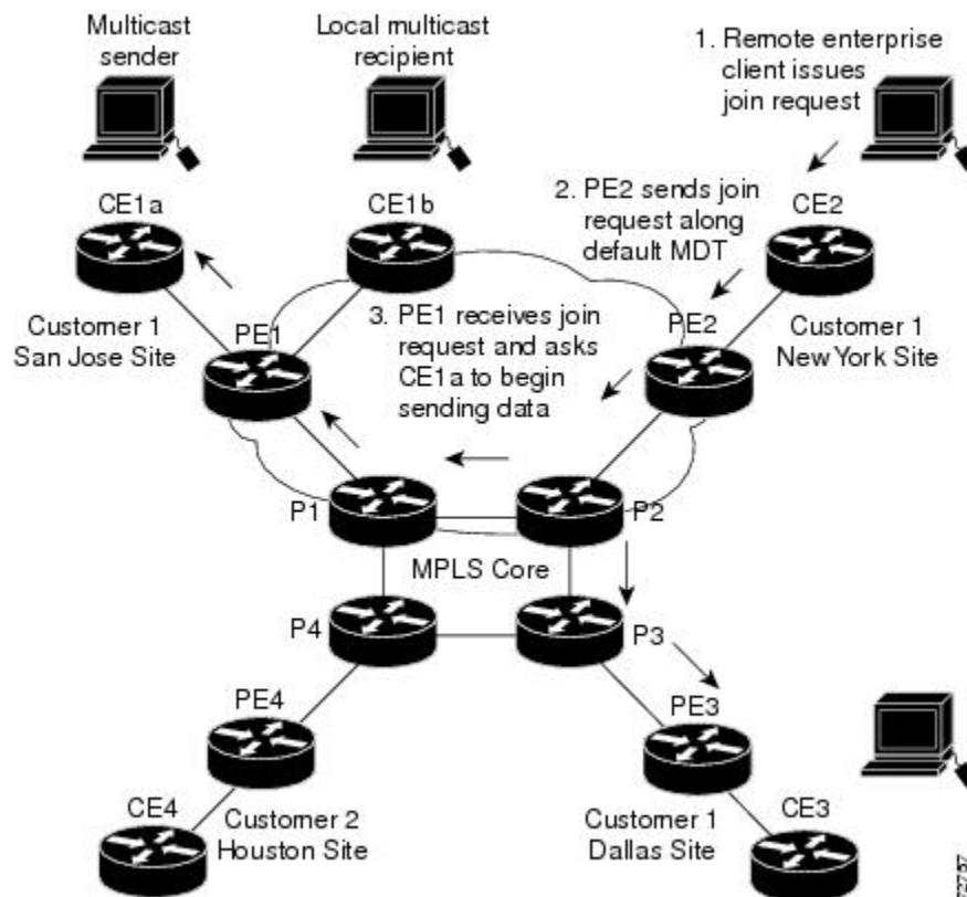
図 16: データ MDT の初期化
