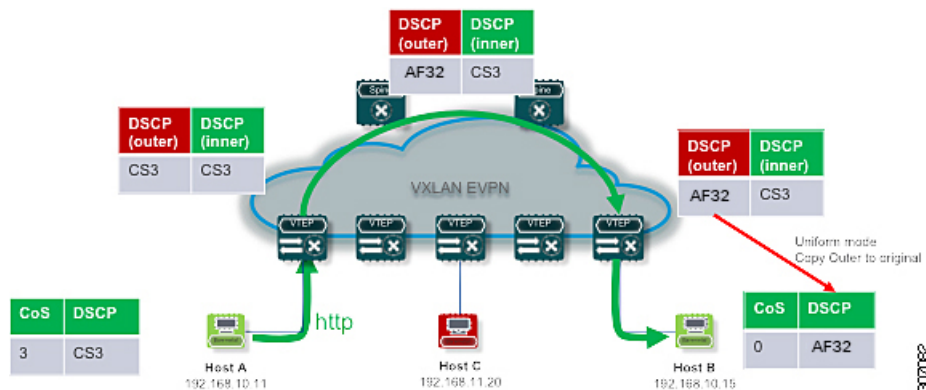
図 44: ユニフォームモードの外部 DSCP 値がレイヤ 3 パケットのカプセル化解除されたパケット DSCP 値にコピーされる
