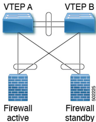
図 56: 静的ルーティングを使用するデュアル接続ファイアウォール
