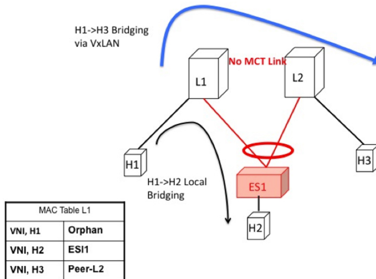
図 61: L1でのローカルブリッジング。VXLAN経由のH1からH3へのブリッジング。vPCでは、H1からH3へはMCTリンク経由です。
