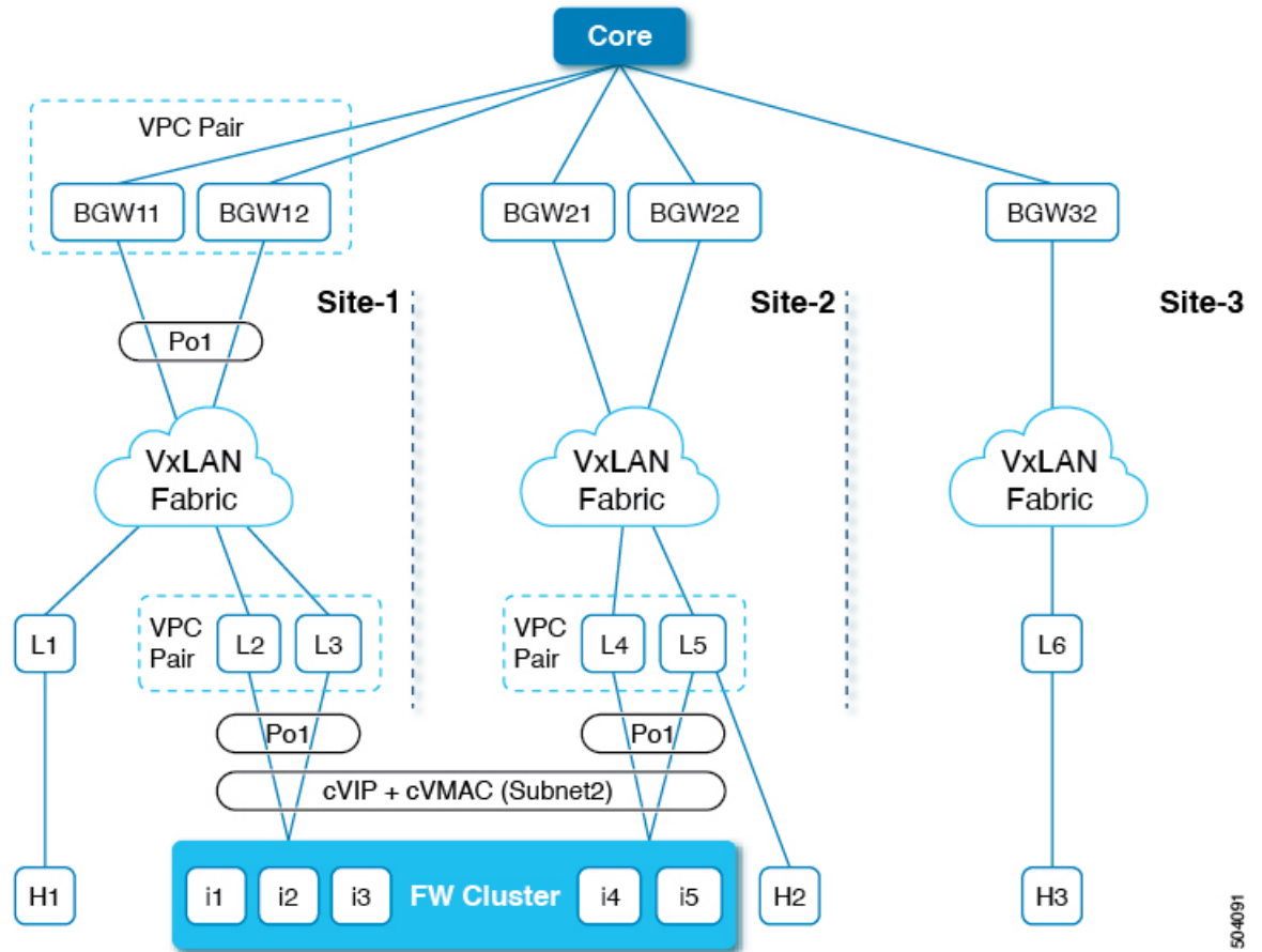
図 16: VXLAN EVPN によるファイアウォール クラスタリング
