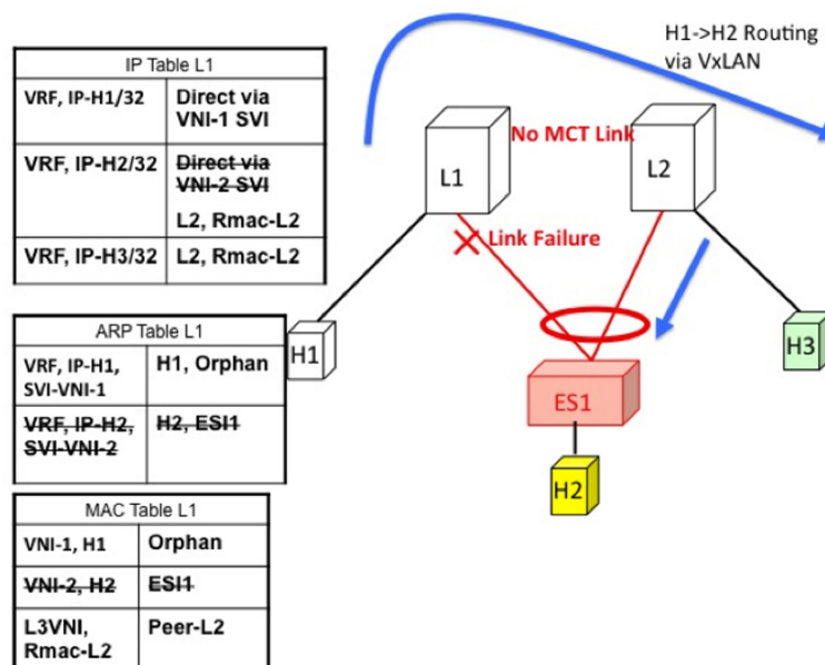
図 65: H1、H2、および H3 は異なる VLAN にあります。L1 で ESI が失敗します。H1 から H2 へのルーティングは、VXLAN トンネルカプセル化によって行われます。
