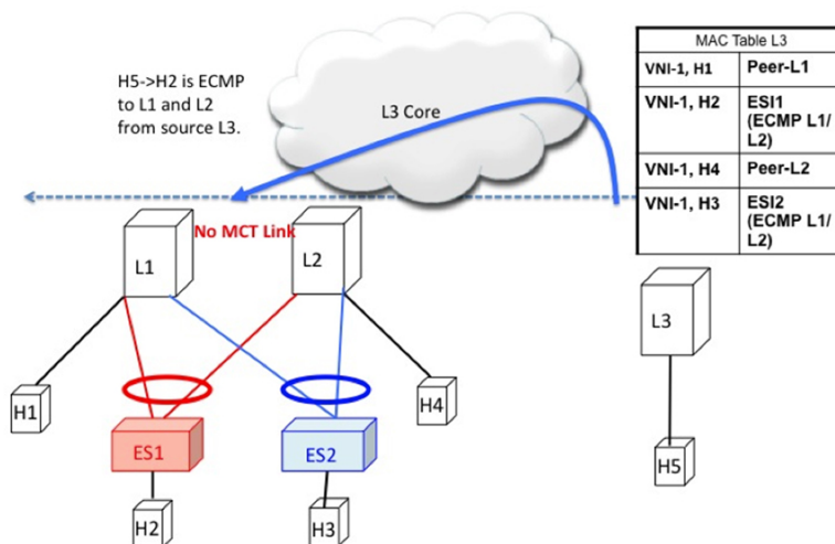
図 67: レイヤ 2 VXLAN ゲートウェイ。L3 は MAC ECMP を L1/L2 に実行します。
