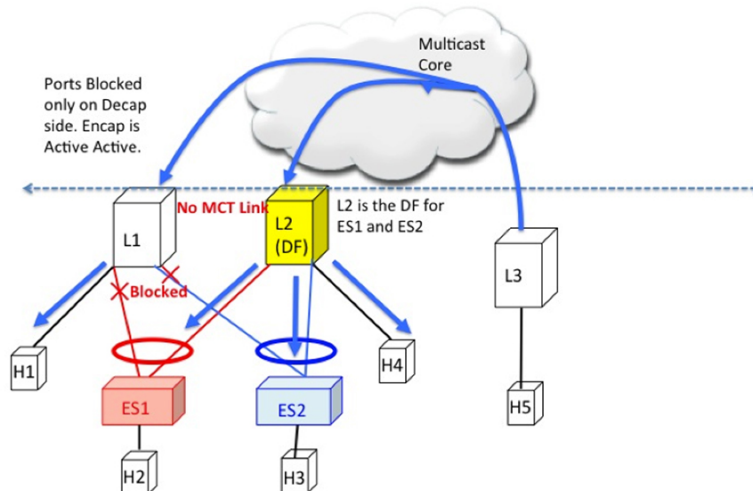
図 73: L3 で発信される BUM トラフィック。L2 は ES1 および ES2 の DF です。L2 はカプセル化を解除し、ES1、ES2、およびオーファンに転送します。L1 はカプセル化を解除し、オーファンにのみ転送します。
