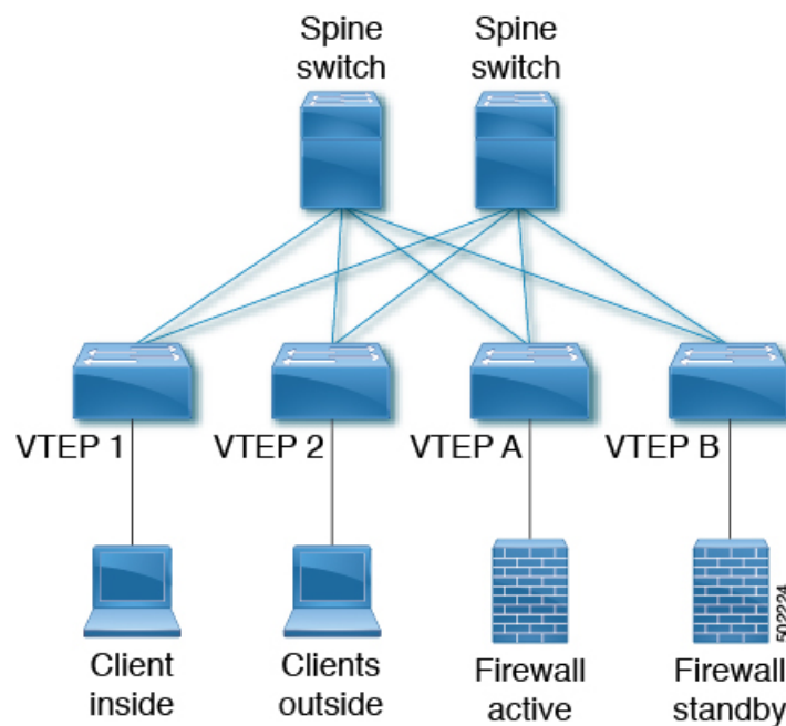
図 55: ファイアウォール接続を使用したトポロジの概要
