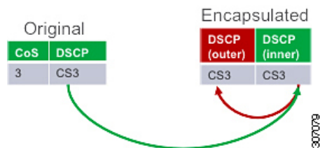
図 41: レイヤ 3 パケットから VXLAN 外部ヘッダーへの優先順位のコピー
