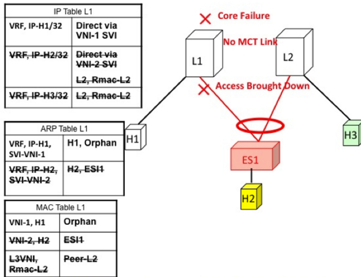
図 66: H1、H2、および H3 は異なる VLAN にあります。コアが L1 で失敗します。アクセスがダウンします。H1 はすべての接続を失います。
