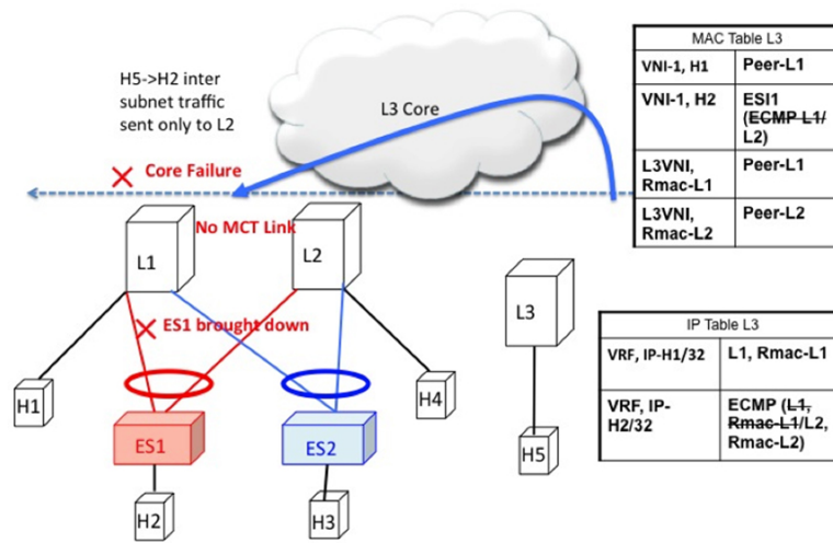
図 72: レイヤ 3 VXLAN ゲートウェイ。コア障害。L1 へのすべての L3 ECMP パスは、ルートの到達可能性がなくなるため、L3 で取り消されます。
