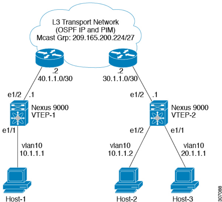
図 36: VXLAN Decap スイッチのレイヤ 2 VNI の VLAN ACL
