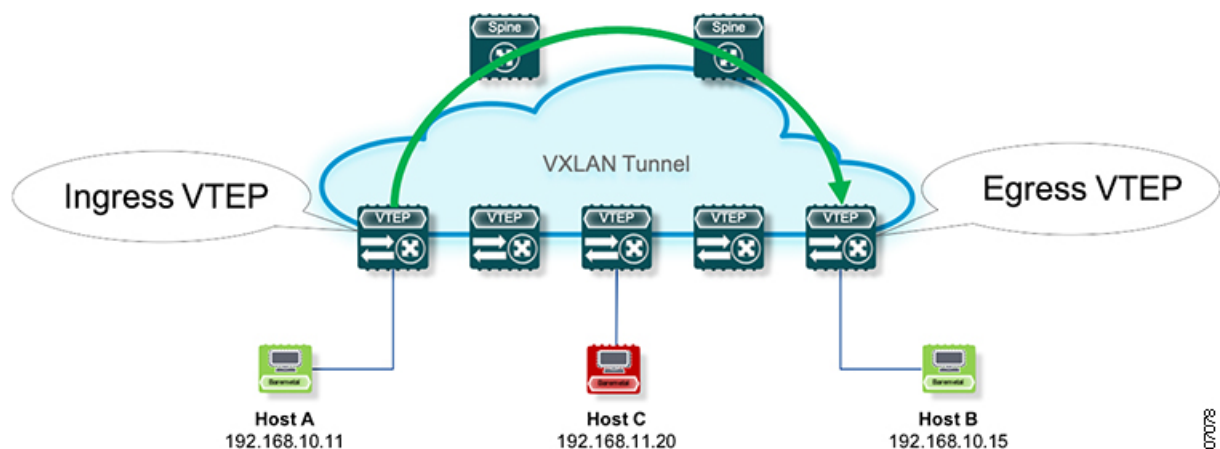
図 40: VXLAN ネットワーク
