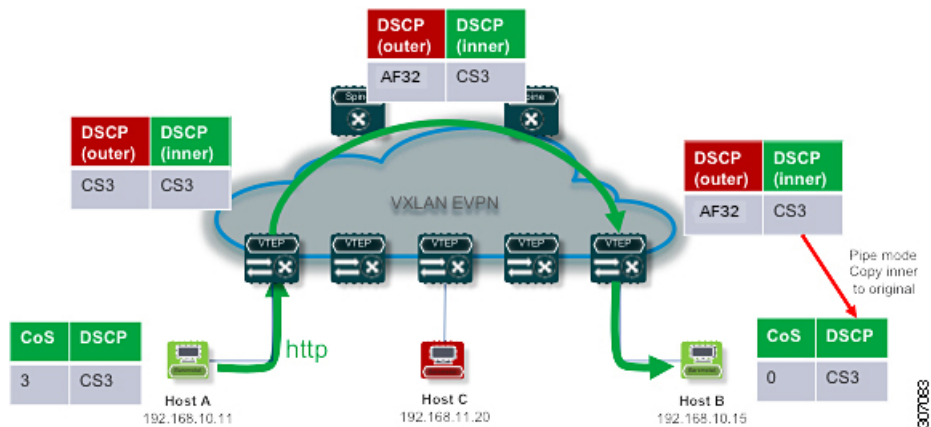
図 45: パイプモードの内部 DSCP 値がレイヤ 3 パケットのカプセル化解除されたパケット DSCP 値にコピーされる
