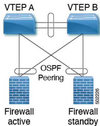
図 59: OSPFを使用したデュアル接続ファイアウォール
