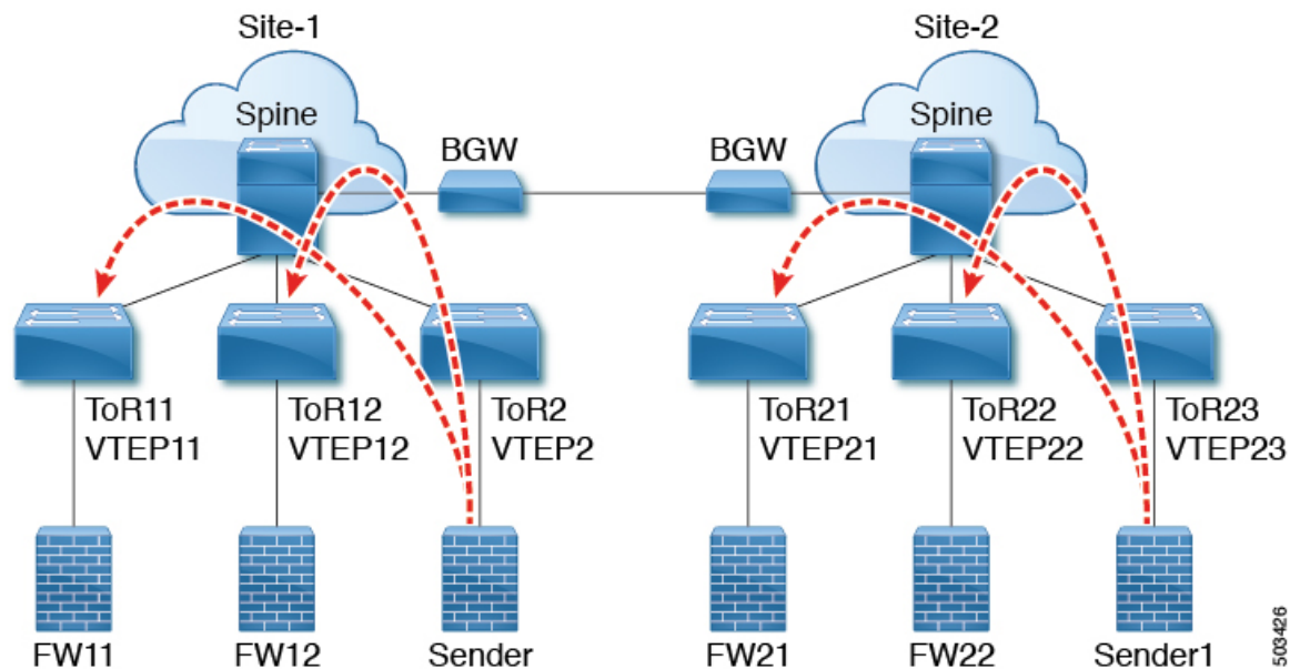
図 78: マルチサイトトポロジの VNF
