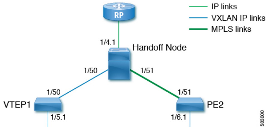
図 52: EVPN (TRM) と MVPN のシームレスな統合のサンプルトポロジ
