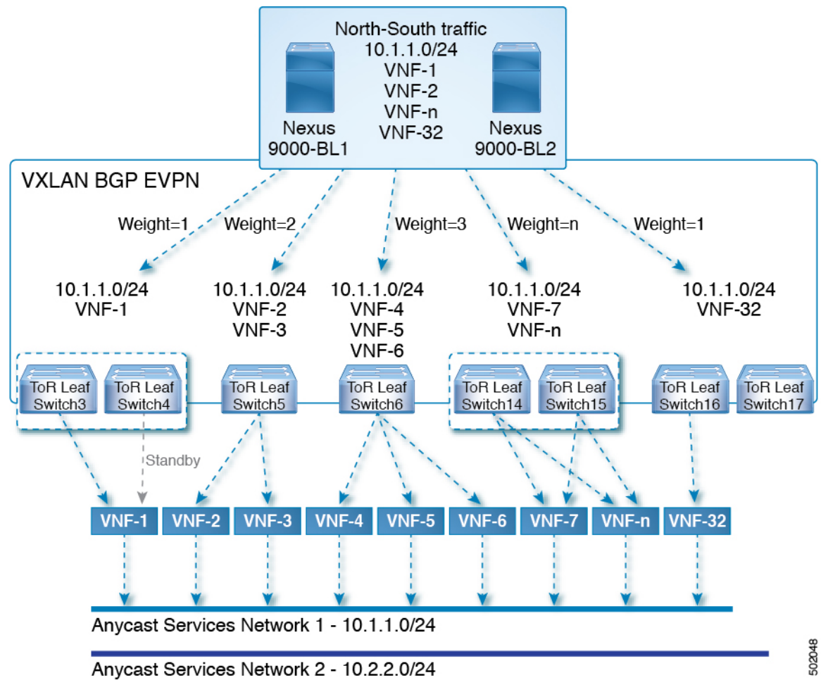
図 76: サンプル トポロジ (North-South トラフィック)
