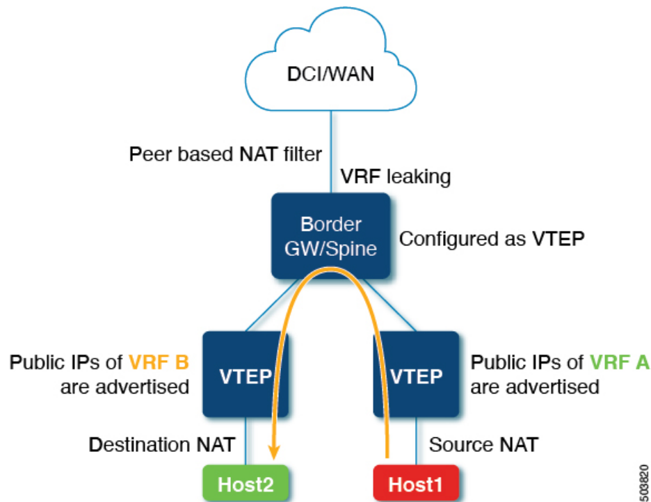
図 21: EVPN分散NAT設定トポロジ
