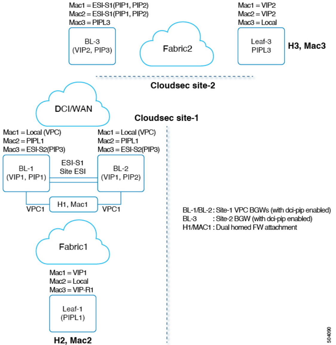
図 39: Cloudsec の MLAG BGW サポート
