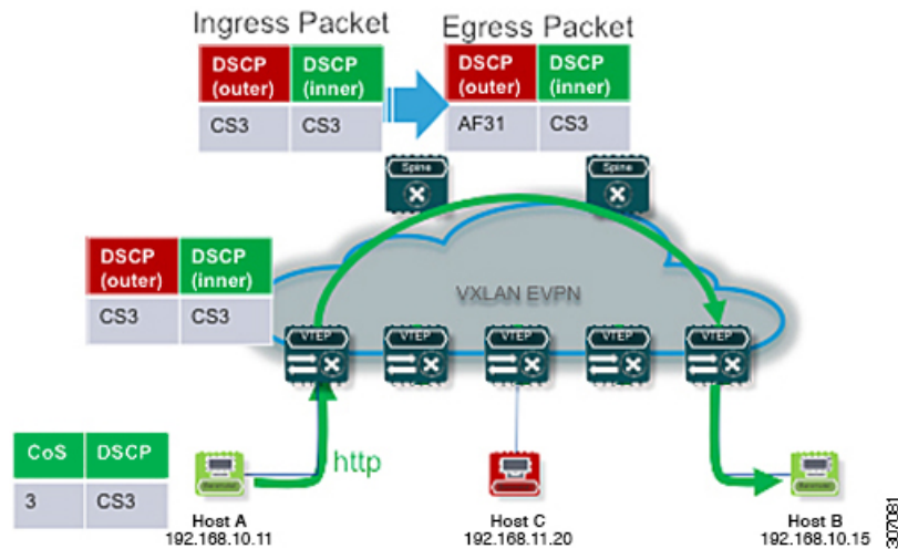
図 43: VXLAN トンネル内部のマーキング
