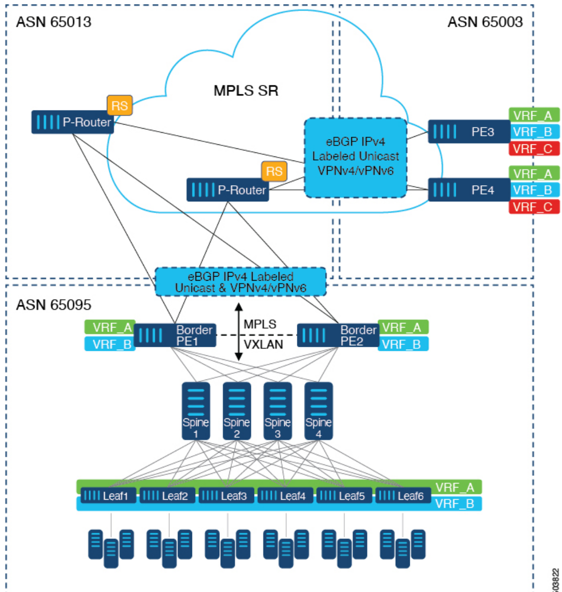
図 49: コアネットワーク内の複数の管理ドメイン
