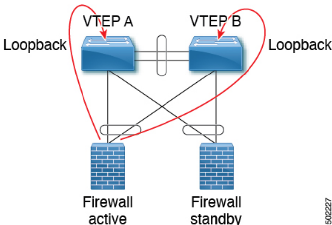
図 58: eBGP を使用したデュアル接続ファイアウォール
