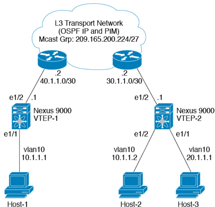
図 34: VXLAN Encap スイッチの VLAN ACL
