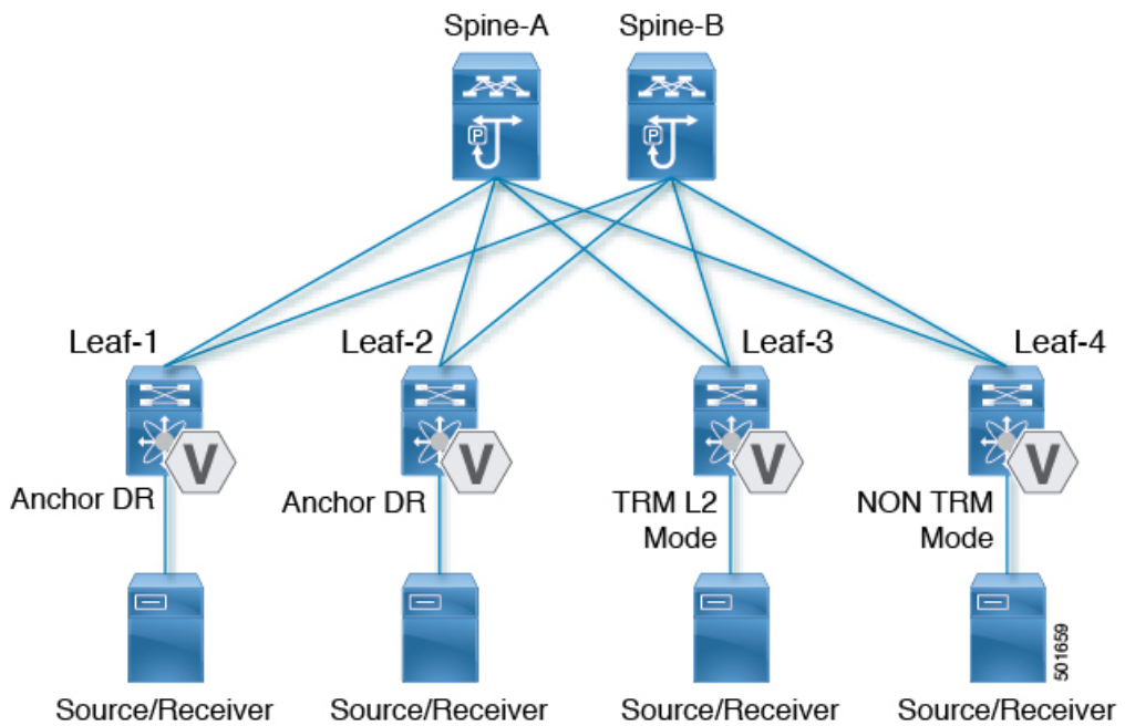
図 29: TRM レイヤ 2/レイヤ 3 混合モード
