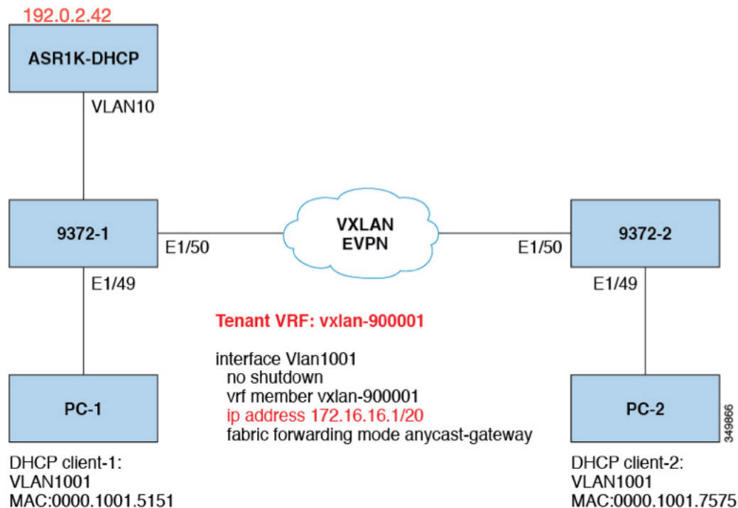
図 54: トポロジの例
