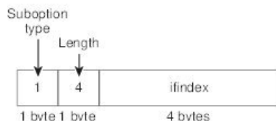
Figure 4: サブオプションの packets 形式
