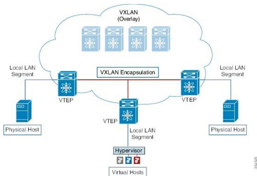
図4: オーバーレイの概要
