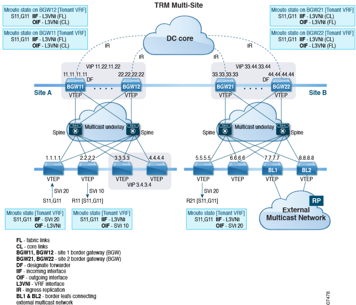
図 26: マルチサイトトポロジの TRM、BL 外部マルチキャスト接続
