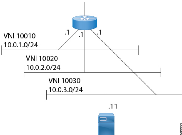
図 58: レイヤ 2 VXLAN ファブリックを使用したデフォルトゲートウェイとしてのファイアウォール
