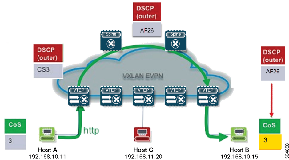
図 42: カプセル化解除されたパケットで復元された非 IP CoS 値
