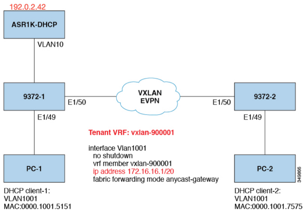
図 51: トポロジの例
