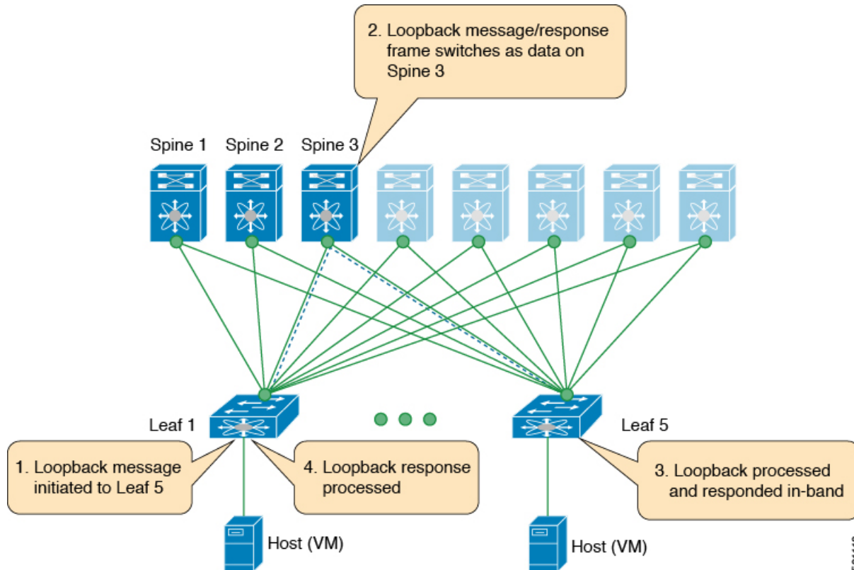
図 21: loopback メッセージ
