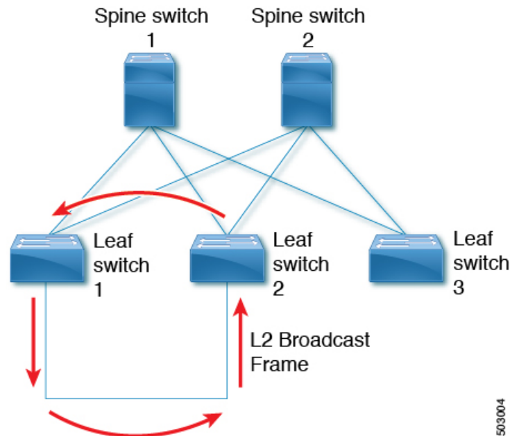
図 23: 直接接続された 2 つのリーフ ノード
