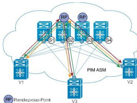
図 9: IP マルチキャストルーティング プロトコルとしての PIM ASM
