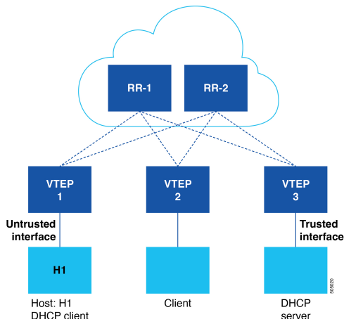
図 52: VXLAN での DHCP スヌーピング
