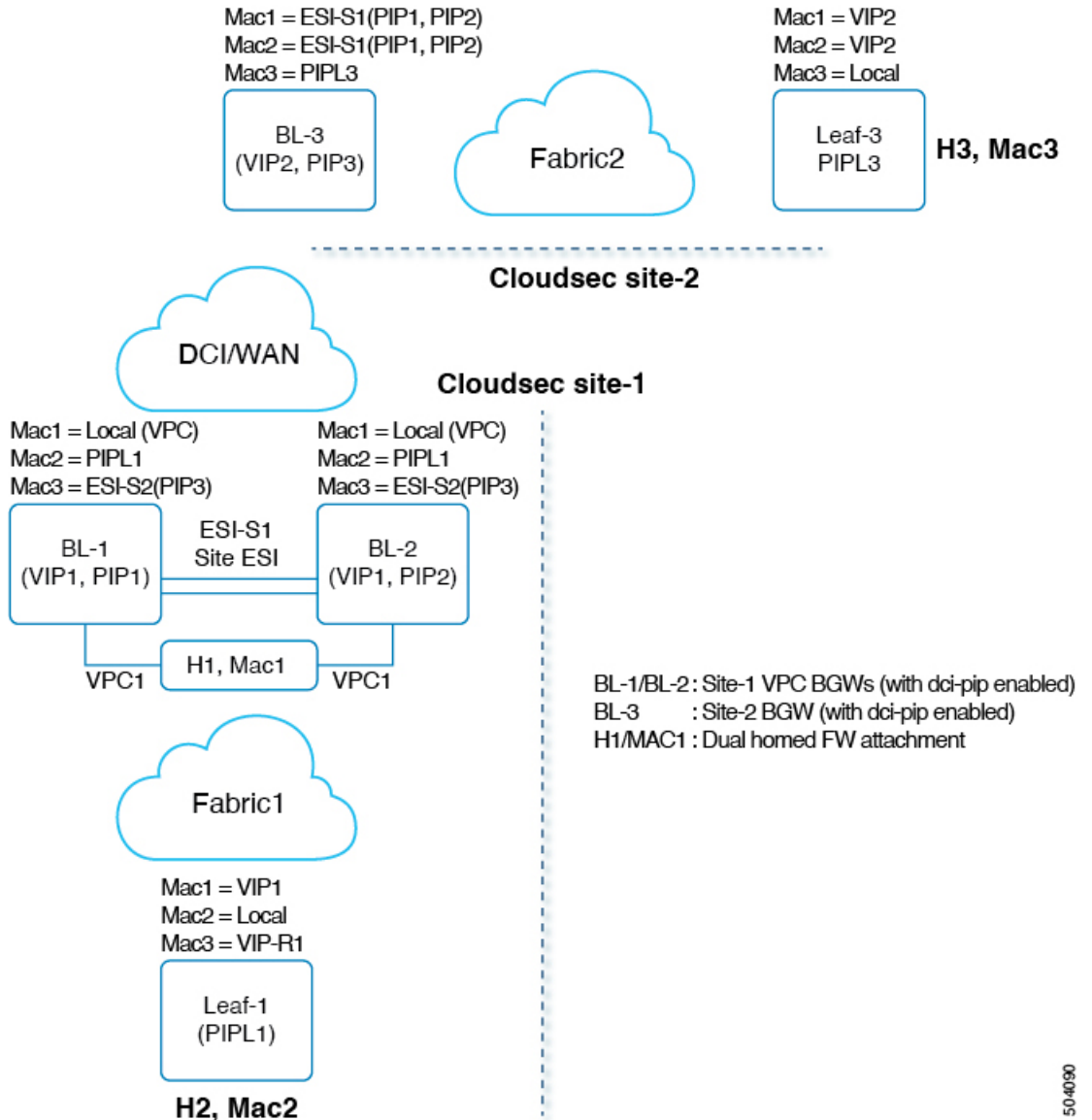
図 34 : Cloudsec の vPC BGW サポート
