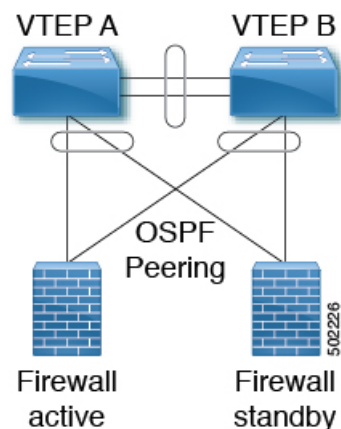
図 57: OSPF を使用したデュアル接続ファイアウォール
