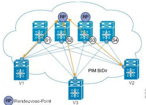
図 10: IP マルチキャストルーティング プロトコルとしての PIM BiDir
