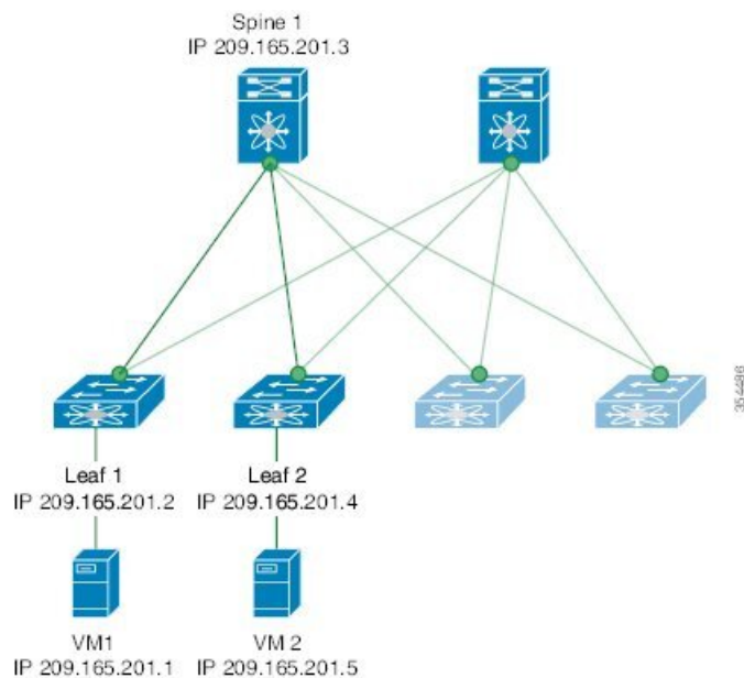
図 24: VXLAN ネットワーク
