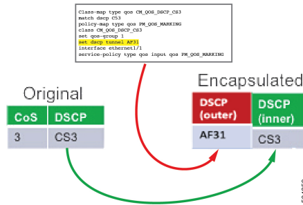
図 38: セット構成から適用された VXLAN 外部 DSCP 値
