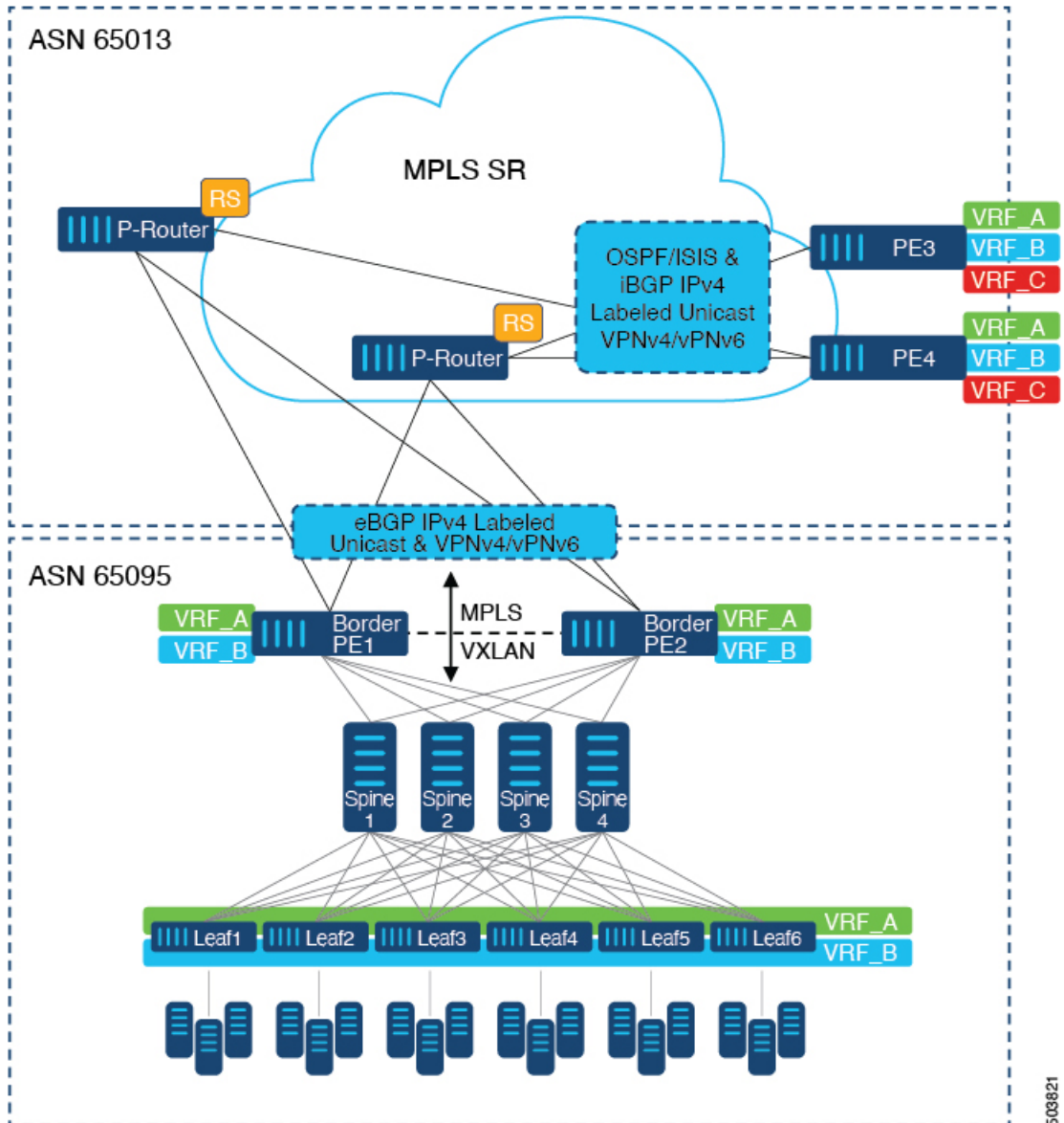
図 45: DC からコアネットワークドメインへの分離を使用したトポロジ
