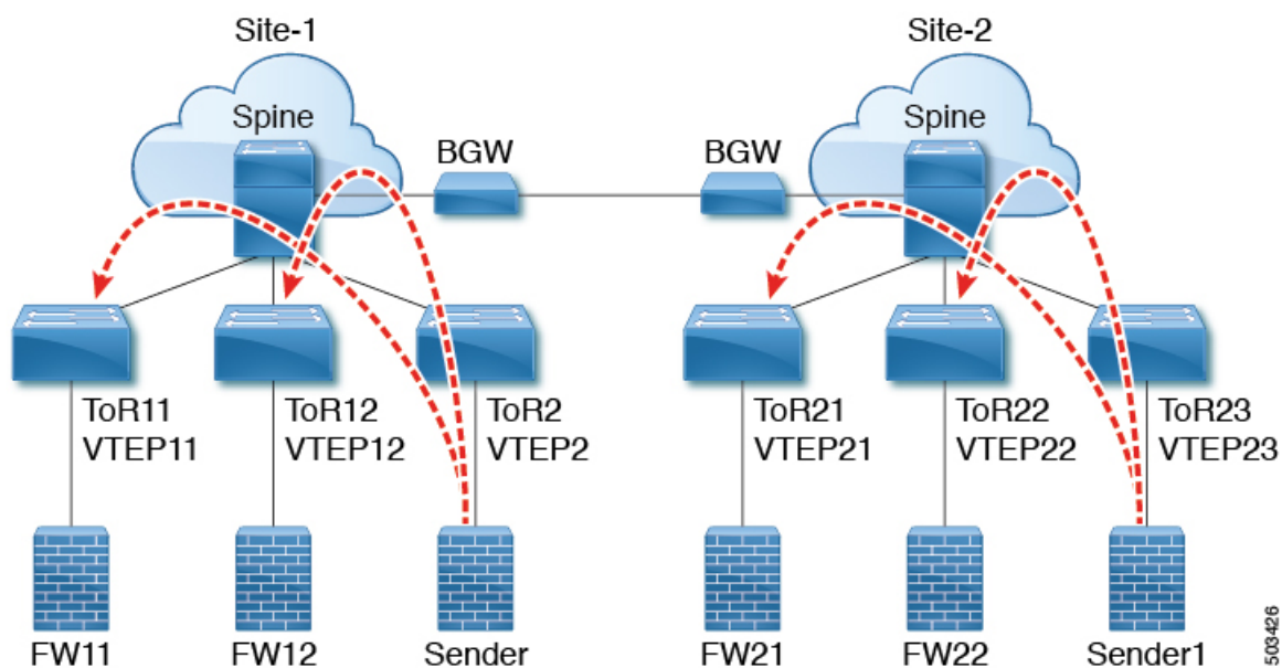
図 63: マルチサイトトポロジの VNF
