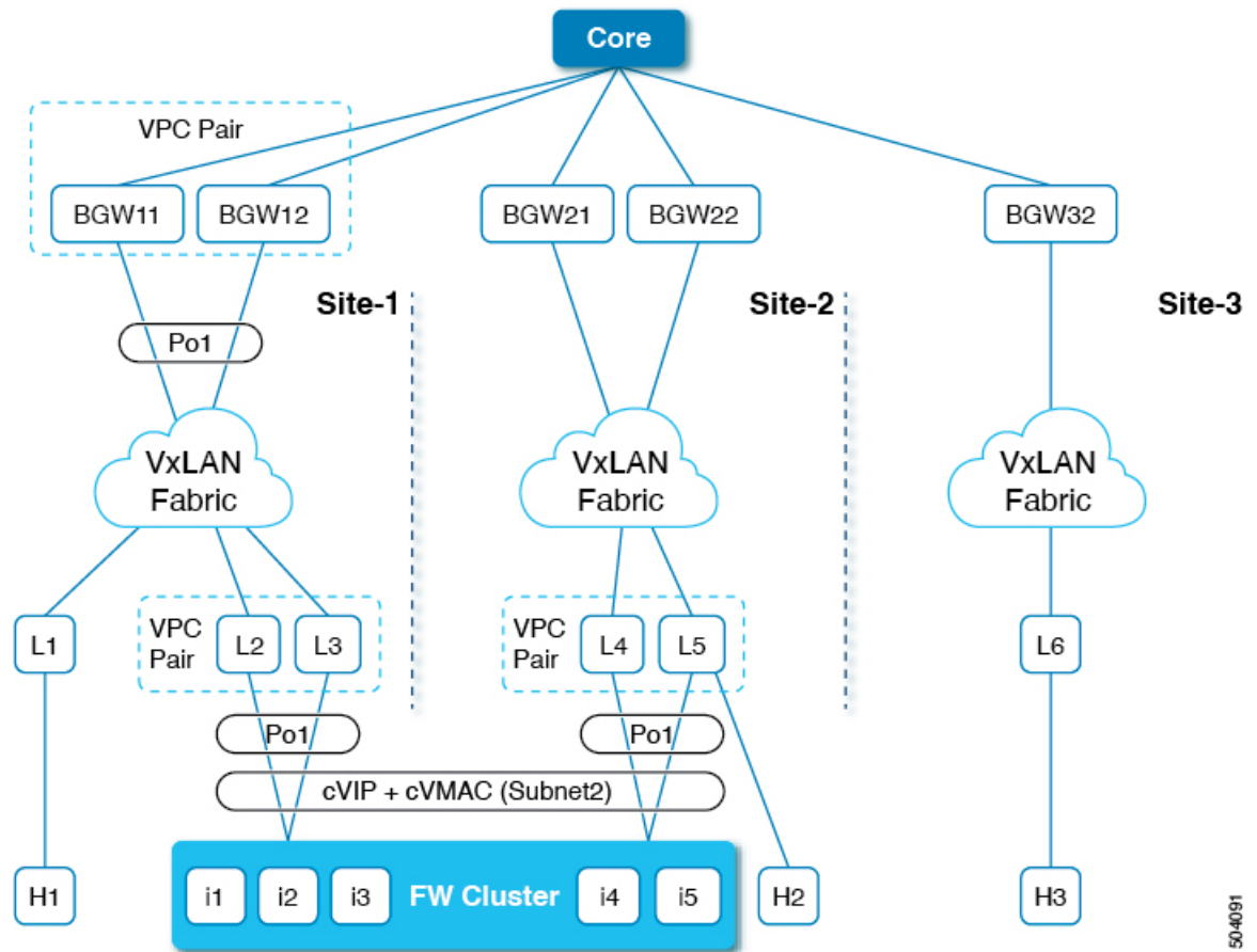
図 59: VXLAN EVPNによるファイアウォールクラスタリング
