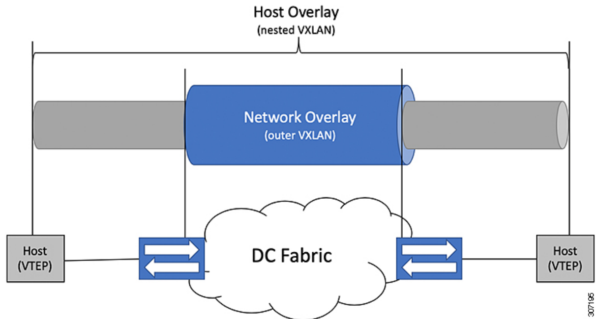
図 2: ホストオーバーレイ
