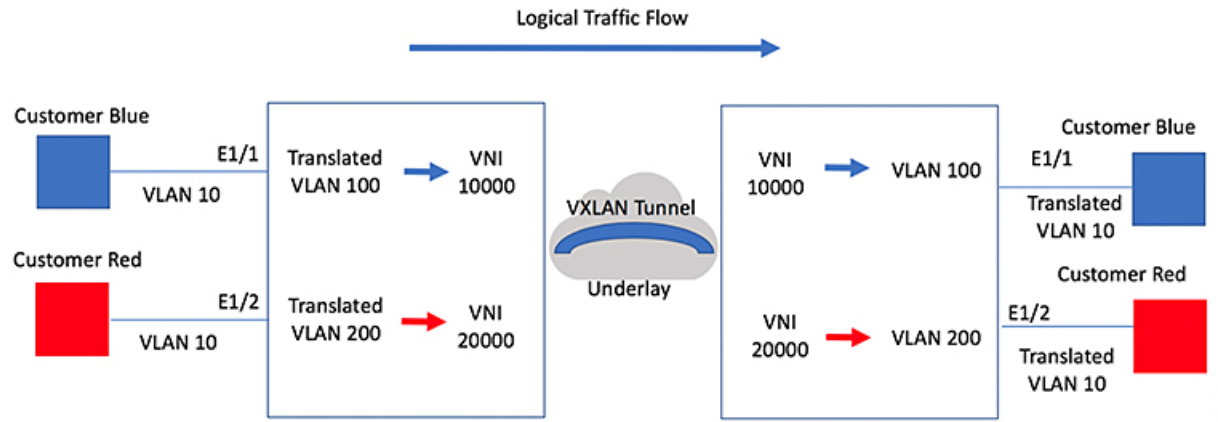
図 31: 論理的トラフィック フロー
