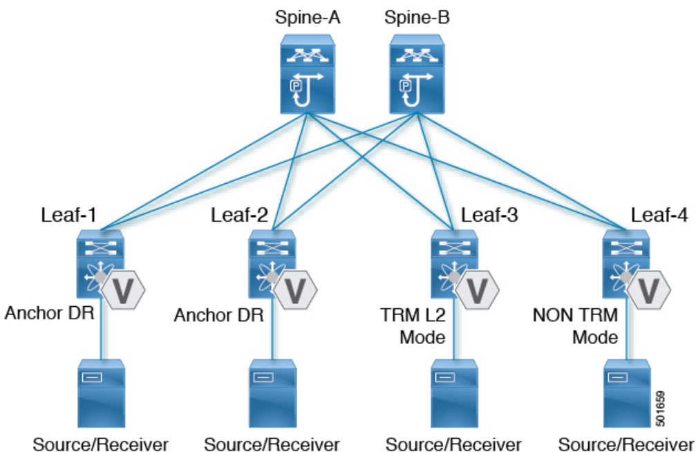
図 29: TRM レイヤ 2/レイヤ 3 混合モード
