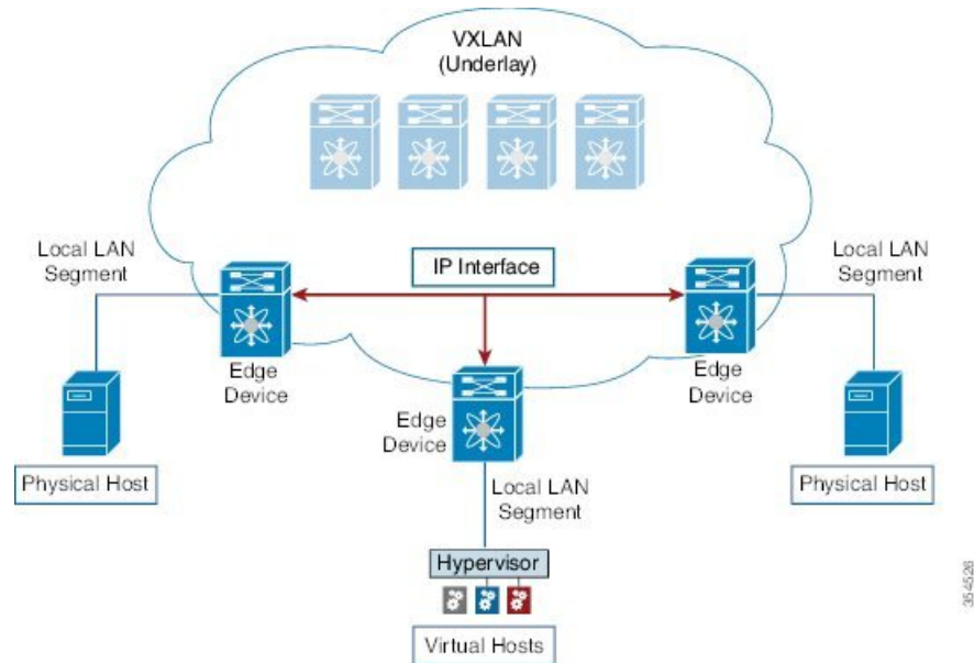
図 5: アンダーレイの概要
