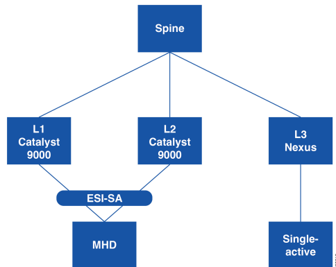
図 25: ESI シングルアクティブ マルチホーミング
