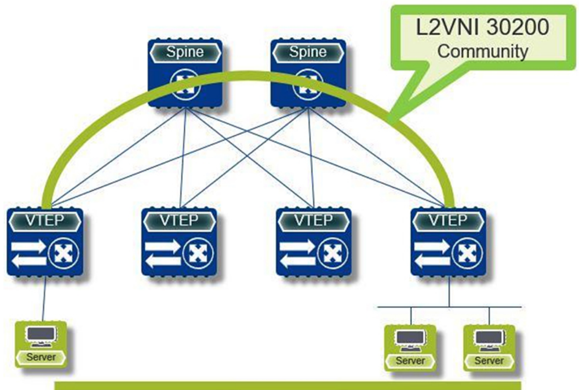
図 32: L2VNI 30200 コミュニティ
