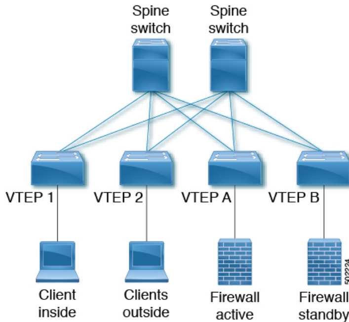
図 53: ファイアウォール接続を使用したトポロジの概要
