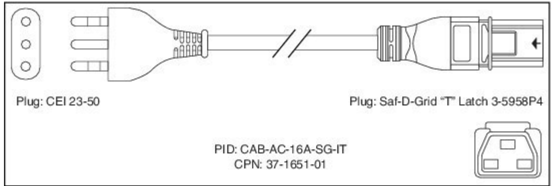
図 83: CAB-AC-16A-SG-IT 電源コード
