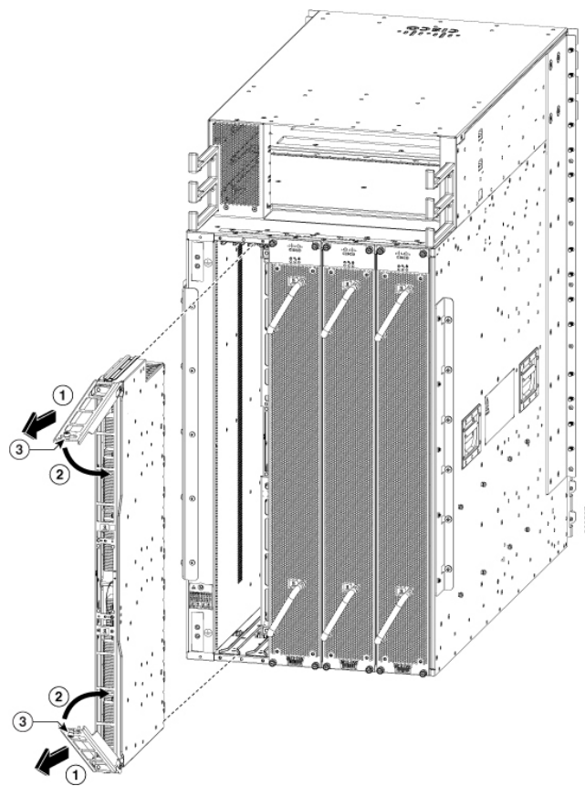
図 132: シャーシからのファブリック カードの取り外し
