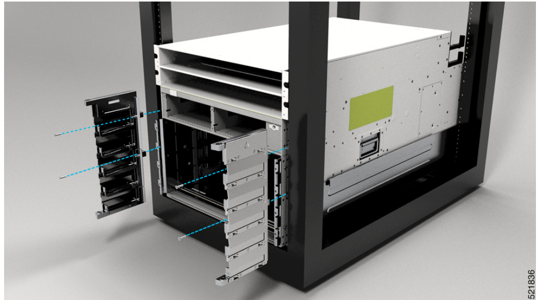
図 37: 8804 シャーシのケーブル管理ブラケット
