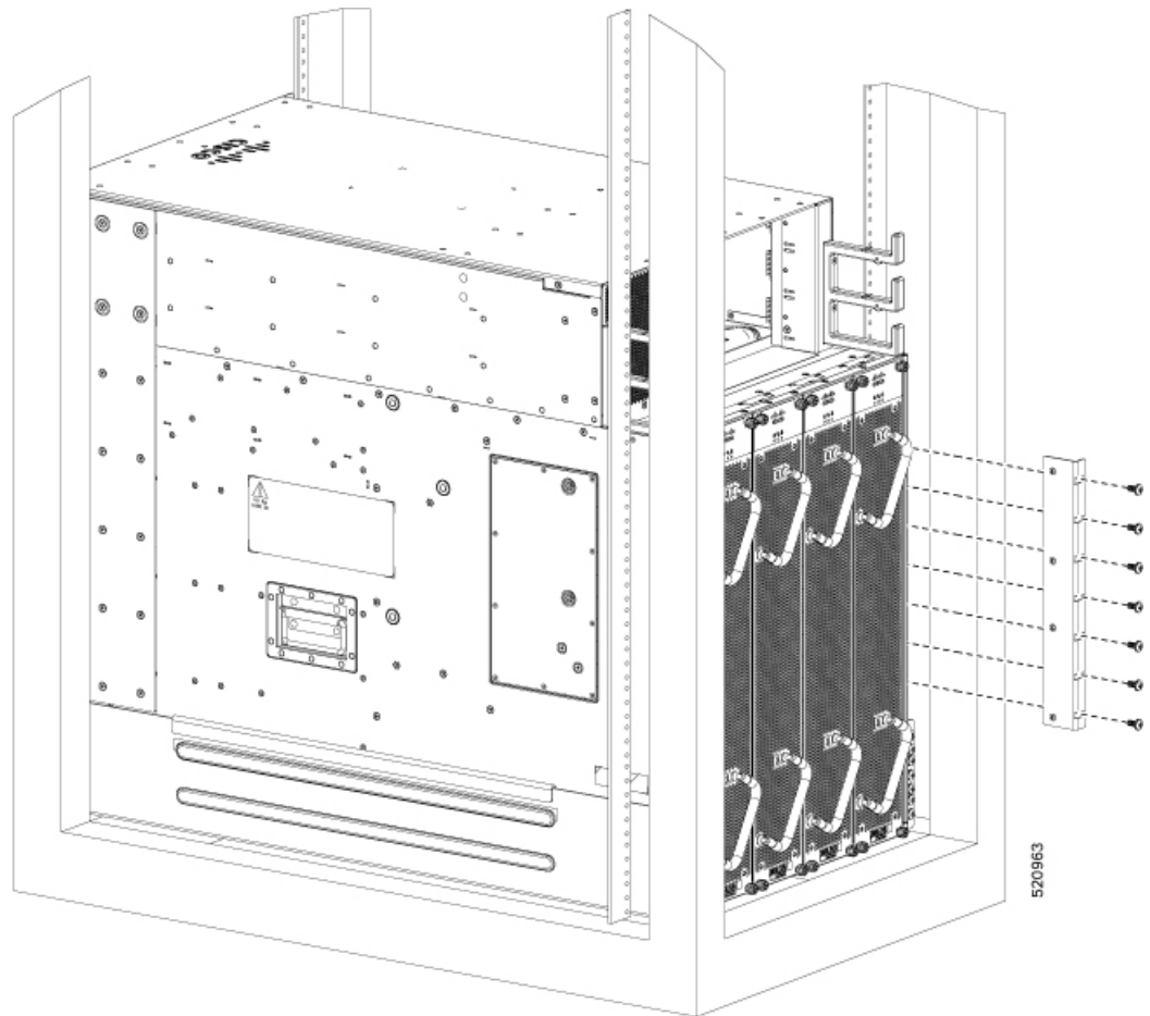
図 26: ラックへの 8808 シャーシの取り付け (右左背面図)
