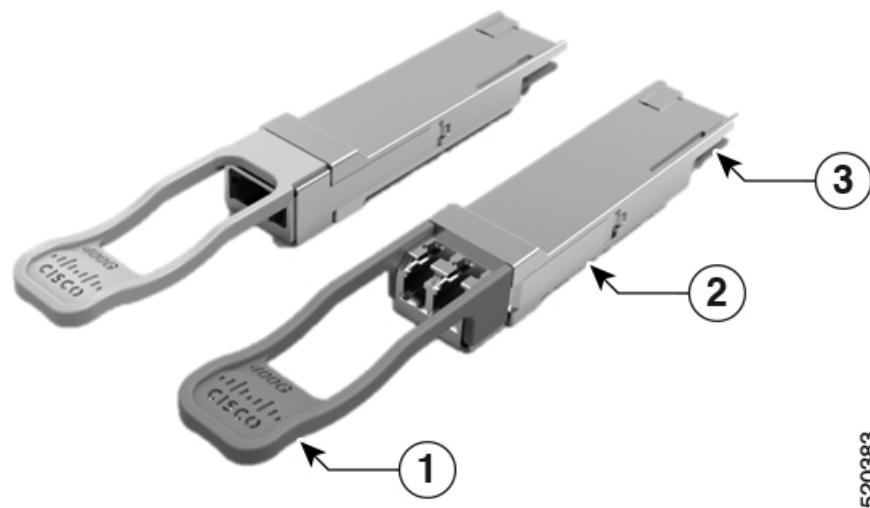
図 104: 400 ギガビット QSFP-DD トランシーバモジュール
