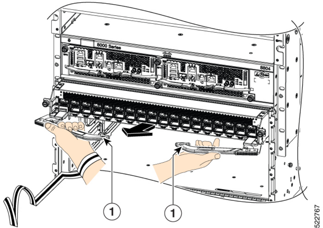
図 126: シャーシからのラインカードの引き出し
