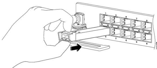
図 101: ポートへのベールクラスプ SFP28 または SFP+ モジュールの取り付け
