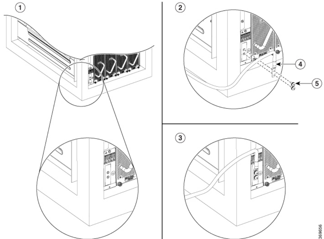
図 33: シャーシの接地
