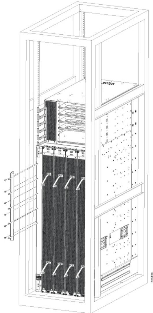
図 21: ラックへの 8818 シャーシの取り付け (左背面図)
