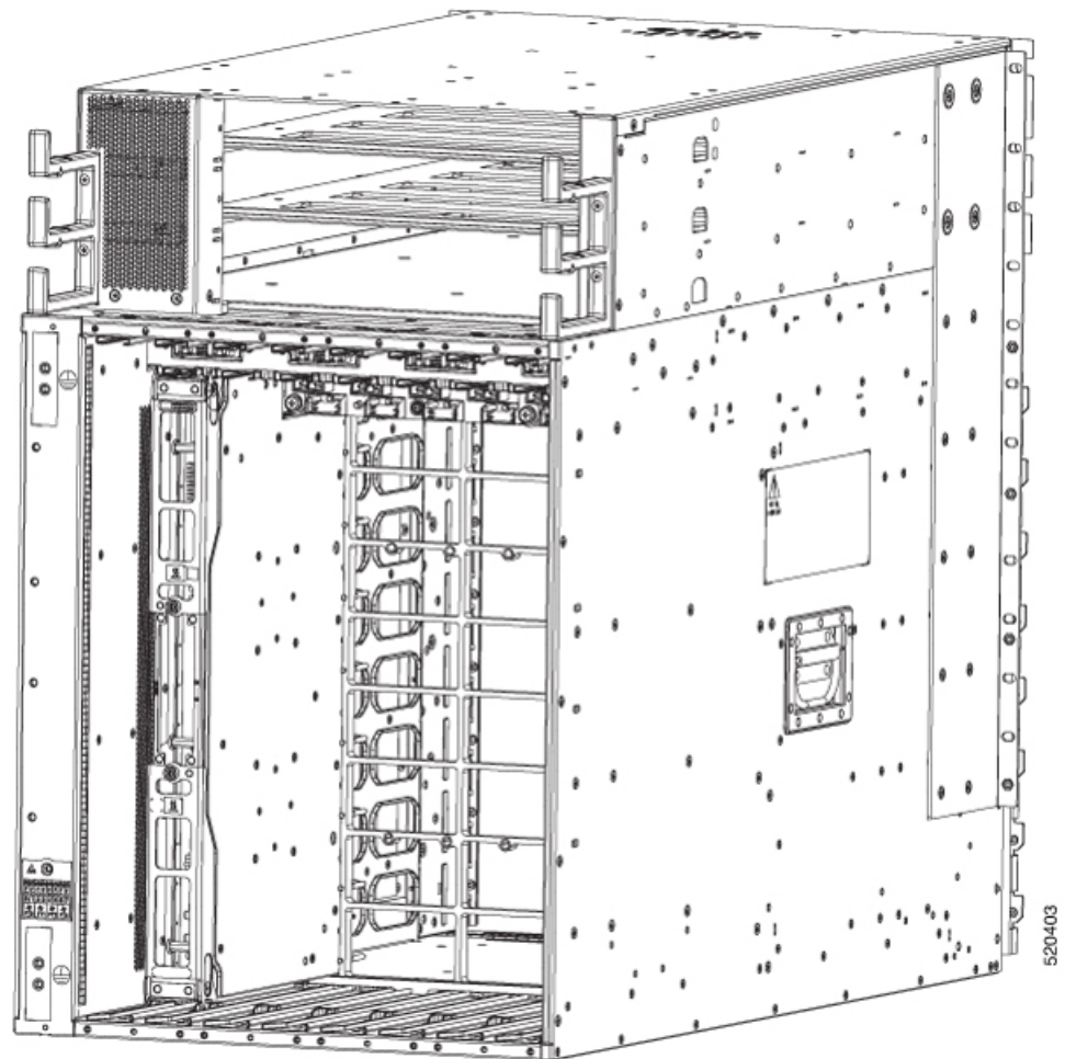
図 138: シャーシに取り付けられたファブリックカード
