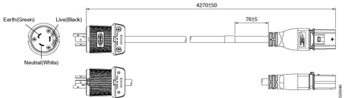
図 69: CAB-AC-30A-US4 電源コードと標準 AC 電源用プラグ
