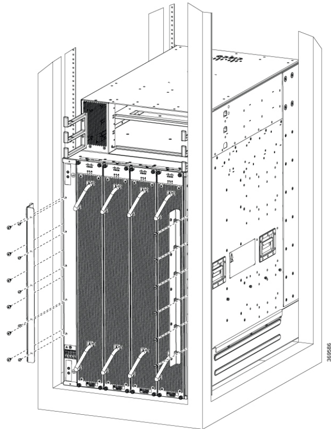
図 23: ラックへの 8812 シャーシの取り付け (左背面図)
