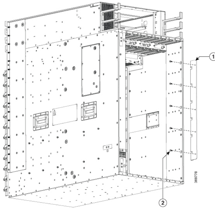
図 24: ラックへの 8812 シャーシの取り付け (右左背面図)
