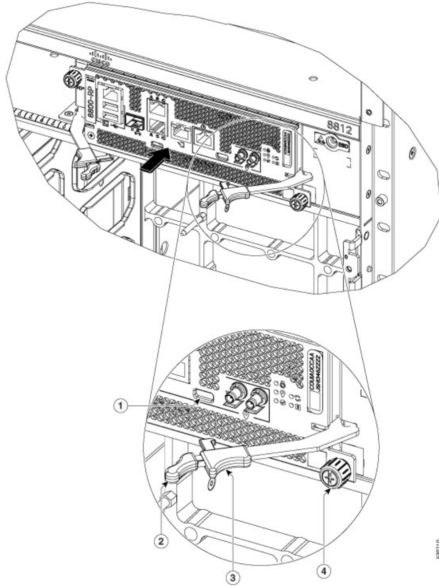
図 111: ルートプロセッサカードのコンポーネント
