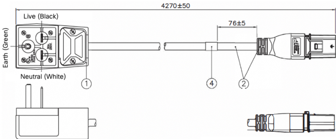
図 64: CAB-AC-30A-US1 電源コードと標準 AC 電源用プラグ
