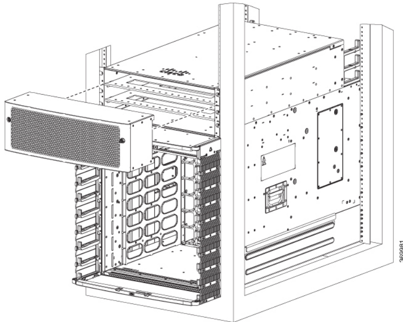
図 142: 8808 シャーシの電源ベゼル
