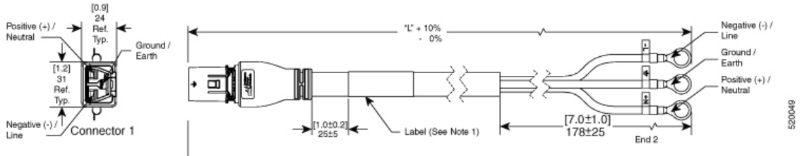
図 73: CAB-AC-32A-CHN 電源コードと標準 AC 電源用プラグ
