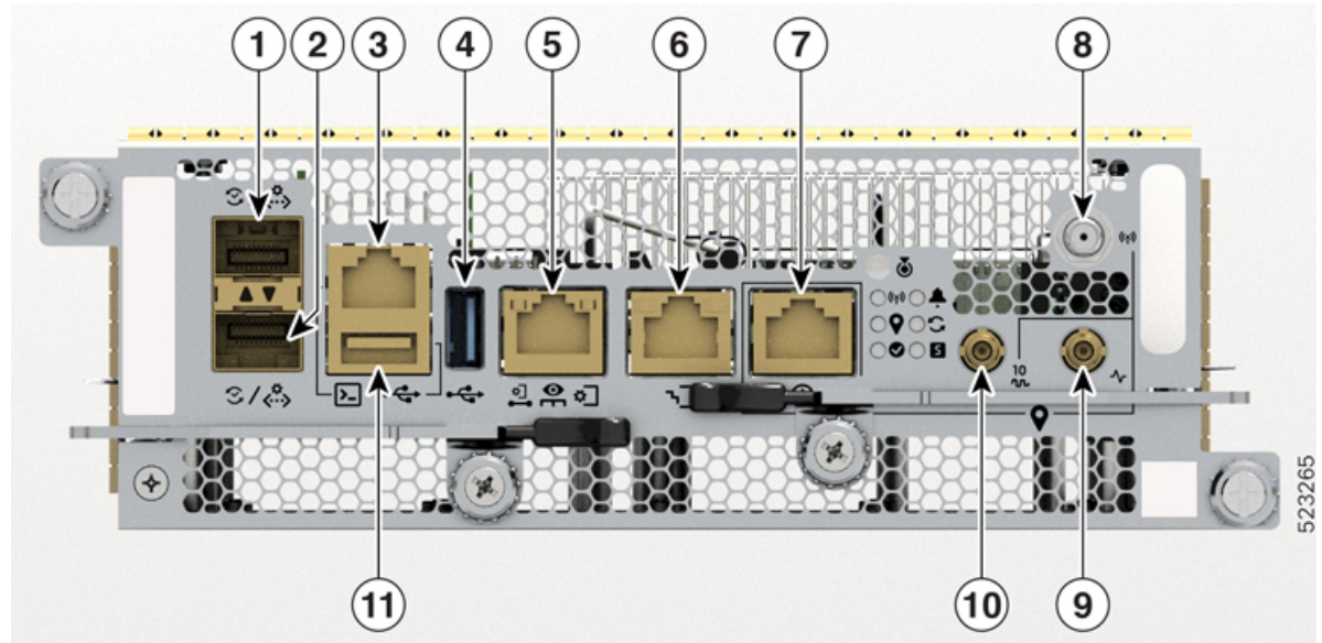
図 5: ルートプロセッサ - 8800-RP2
