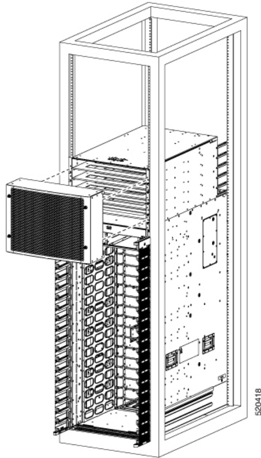
図 140: 8818 シャーシの電源ベゼル
