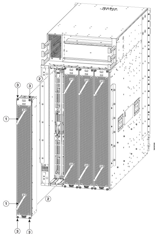
図 131: シャーシからのファントレイの取り外し
