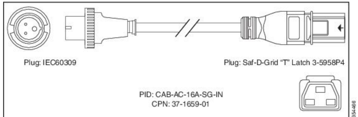
図 81: CAB-AC-16A-SG-IN 電源コード
