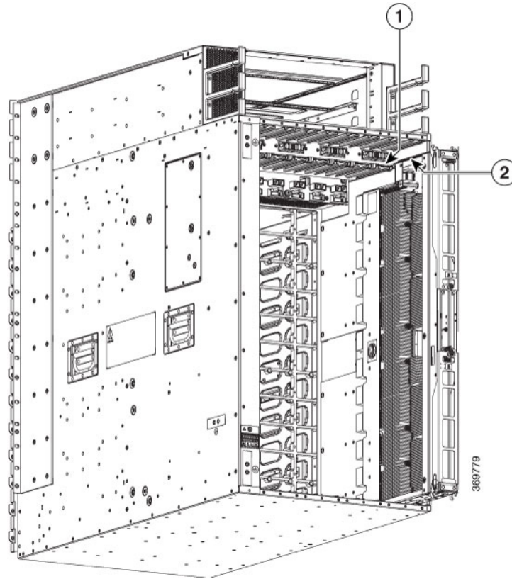
図 137: ファブリックカードの取り付け - 8808-FC1
