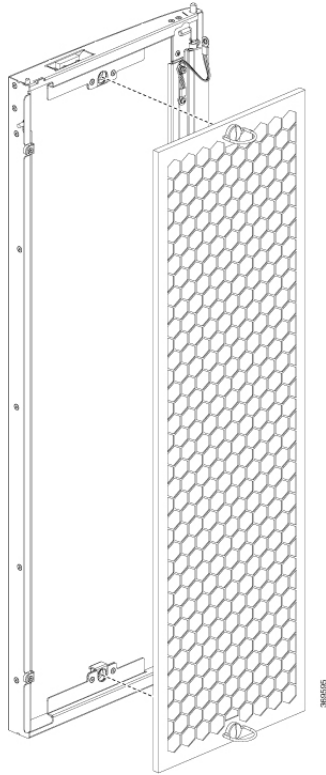
図 110: エアフィルタの交換
