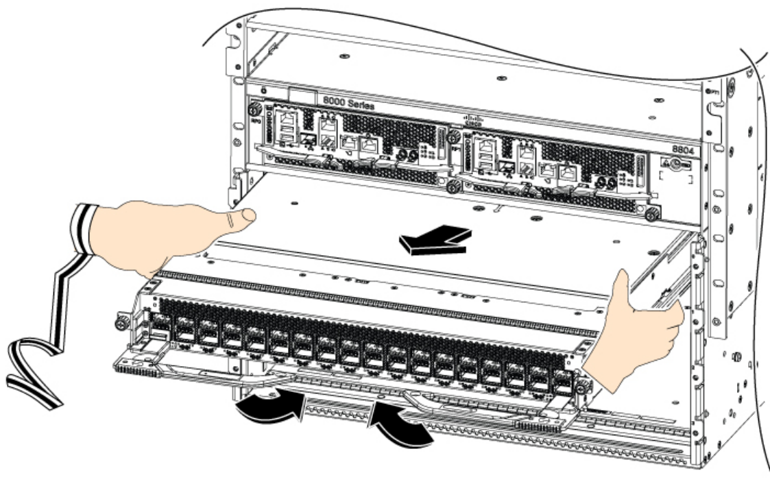
図 127: シャーシからのラインカードの取り外し
