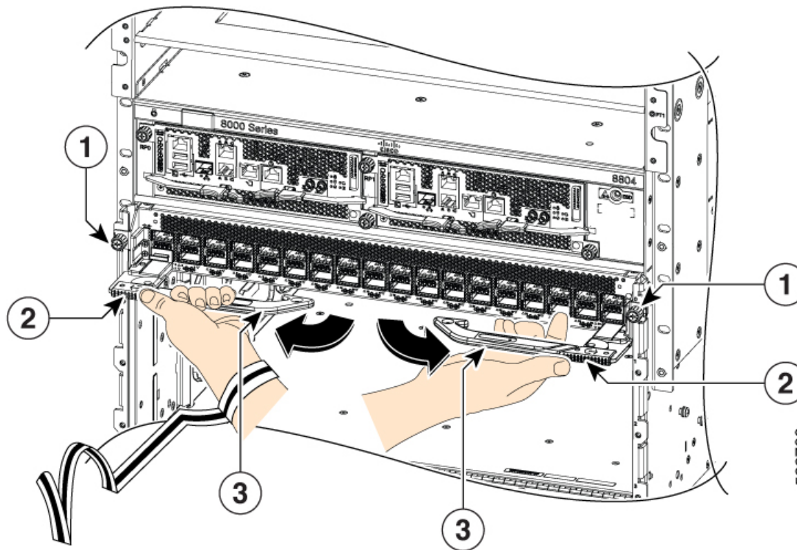
図 125: イジェクトレバーラッチのスライド
