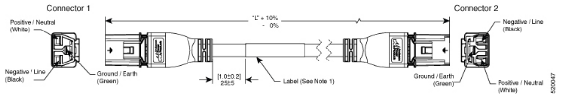
図 69: CAB-AC-30A-US4 電源コードと標準 AC 電源用プラグ
