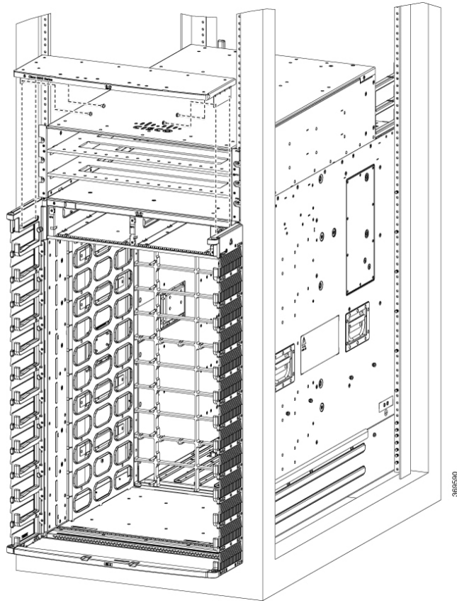
図 45: 8812 シャーシの上部フード
