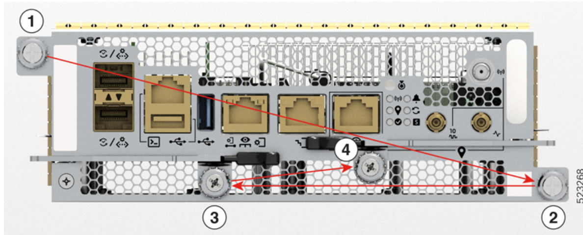
図 118: ネジを締める順序
