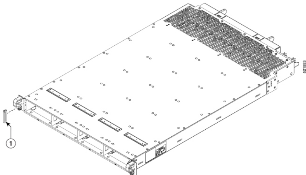
図 57: 電源モードスイッチのカバー
