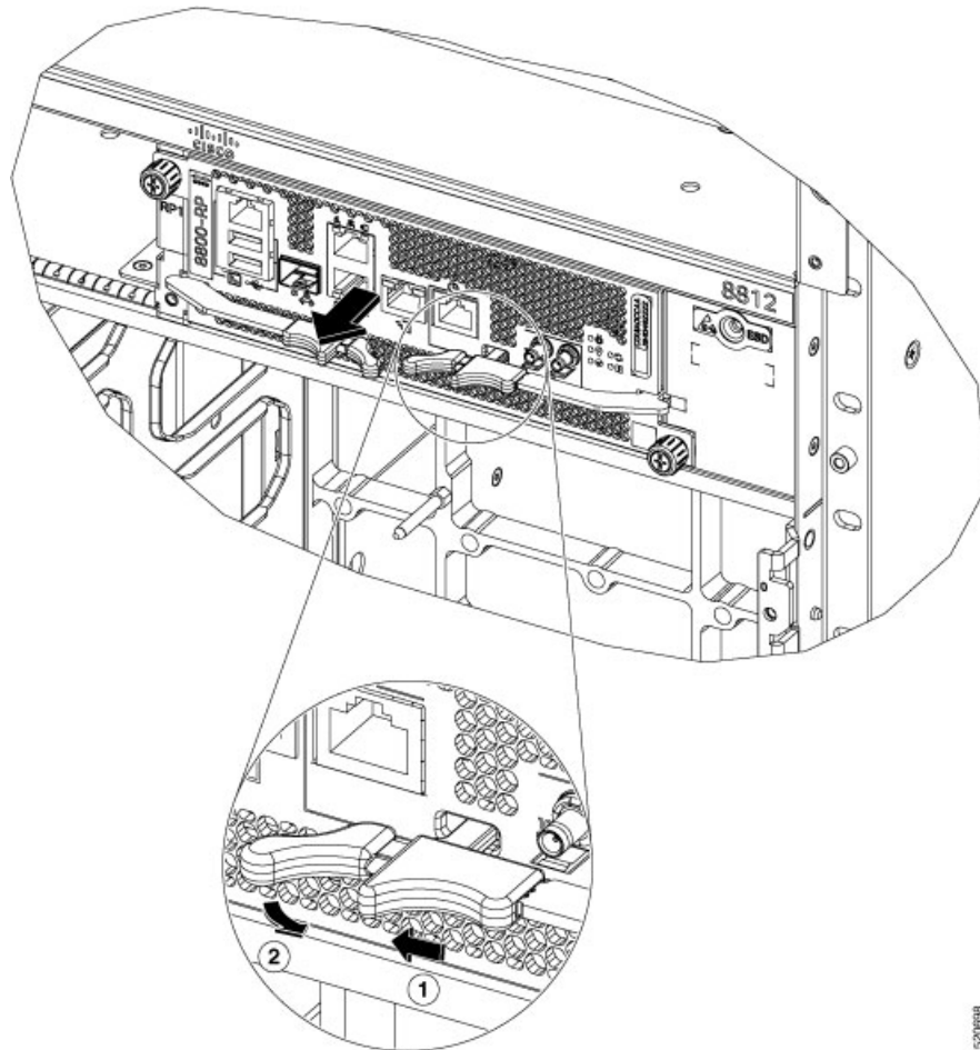
図 112: シャーシからのルート プロセッサ カードの取り外し
