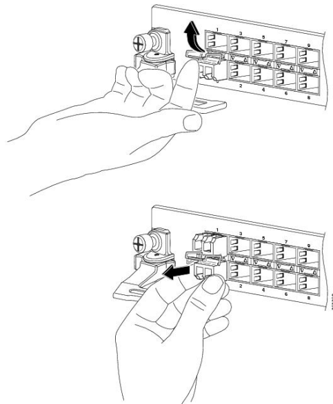
図 102: ベールクランプ SFP または SFP+ モジュールの取り外し
