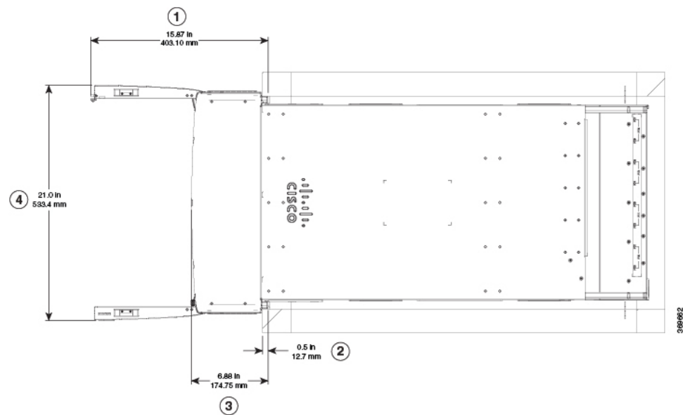
図 9: シャーシの扉周りに必要なスペース
