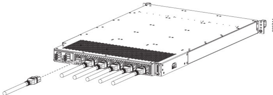
図 62: HVAC 電源接続
