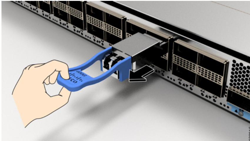
図 109: Cisco 8202-32FH-M ルータからの QSFP トランシーバモジュールの取り外し
