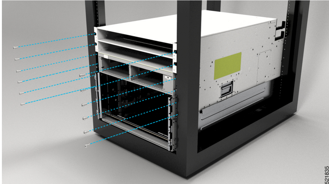
図 20: ラックへの 8804 シャーシの取り付け (前面)
