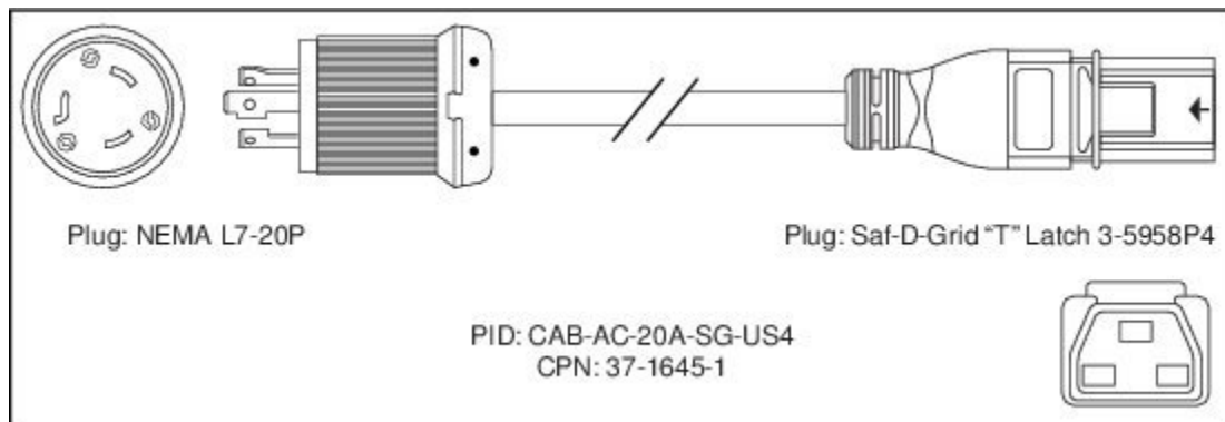
図 93: CAB-AC-20A-SG-C20 電源コード
