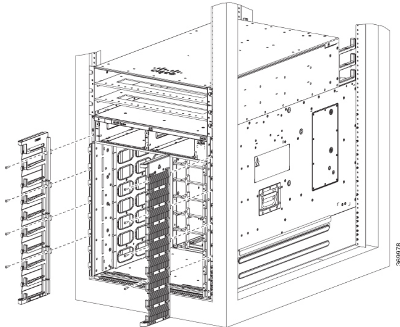
図 36: 8808 シャーシのケーブル管理ブラケット
