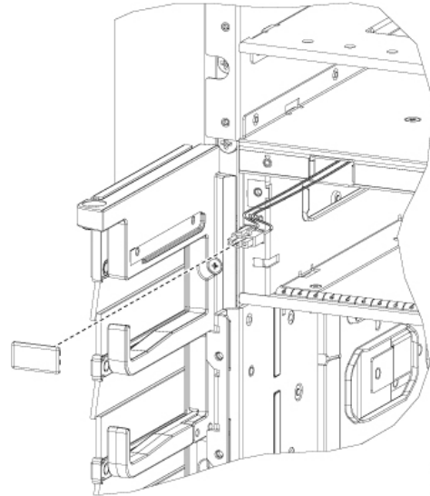
図 42: コネクタキャップの取り外し
