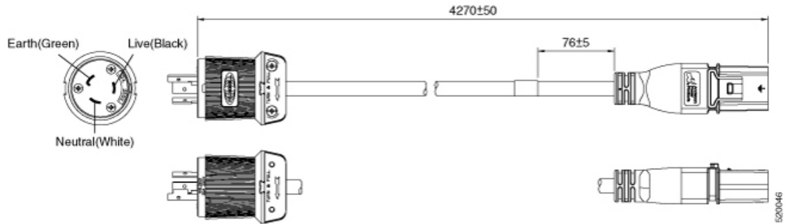
図 66: CAB-DC-30A-US1 電源コードと HVDC 電源用プラグ
