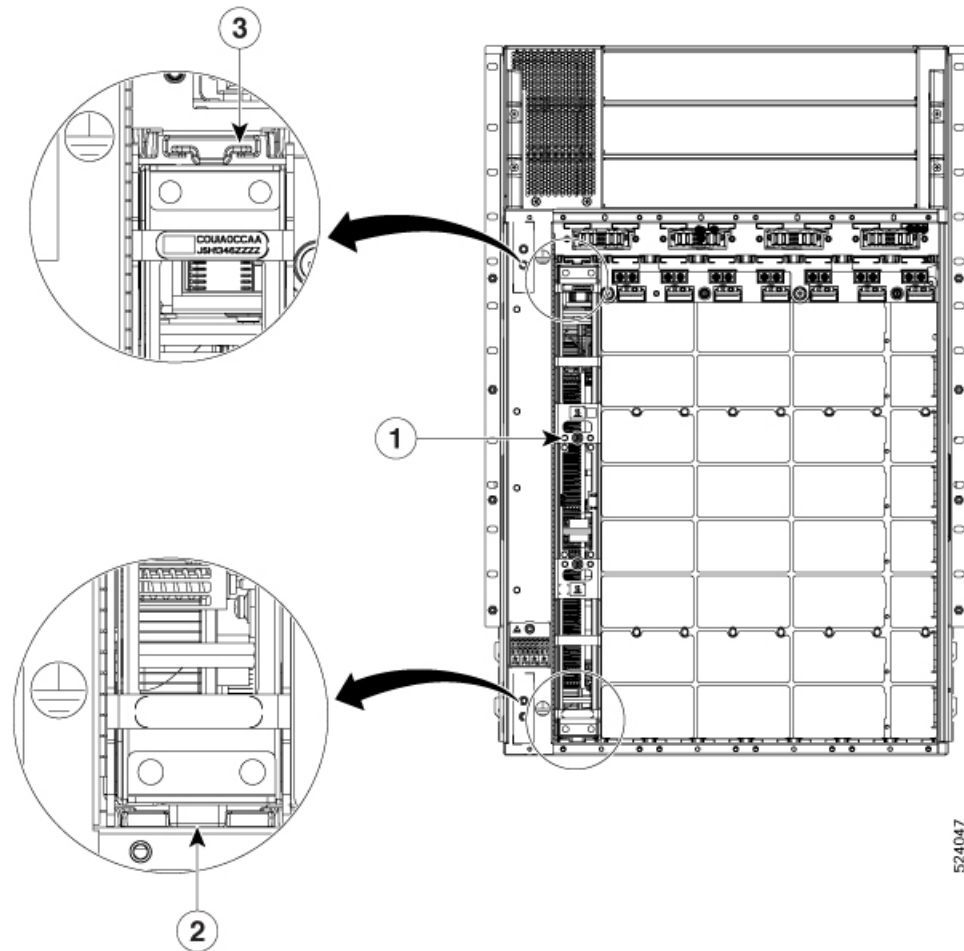
図 135: ファブリックカードの取り付け - 8808-FC1
