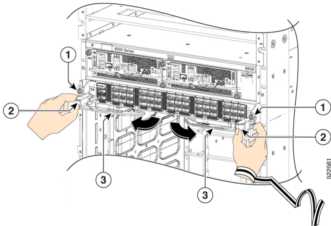
図 119: イジェクトボタンを押す
