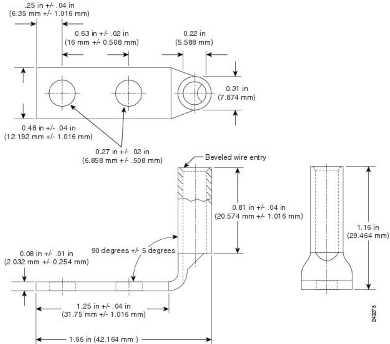
図 58: 一般的な DC 電源コードの端子
