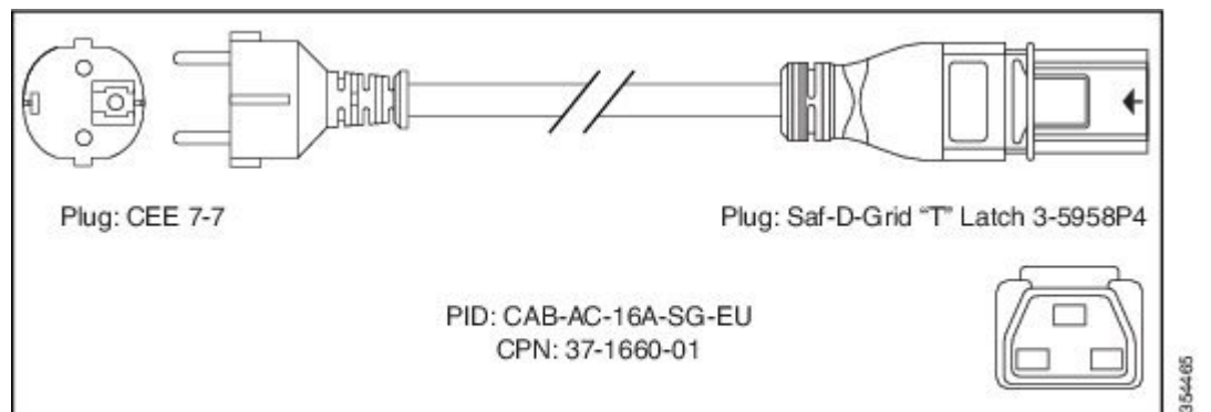
図 79: CAB-AC-16A-SG-EU 電源コード
