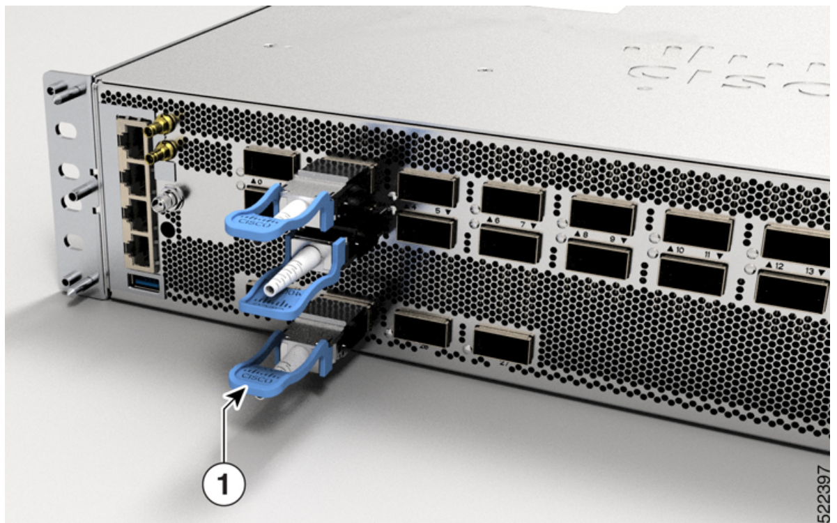
図 109: Cisco 8202-32FH-M ルータからの QSFP トランシーバモジュールの取り外し
