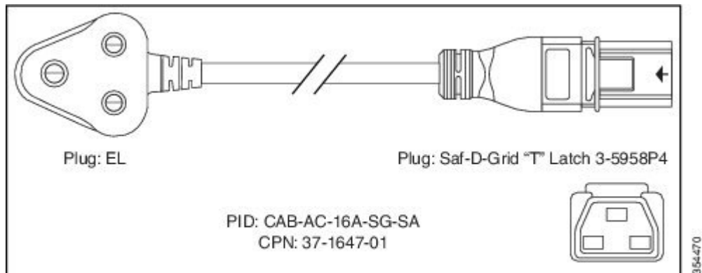
図 85: CAB-AC-16A-SG-SA 電源コード
