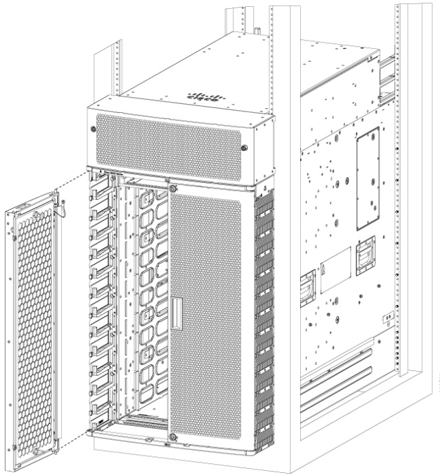
図 51: 8808 シャーシへの前面扉の取り付け
