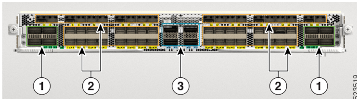
図 2: 88-LC1-52Y8H4F-EM ラインカード
