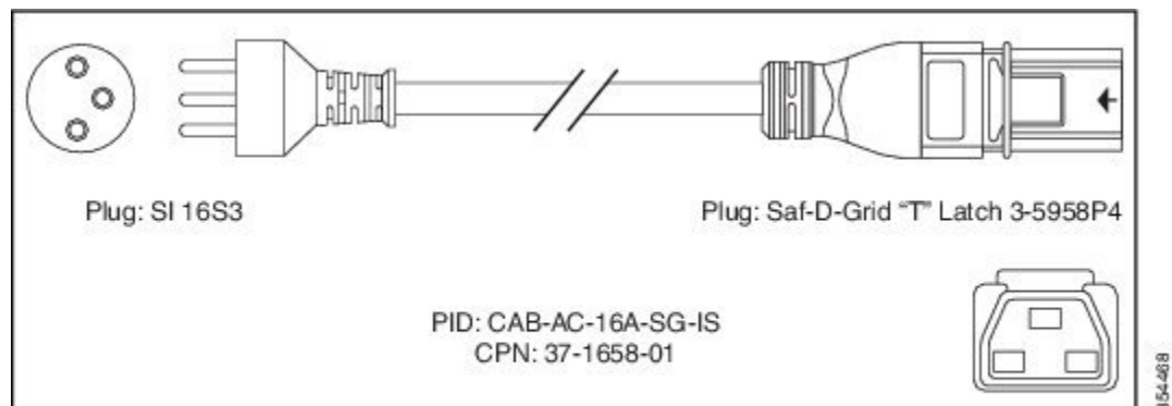
図 82: CAB-AC-16A-SG-IS 電源コード
