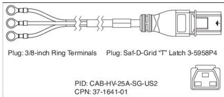
図 94: CAB-HV-25A-SG-US2 電源コード
