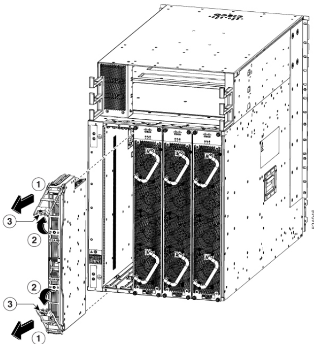
図 133: シャーシからのファブリックカードの取り外し - 8808-FC1
