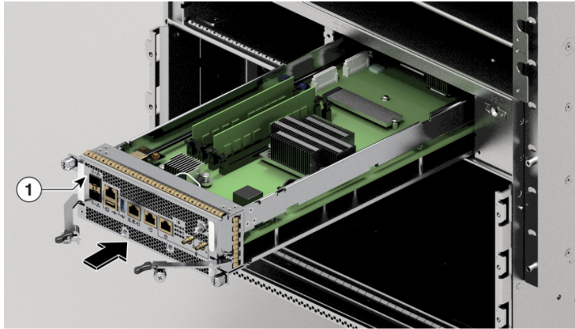
図 116: RP カードをシャーシと平行に固定する
