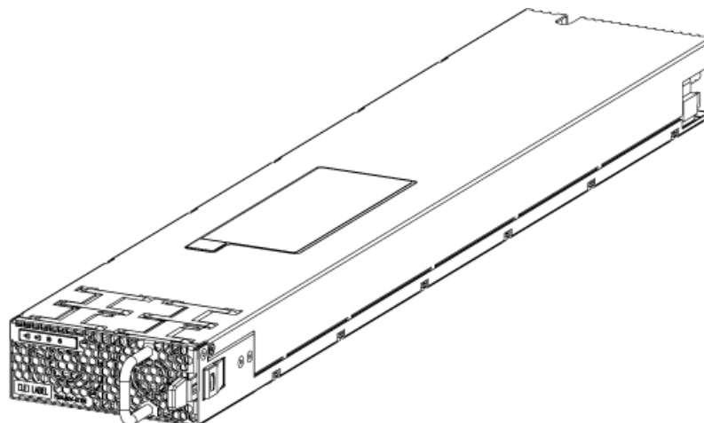
図 55: PSU4.8KW-DC100
