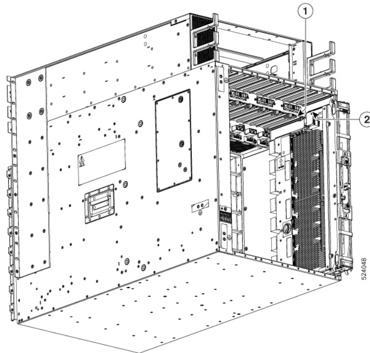
図 137: ファブリックカードの取り付け - 8808-FC1
