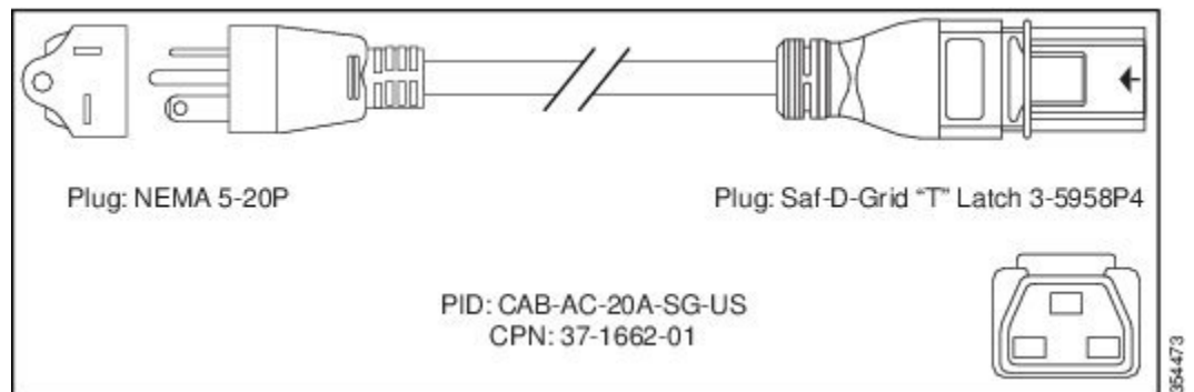
図 88: CAB-AC-20A-SG-US 電源コード
