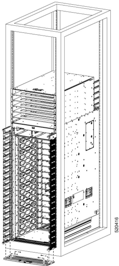
図 38: 8818 シャーシの下部カバー
