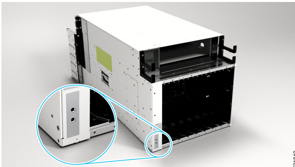
図 32: Cisco 8804 シャーシのシャーシ接地レセプタクル
