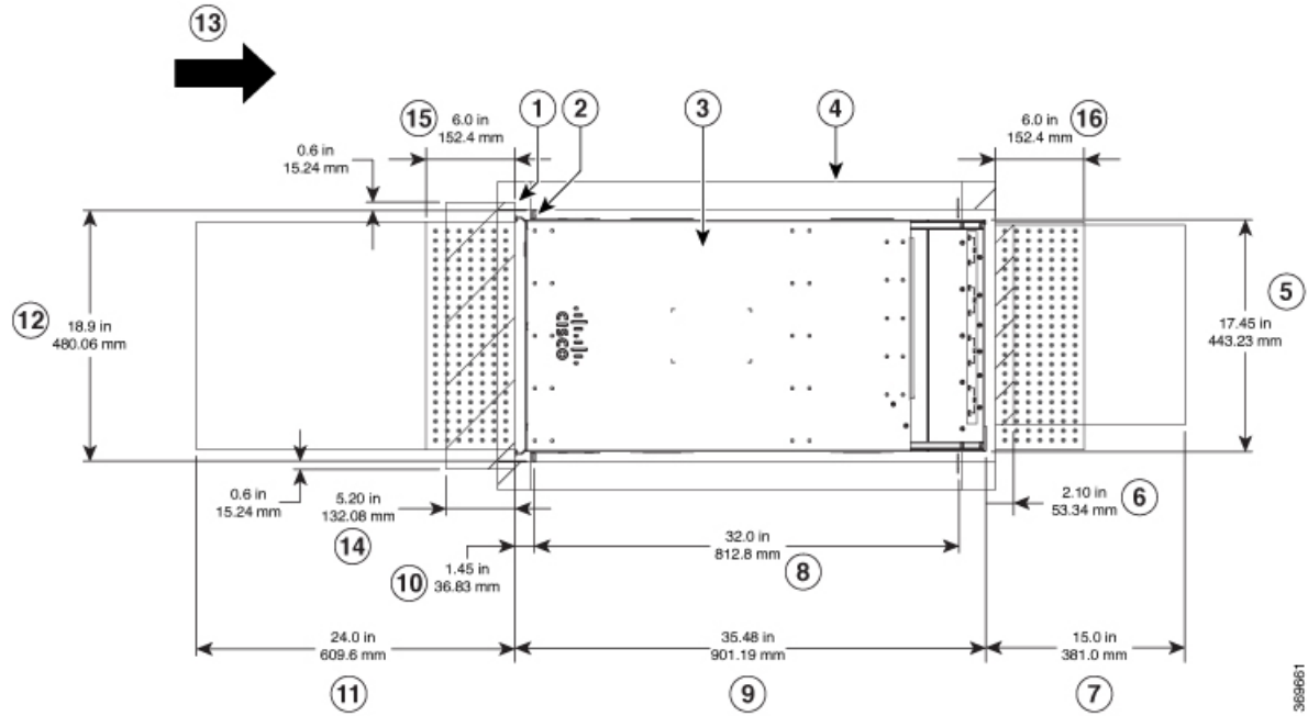
図 8: シャーシの周りに必要なスペース
