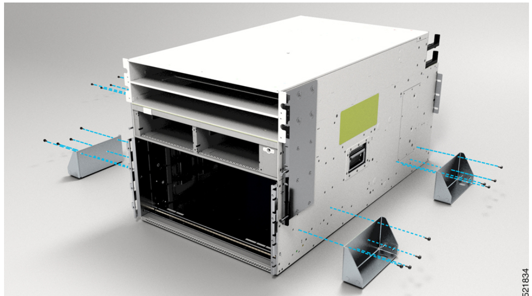
図 13: 8804 シャーシからの輸送用ブラケットの取り外し
