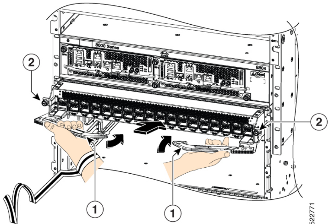
図 130: イジェクトレバーを閉じる
