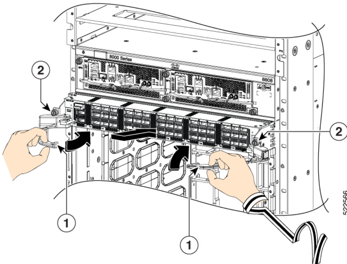
図 124: イジェクトレバーを閉じる
