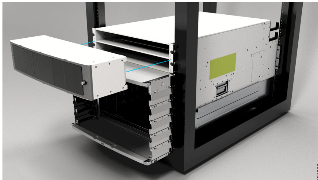
図 143: 8804 シャーシの電源ベゼル
