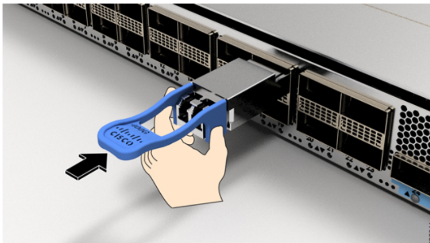
図 105: QSFP トランシーバモジュールの取り付け
