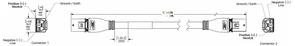
図 72: CAB-DC-32A-EU2 電源コードと HVDC 電源用プラグ
