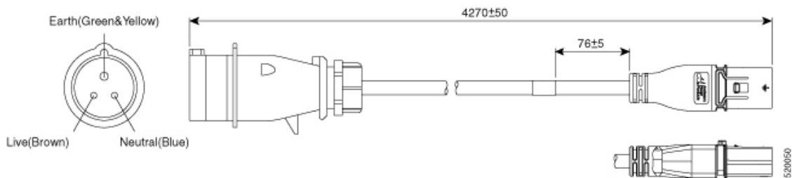
図 74: CAB-AC-32A-KOR 電源コードと標準 AC 電源用プラグ
