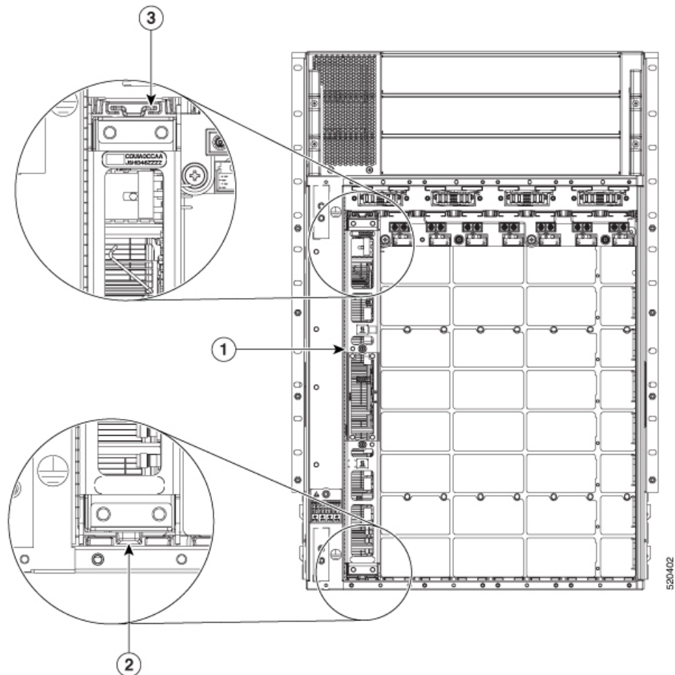
図 134: ファブリックカードの取り付け
