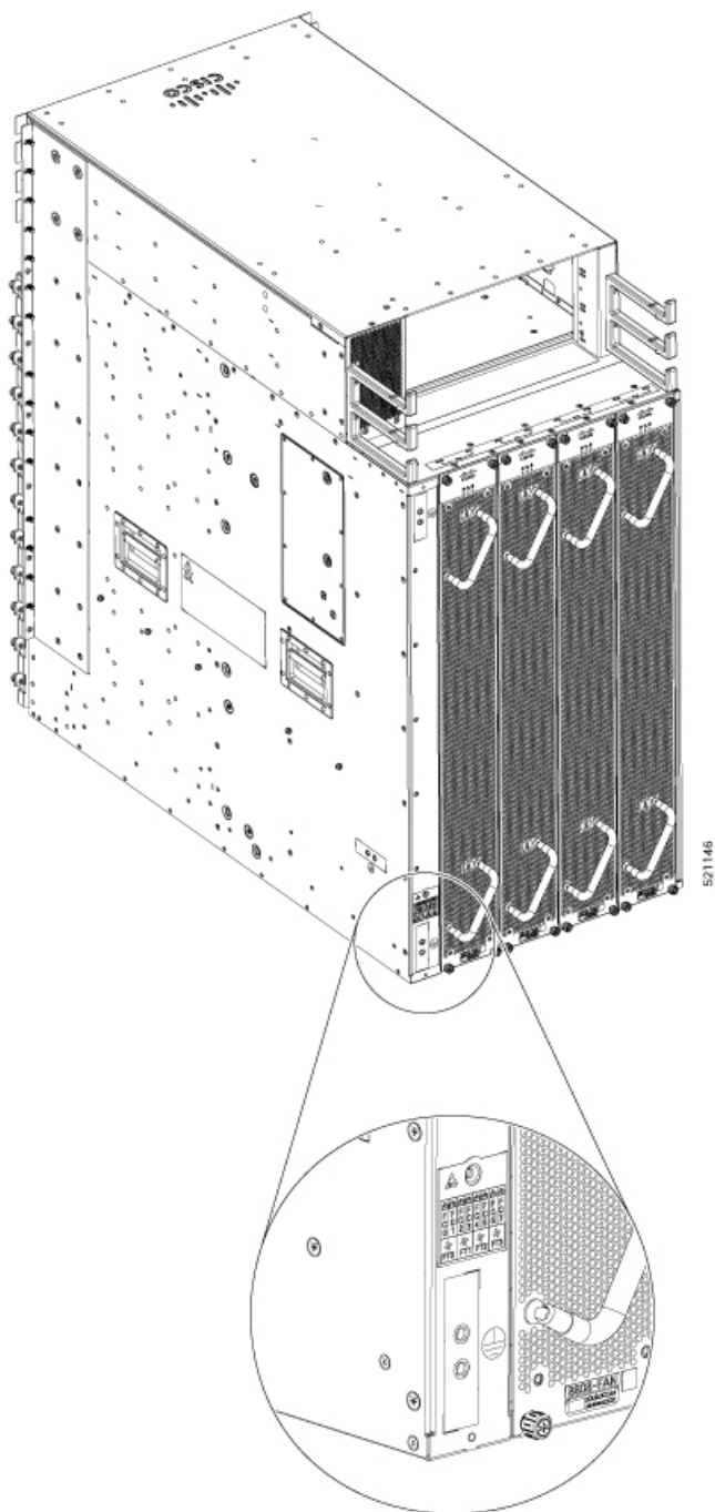
図 30: Cisco 8812 シャーシのシャーシ接地レセプタクル
