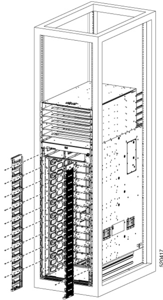
図 34: 8818 シャーシのケーブル管理ブラケット
