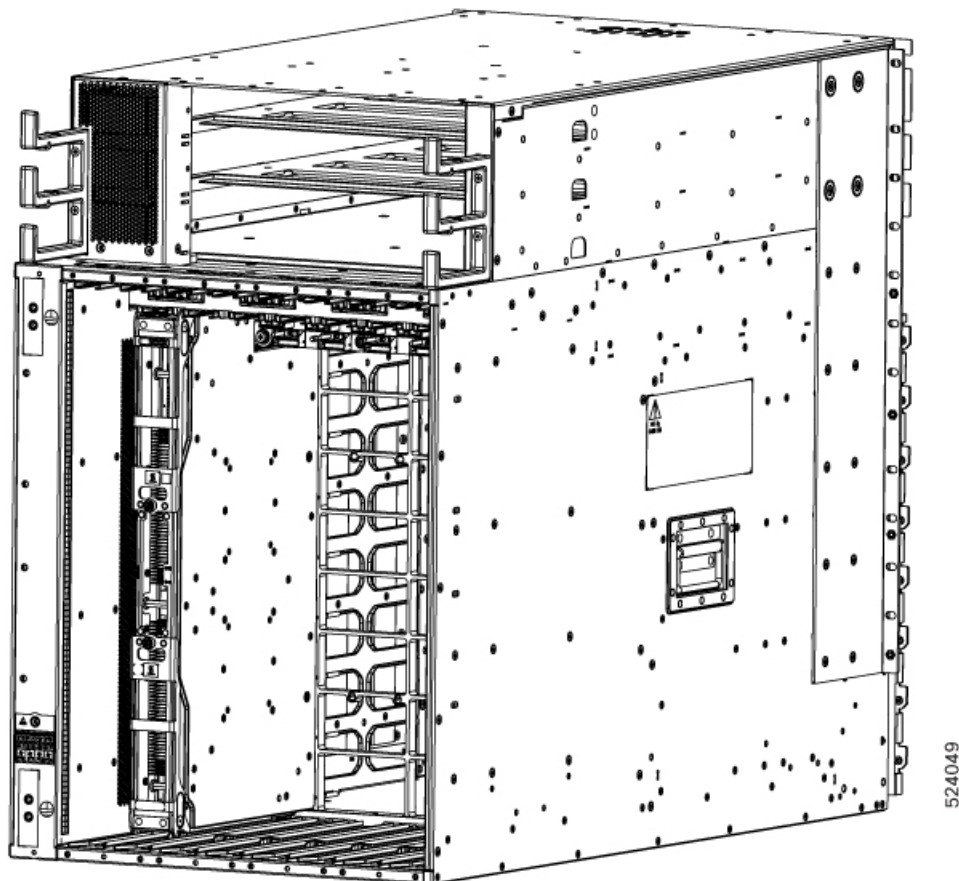
図 139: シャーシに取り付けられたファブリックカード - 8808-FC1
