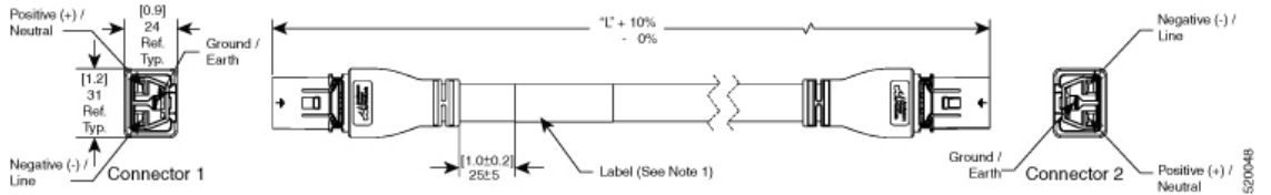
図 71: CAB-DC-32A-EU1 電源コードと HVDC 電源用プラグ
