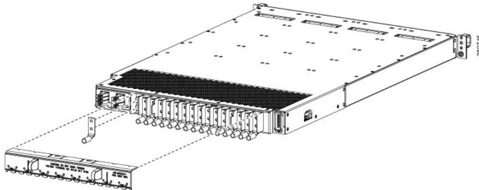
図 60: DC 電源の接続
