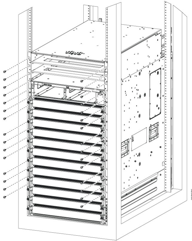
図 18: ラックへの 8812 シャーシの取り付け (前面)
