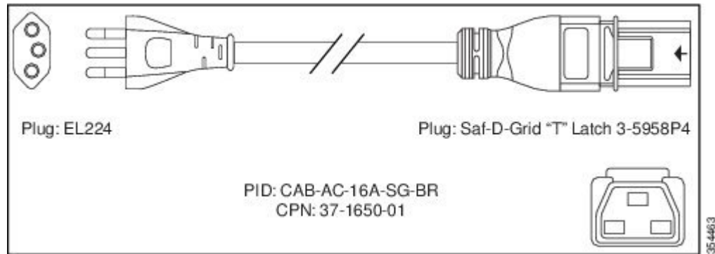
図 78: CAB-AC-16A-SG-CH 電源コード
