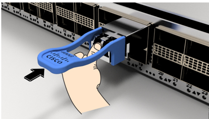
図 106: QSFP トランシーバモジュールの装着
