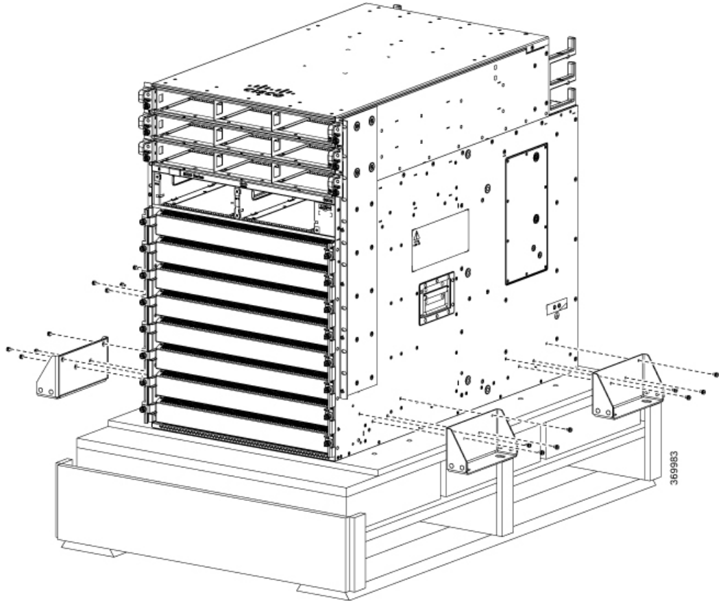
図 13: 8804 シャーシからの輸送用ブラケットの取り外し
