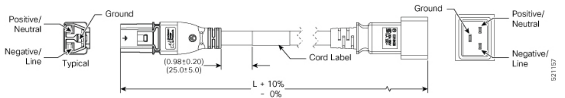
図 97: CAB-AC-20A-NA 電源コード
