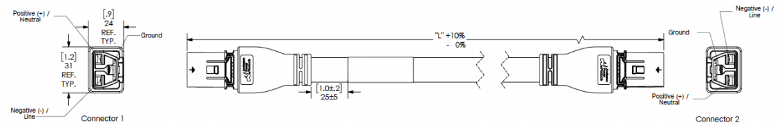
図 67: CAB-DC-30A-US2 電源コードと HVDC 電源用プラグ
