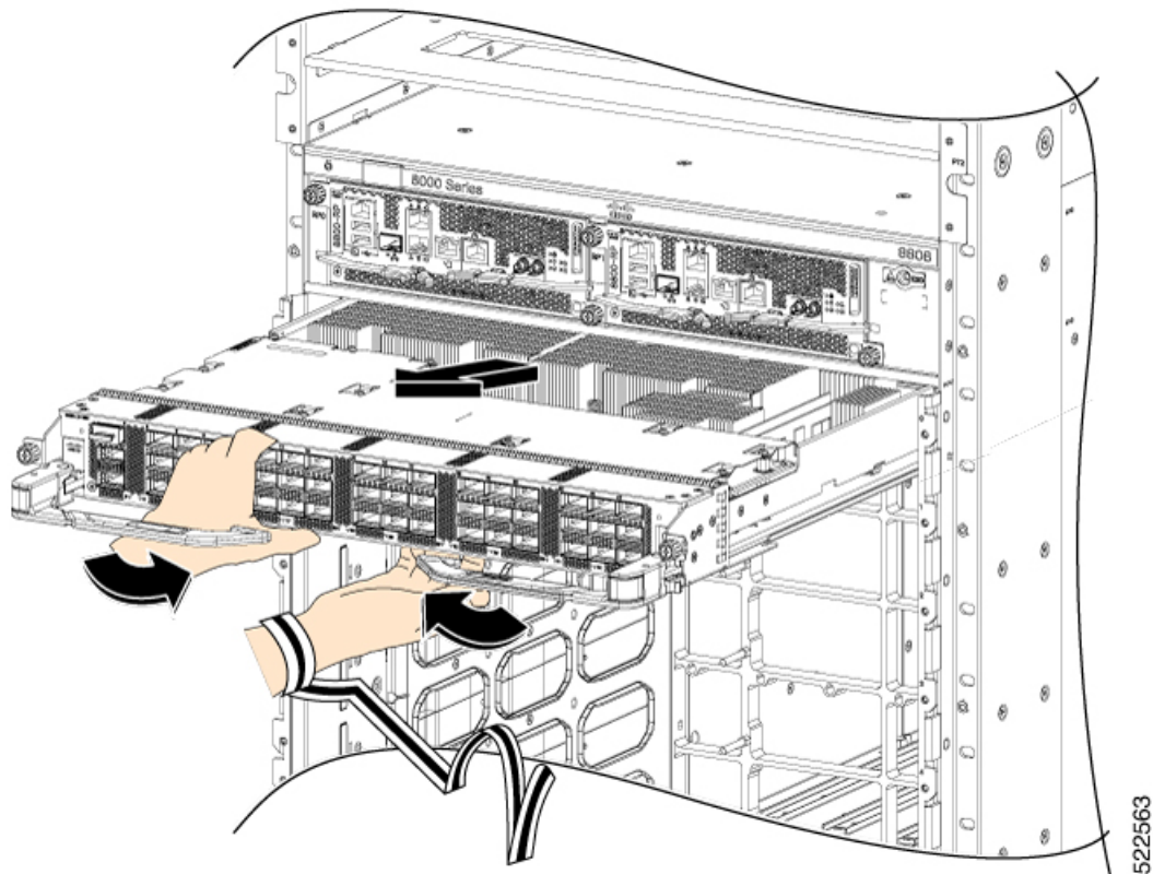
図 121: シャーシからのラインカードの取り外し
