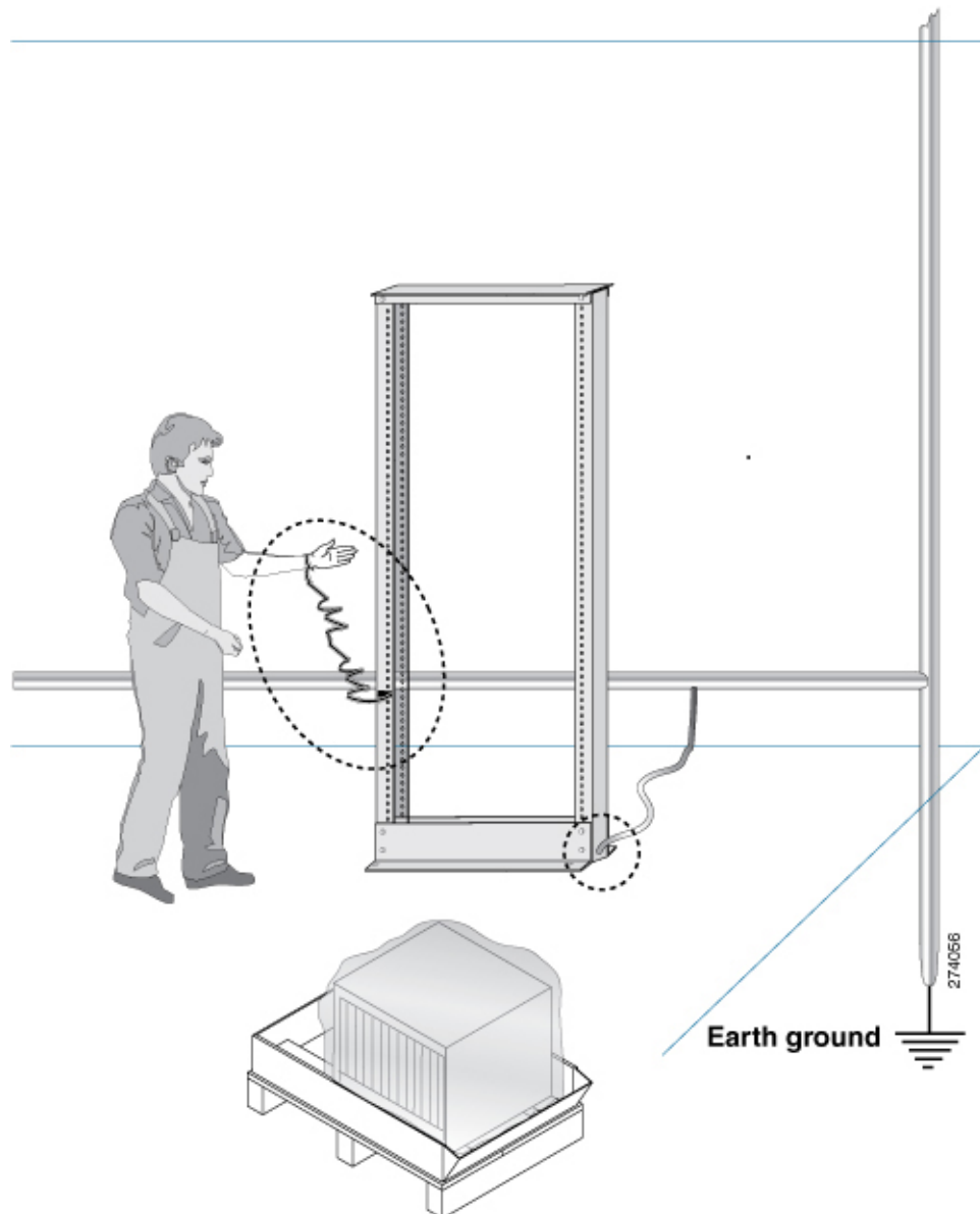
図 7: 静電気防止用ストラップの着用
