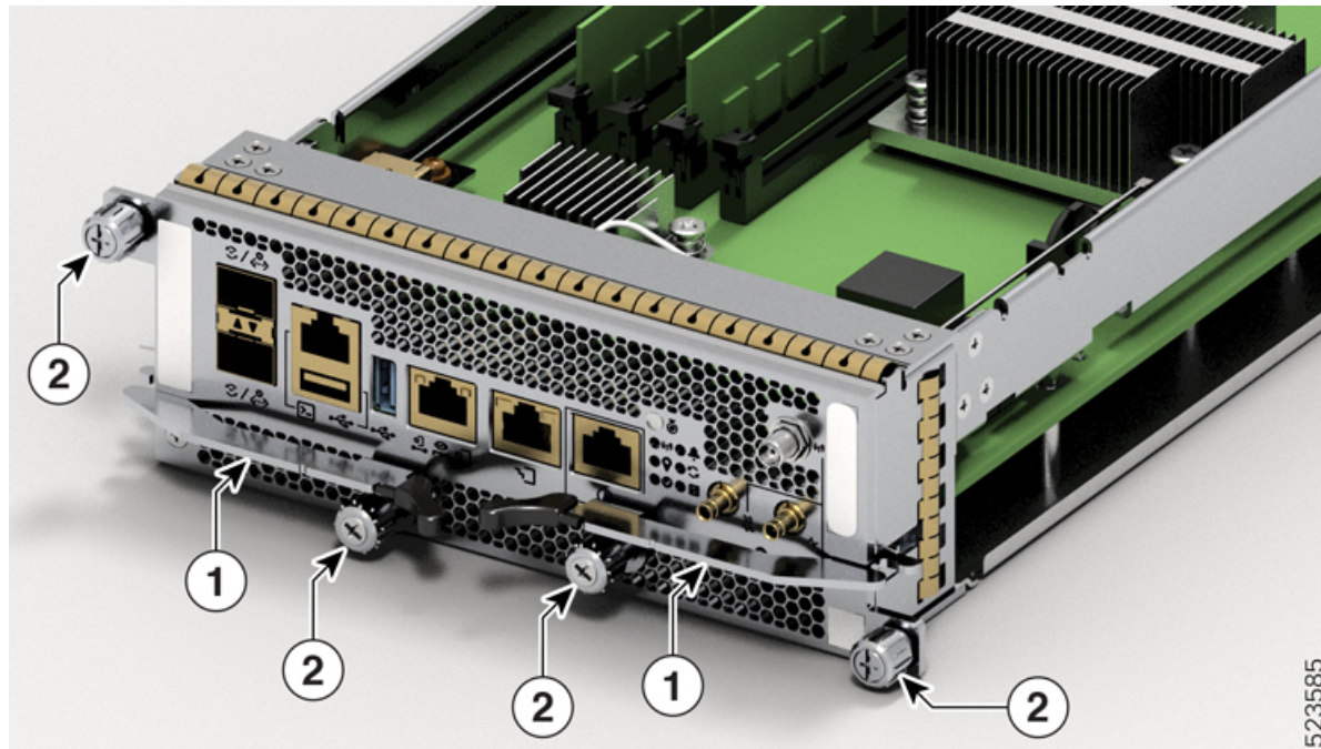
図 114: ルートプロセッサカード (8800-RP2) のコンポーネント
