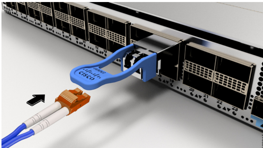
図 107: トランシーバモジュールのケーブル配線
