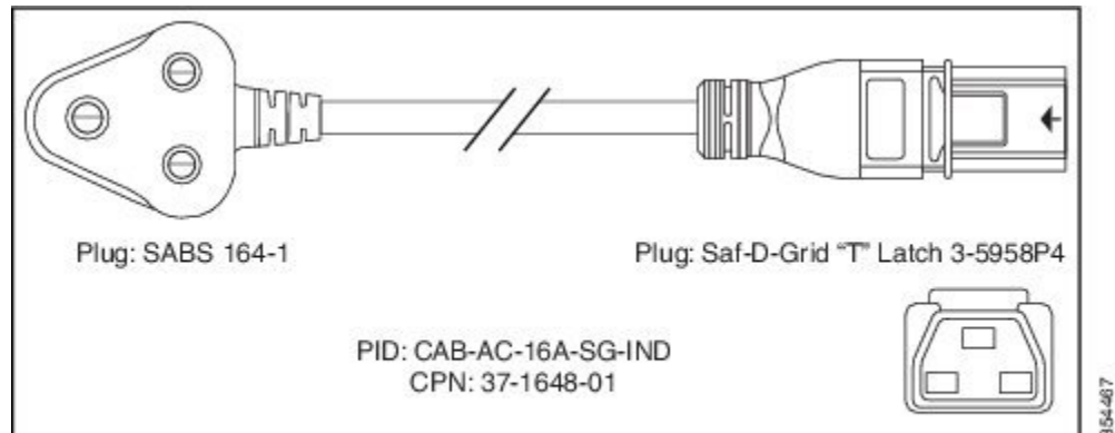
図 80: CAB-AC-16A-SG-IND 電源コード
