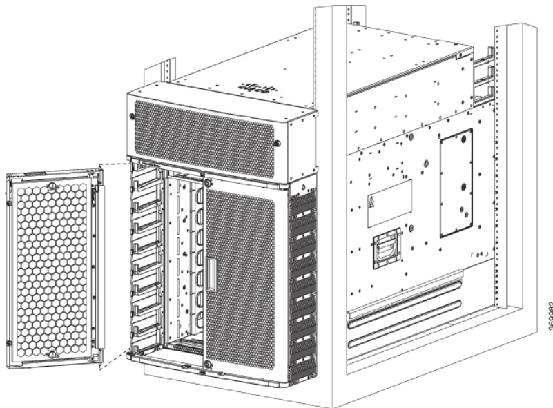
図 51: 8808 シャーシへの前面扉の取り付け
