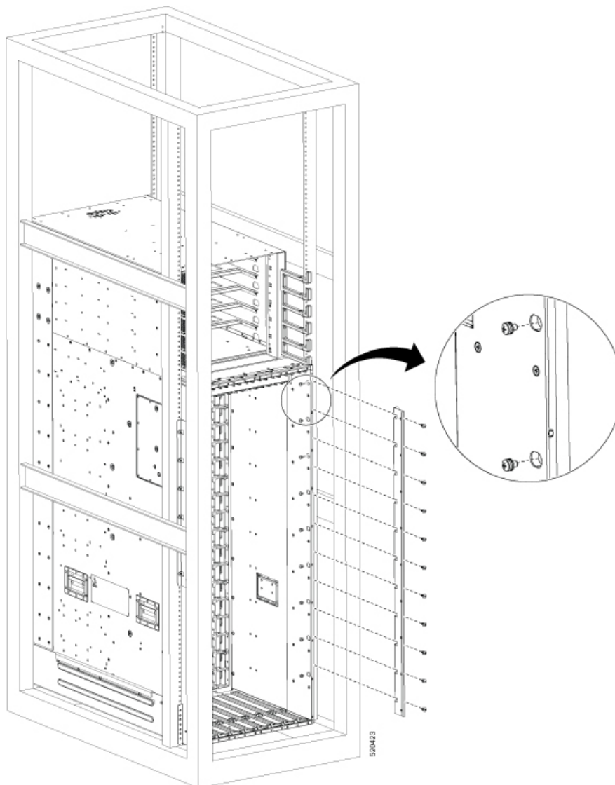
図 22: ラックへの 8818 シャーシの取り付け (右左背面図)
