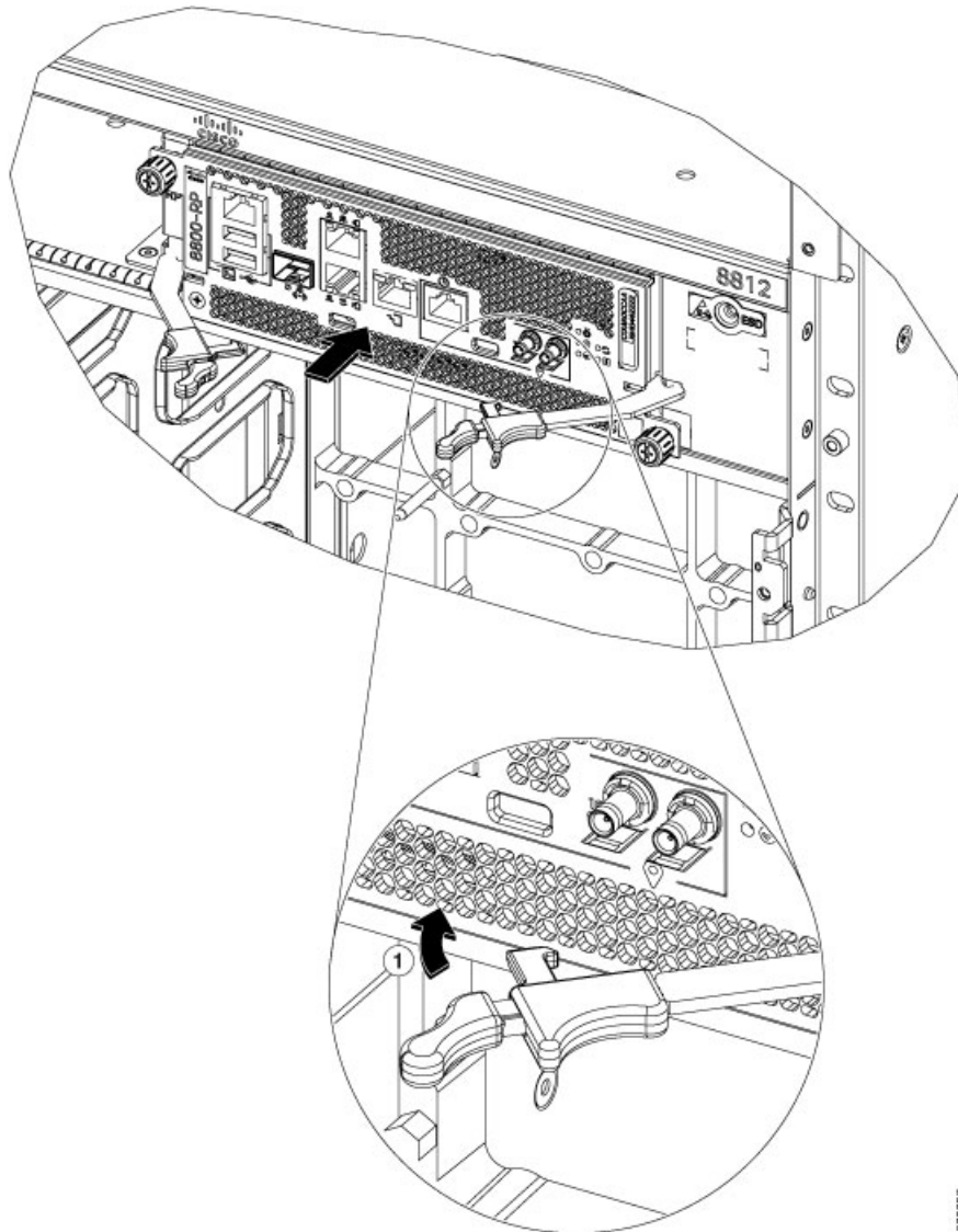
図 113: シャーシへのルートプロセッサカードの取り付け
