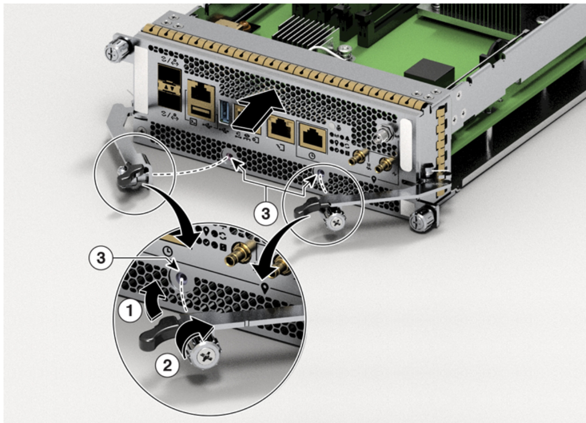
図 117: シャーシへのルートプロセッサカード (8800-RP2) の取り付け
