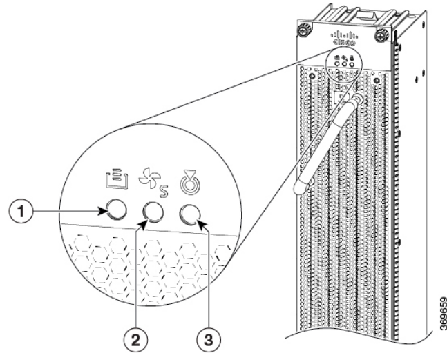
図 151: ファントレイの LED
