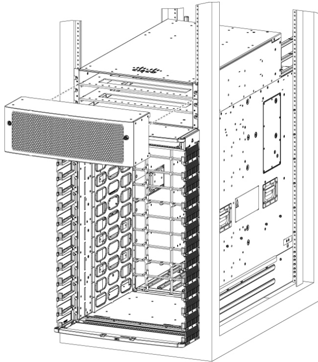
図 142: 8808 シャーシの電源ベゼル
