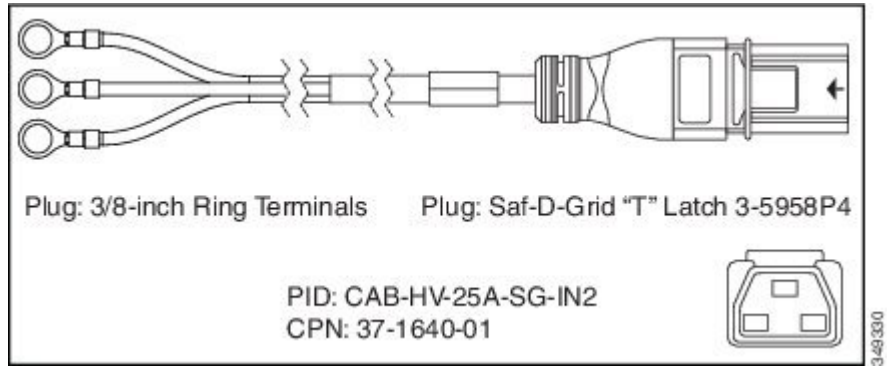
図 96: CAB-HV-25A-SG-IN3 電源コード
