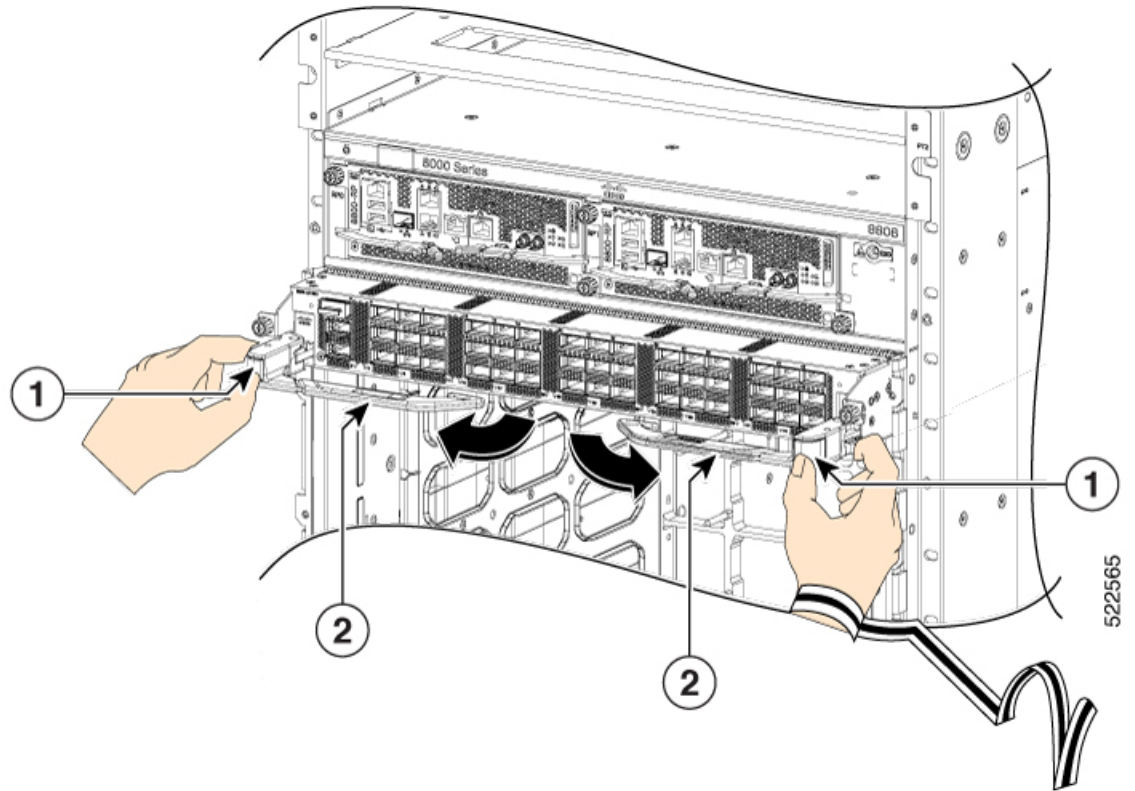
図 123: イジェクトボタンを押す
