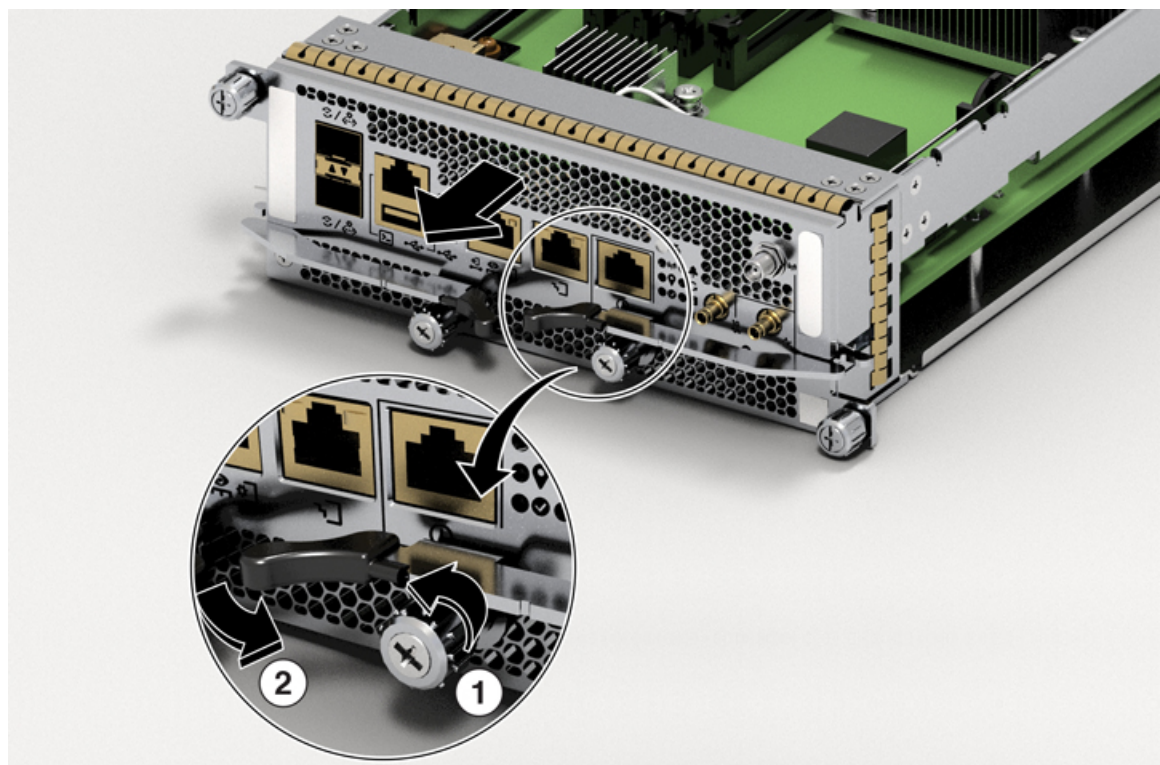
図 115: シャーシからのルートプロセッサカード (8800-RP2) の取り外し
