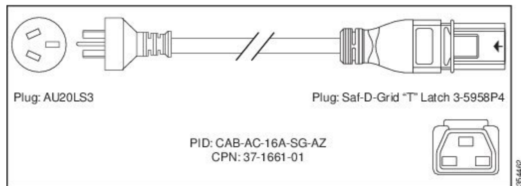
図 76: CAB-AC-16A-SG-AZ 電源コード
