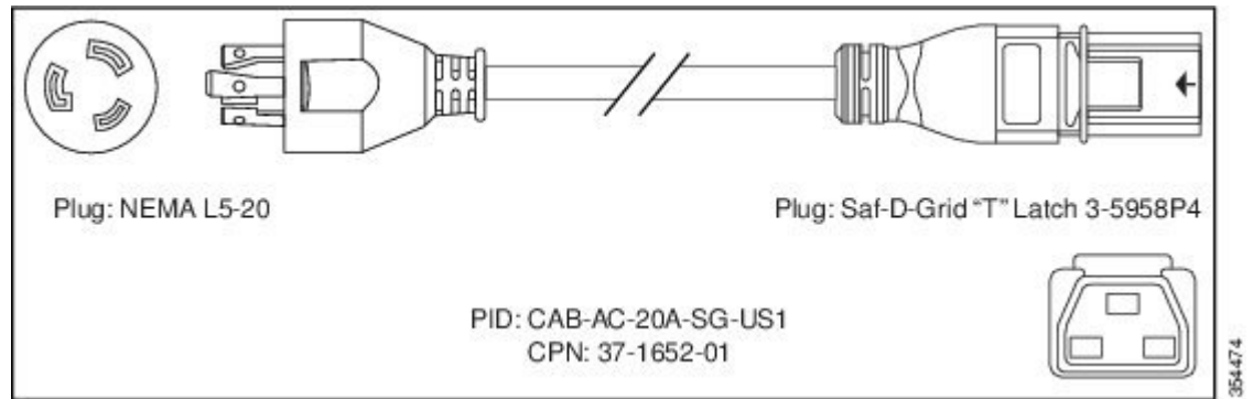
図 90: CAB-AC-20A-SG-US2 電源コード
