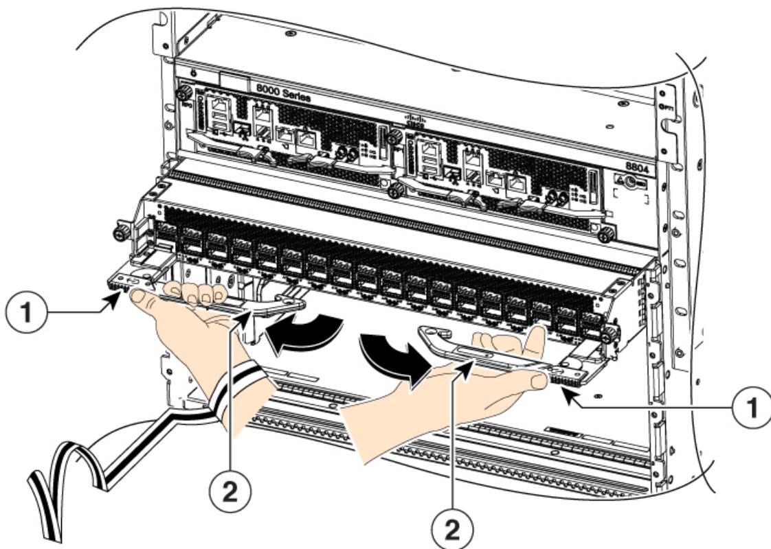
図 129: エジェクトレバーのロック解除
