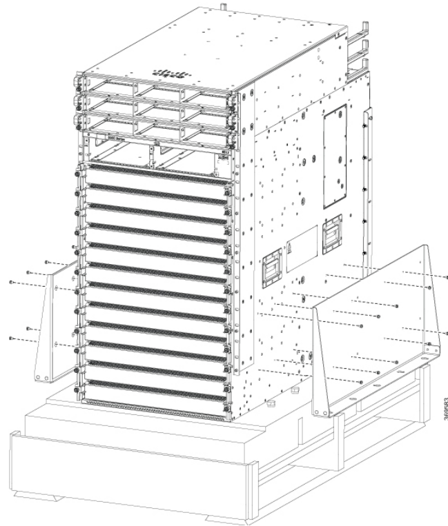
図 11: 8812 シャーシからの輸送用ブラケットの取り外し
