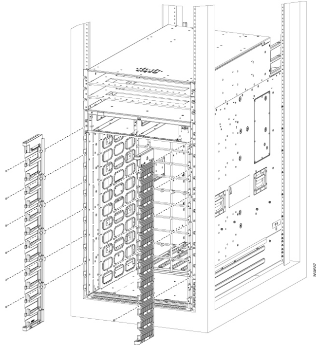
図 36: 8808 シャーシのケーブル管理ブラケット
