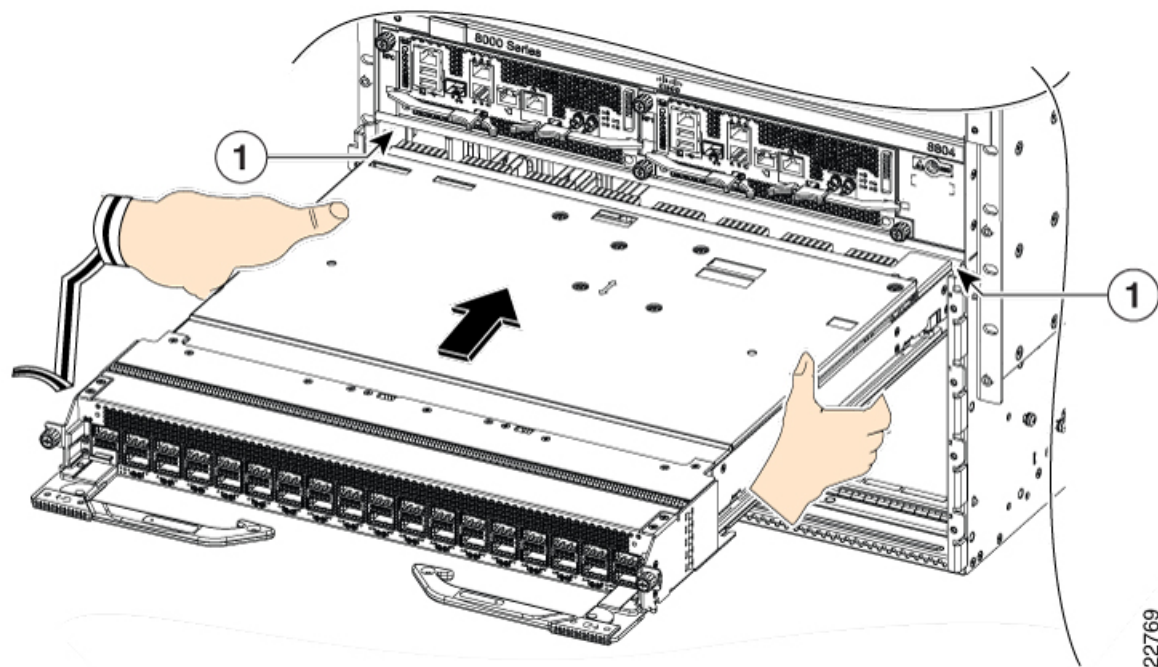
図 128: シャーシへのラインカードの挿入
