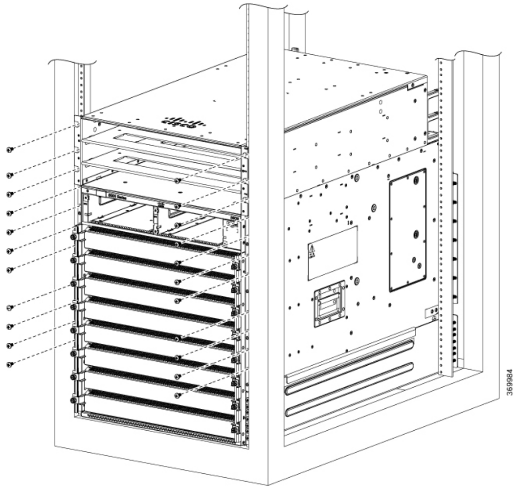
図 19: ラックへの 8808 シャーシの取り付け (前面)
