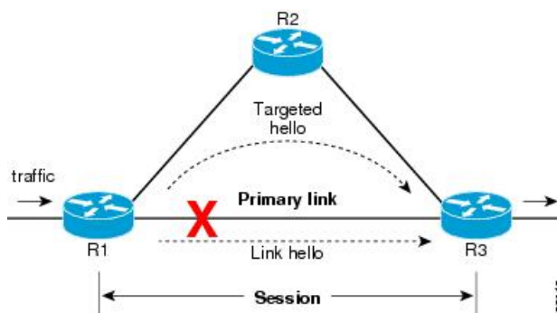
Figure 5: セッション保護
