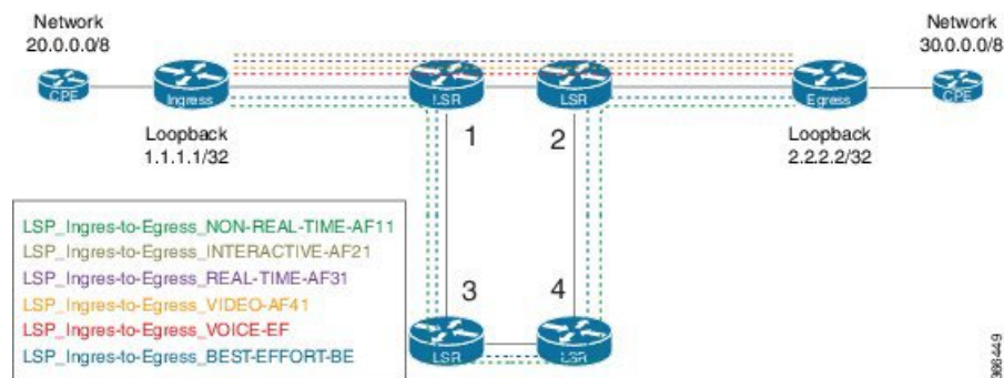
図 12: ポリシーベース トンネル選択の実装
