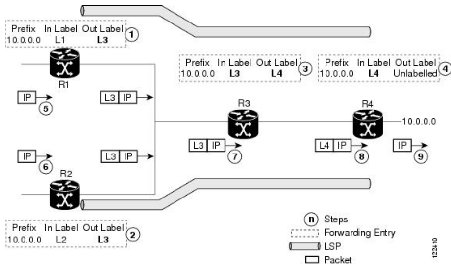
Figure 2: MPLS 転送
