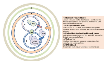
図 16: 複数レイヤで保護された境界アーキテクチャ：強化された外部シェルを備えた仮想アプライアンスシステム
