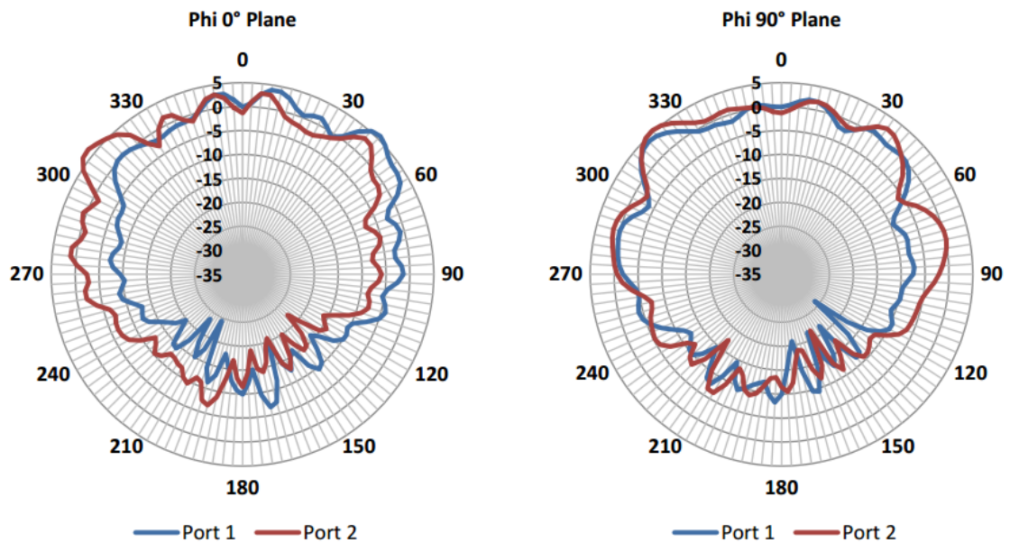
図 8: 5.55 GHz アンテナ放射パターン - 垂直面
