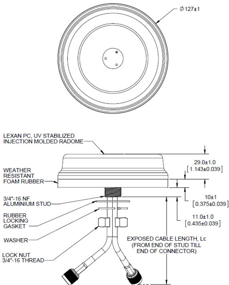
図 2: ANT-2-WLAN-D-0 の機械的詳細
