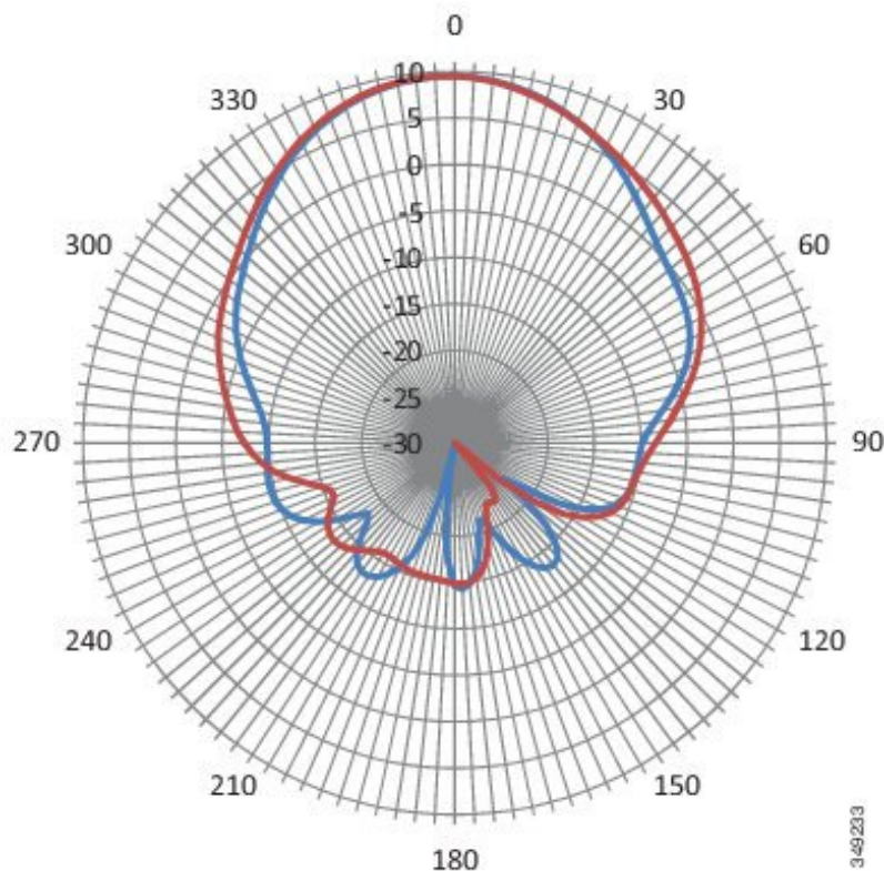
図 15: 2700 MHz アンテナ放射パターン - 垂直面
