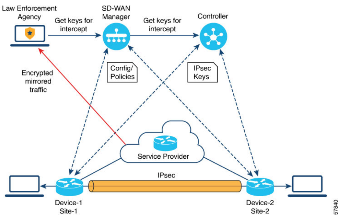
図 21:合法的傍受 2.0 アーキテクチャ
