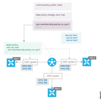
図 10: VPN メンバーシップトポロジ
