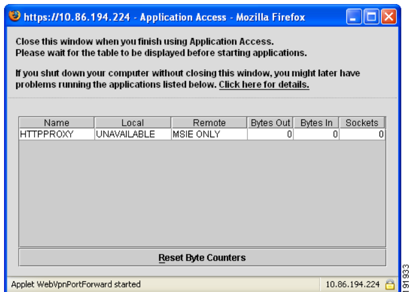
図 11-9 クライアントレス SSL VPN の [Application Access] ウィンドウ
