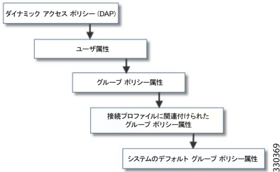
図 14-1 ポリシー実施フロー
