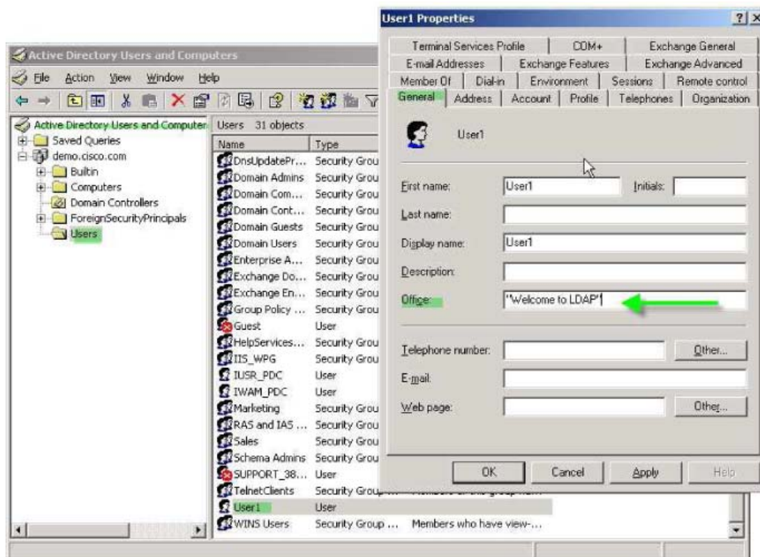
図 14-3 LDAP ユーザの設定
