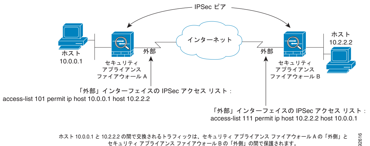
図 1-4 暗号 ACL を IPsec に適用する方法
