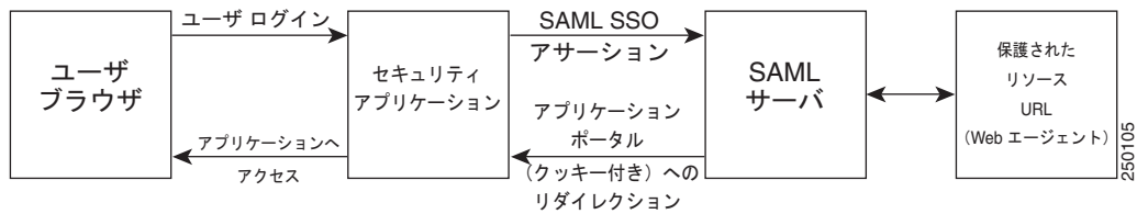
図 11-3 SAML の通信フロー
