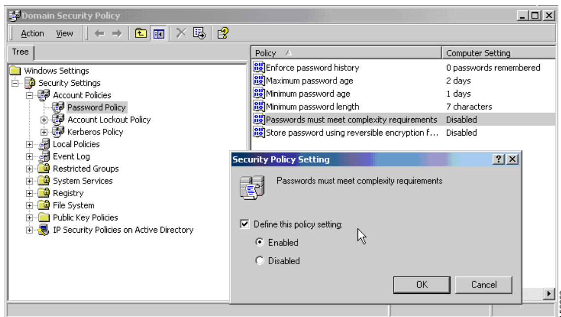
図 4-6 Active Directory : パスワードの複雑性の強制
