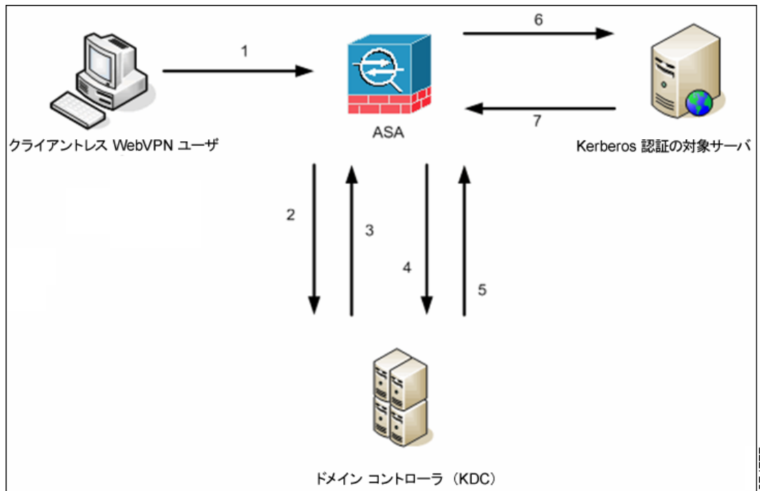
図 11-7 KCD プロセス
