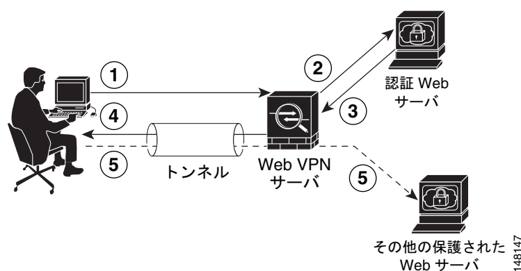
図 11-4 HTTP Form を使用した SSO 認証
