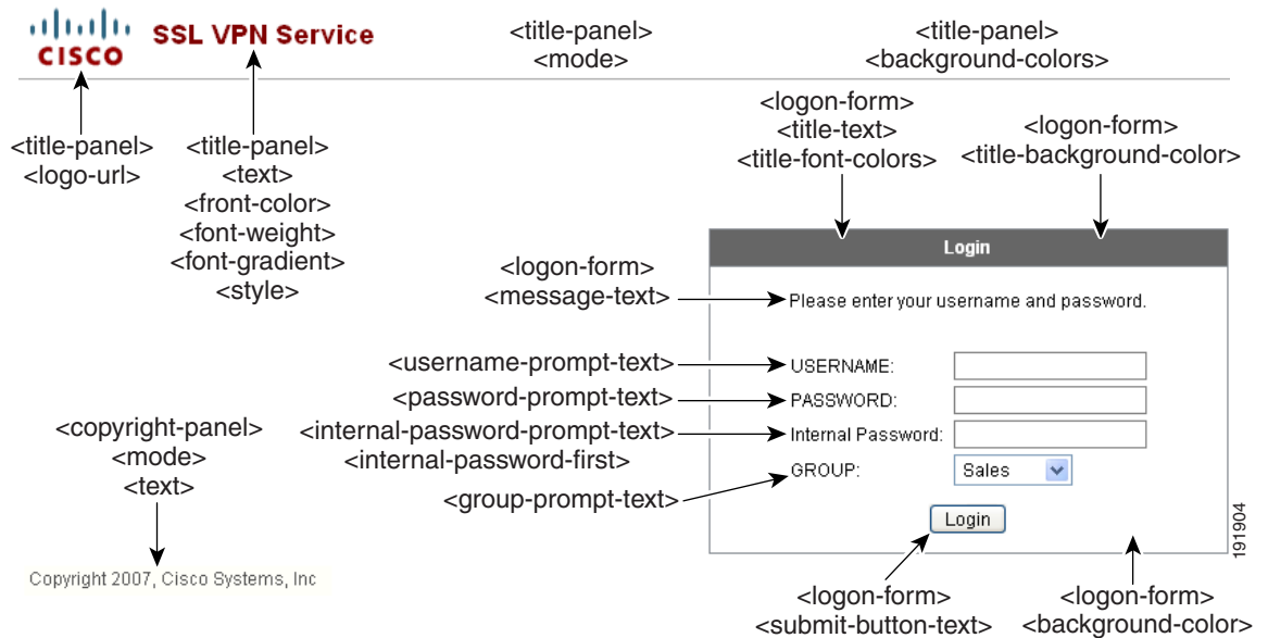
図 11-11 [Login] ページと関連の XML タグ
