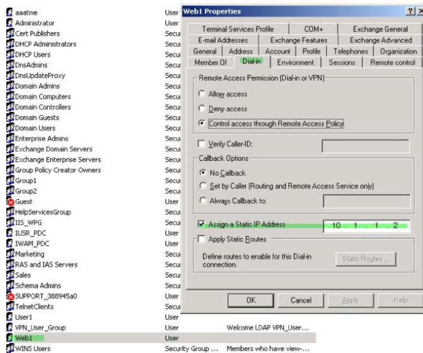
図 14-6 スタティック IP アドレスの割り当て
