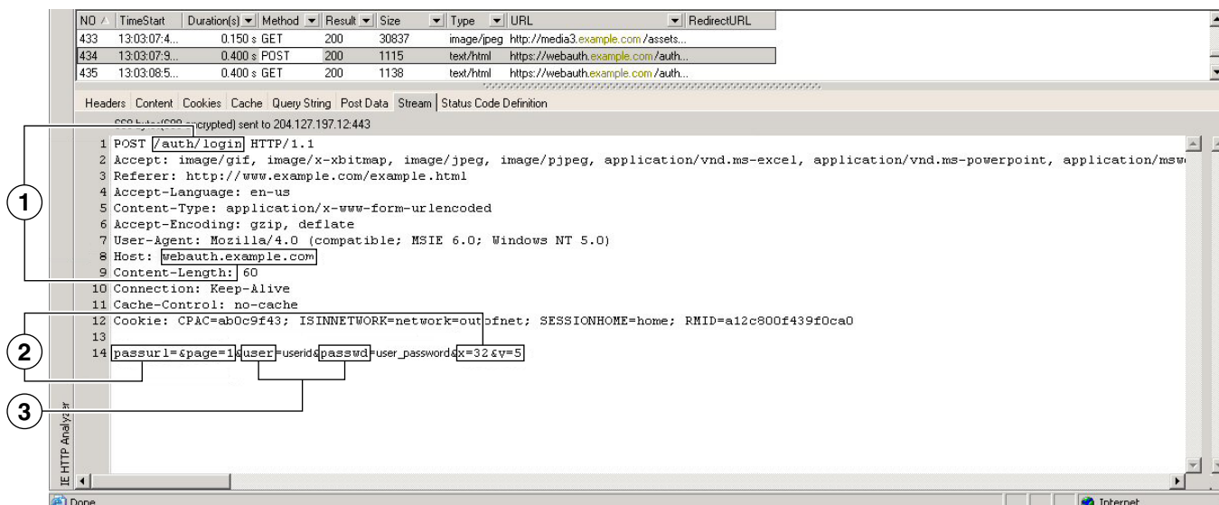
図 11-5 action-uri、非表示、ユーザ名、パスワードの各種パラメータ
