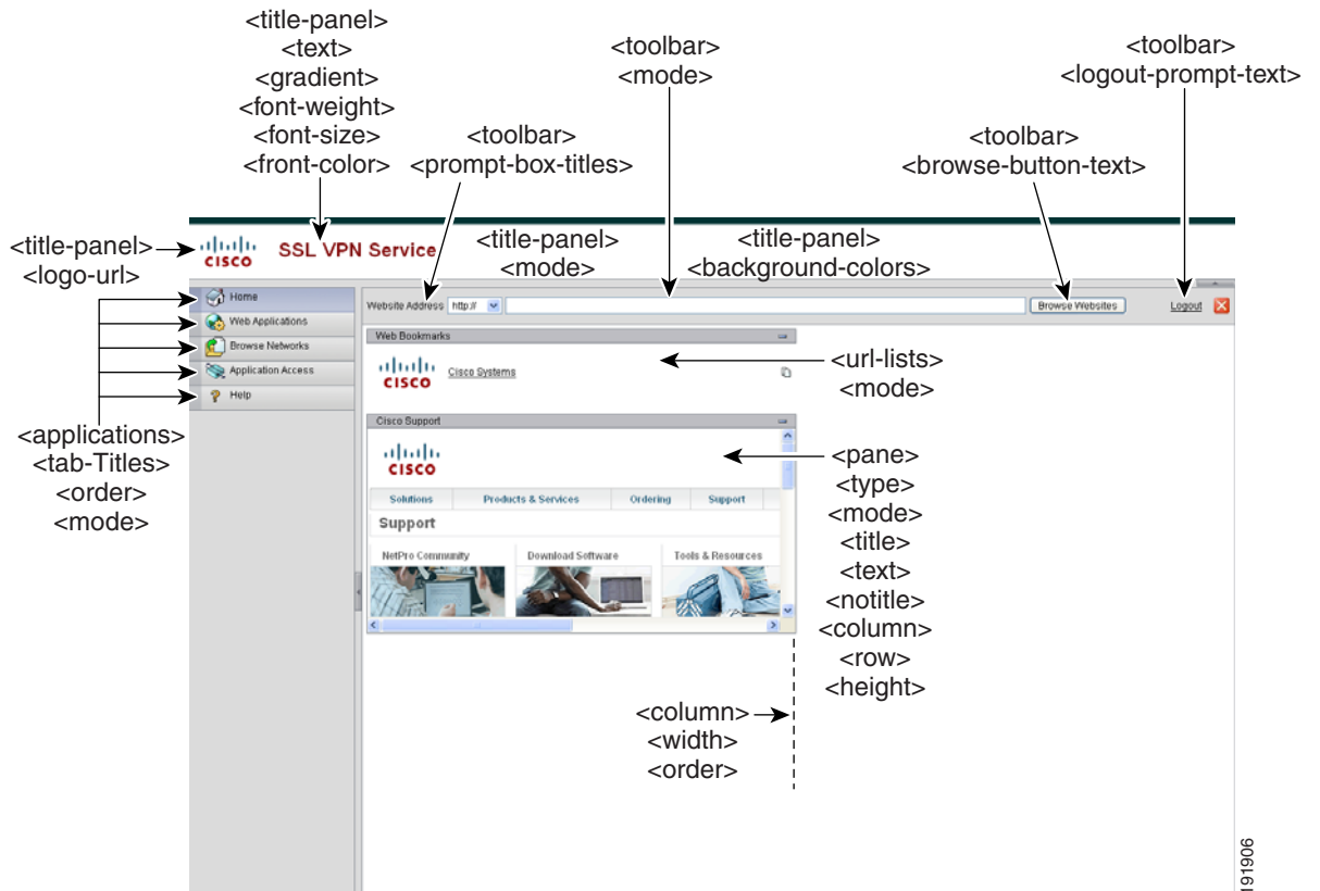
図 11-14 ポータル ページと関連の XML タグ
