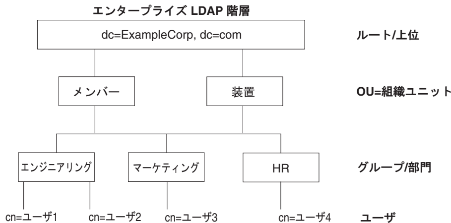
図 14-2 マルチレベルの LDAP 階層
