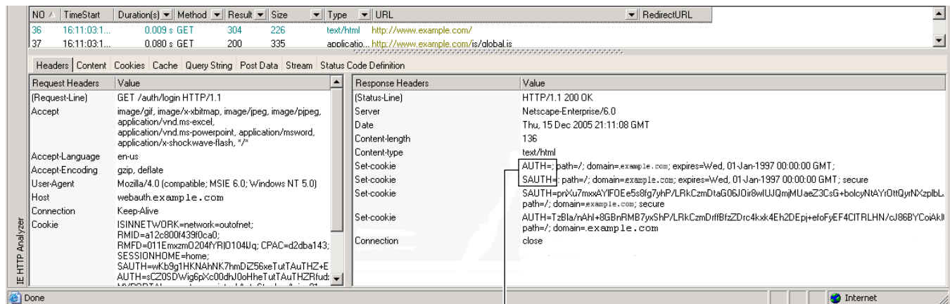
図 11-6 HTTP アナライザの出力例に表示された許可クッキー
