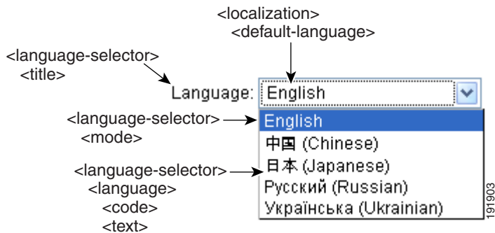
図 11-12 [Login] 画面上的言語セクタと関連の XML タグ
