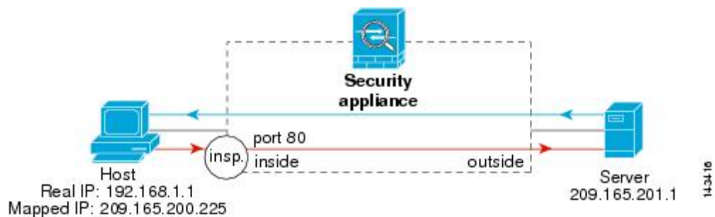
図 50: NATによるHTTPインスペクション
