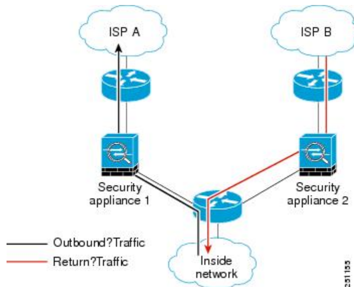
図 50: 非対称ルーティング
