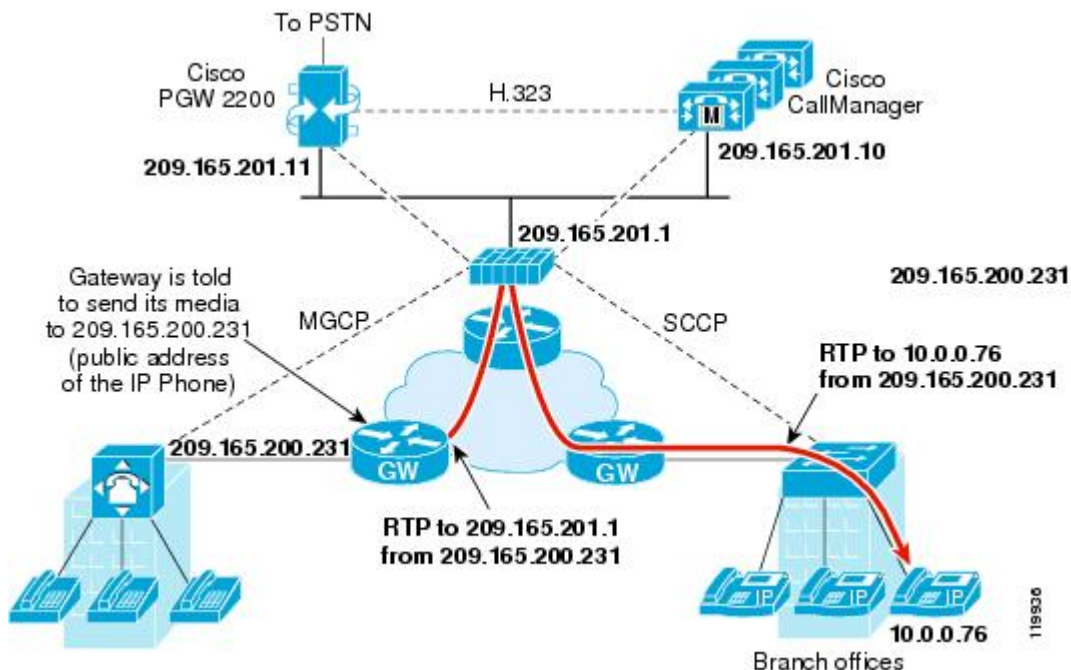
図 47: NAT と MGCP の使用
