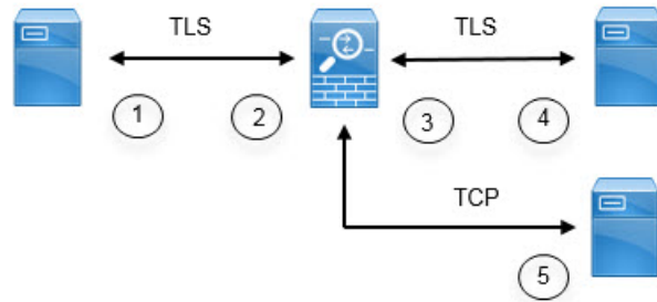
図 49: Diameter TLS インспекション
