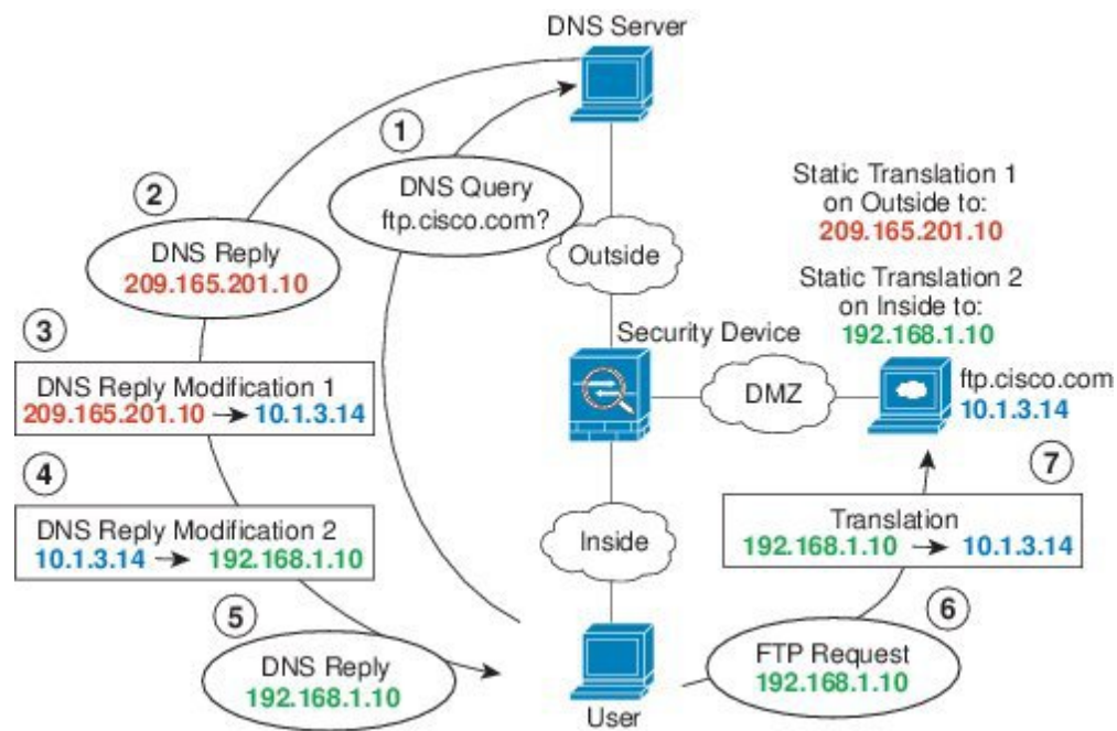
図 45: DNS 応答修正：別々のネットワーク上の DNS サーバ、ホスト、およびサーバ
