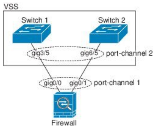
図 63: VSS/vPC への接続
