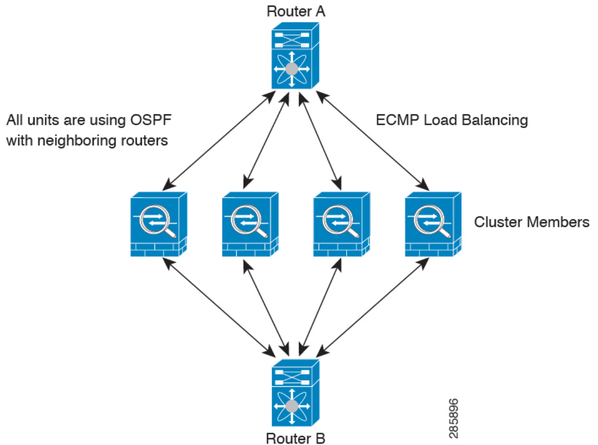
図 61: 個別インターフェイスモードでのダイナミックルーティング
