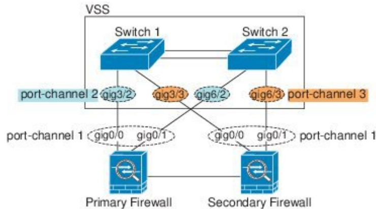
図 64: アクティブ/スタンバイ フェールオーバーと VSS/vPC
