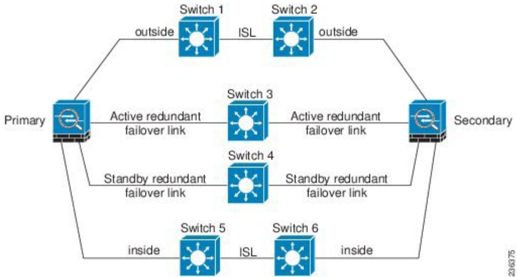
図 52: Inter-Switch Link (ISL) を使用した接続
