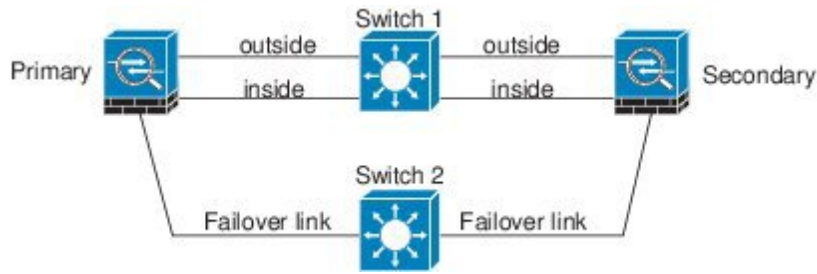
図 49:ケーブルを使用した接続
