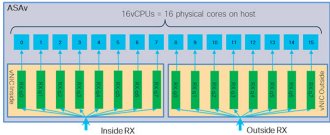
図 10: 16 コア ASA の RSS RX キュー
