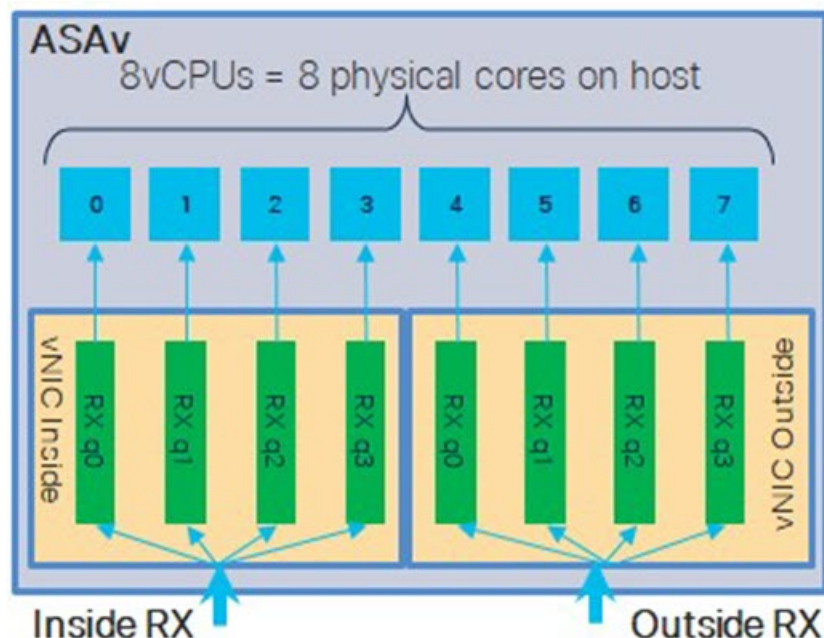
図 5: 8 コア ASA RSS RX キュー
