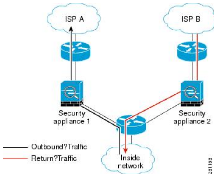
図 47: 非対称ルーティング
