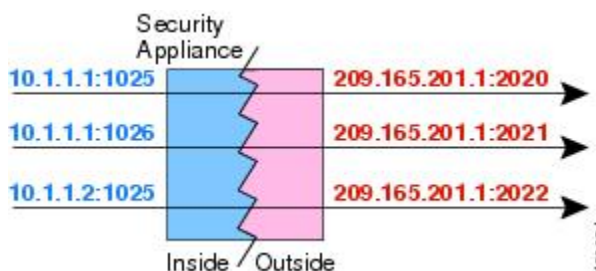
図 19: ダイナミック PAT
