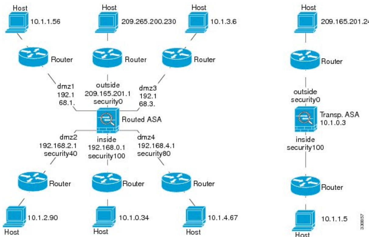
図 78: インターフェイス、ルータ、およびホストを含むネットワーク図
