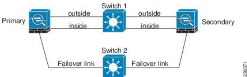
図 48: 異なるスイッチを使用した接続
