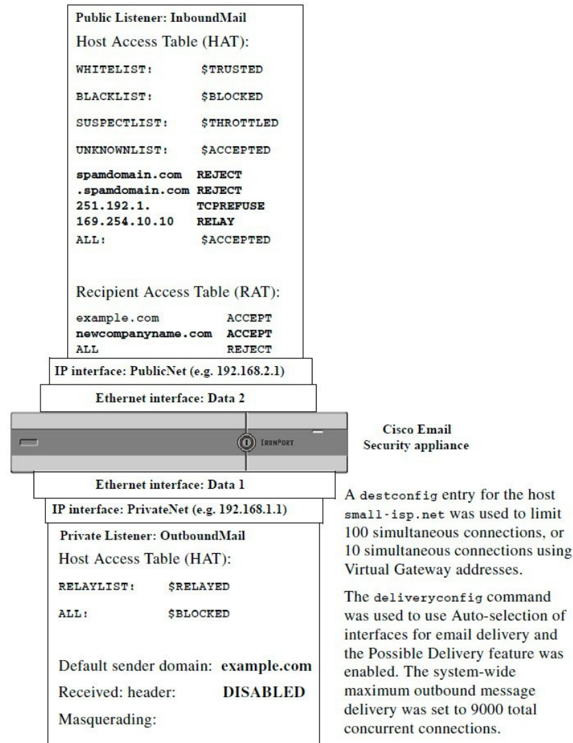
Figure 51: 宛先および配信パラメータの設定
