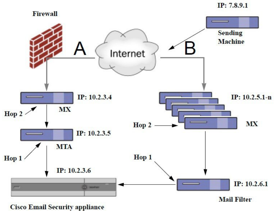
Figure 26: MX/MTAによるメールリレー：拡張
