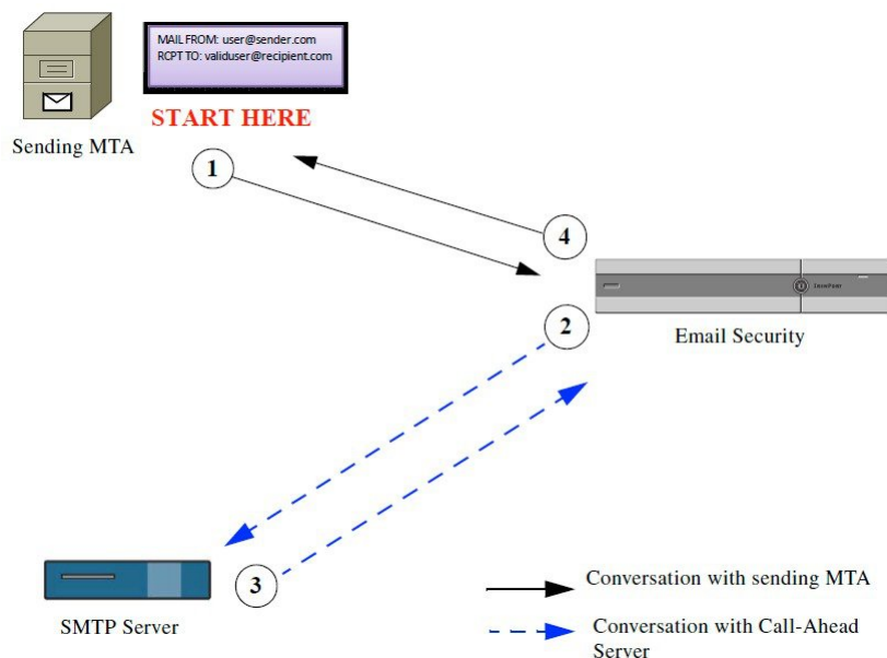
Figure 43: SMTP コール Ahead サーバ通信のワークフロー
