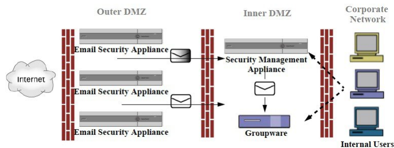
Figure 88: シスコのコンテンツセキュリティ管理アプライアンスによる一般的なネットワーク設定
