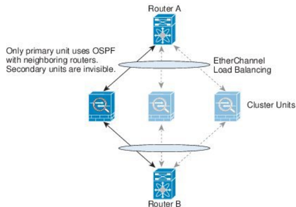
図 15: ダイナミック ルーティング
