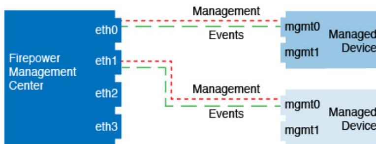
図 19: Firepower Management Center 上の複数の管理インターフェイスを使用する場合
