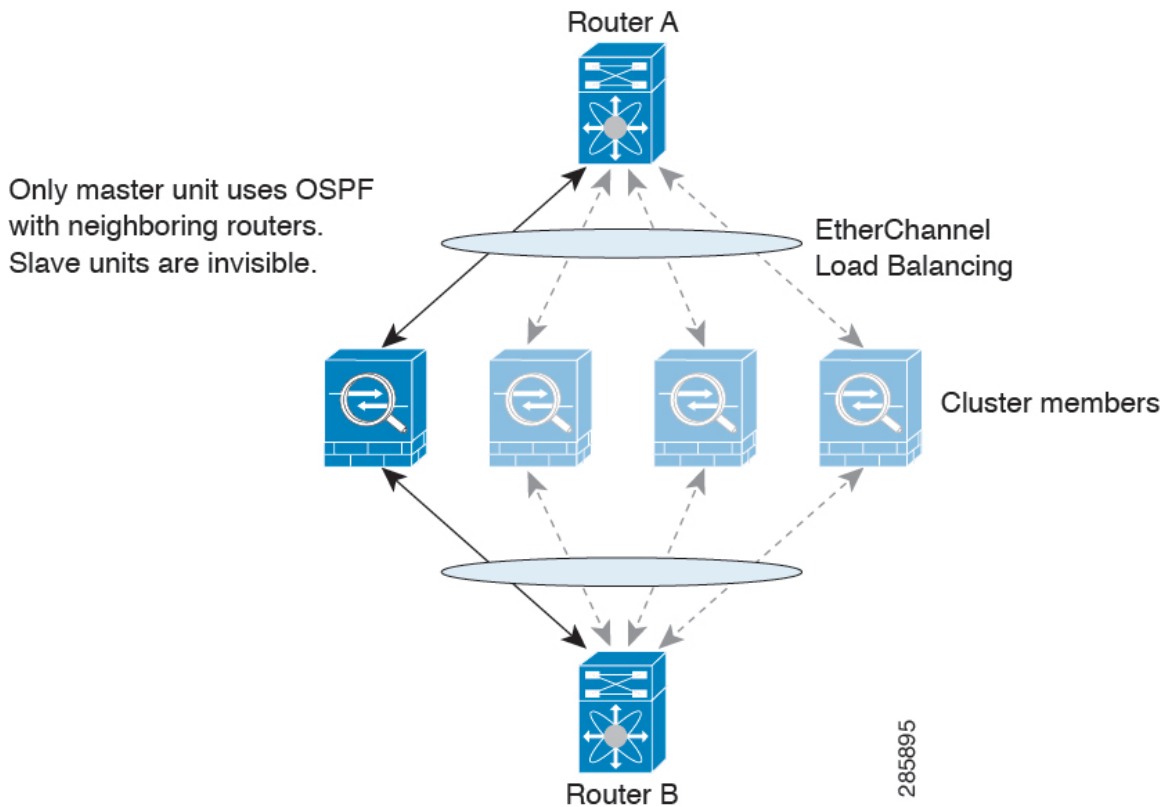
図 17: クラスタリングでのダイナミック ルーティング
