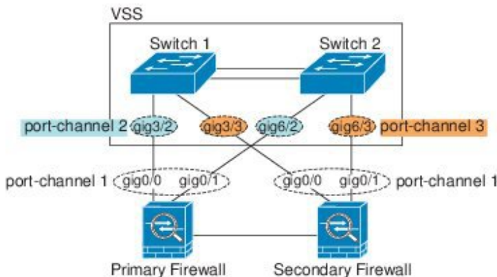
図 7: アクティブ/スタンバイ フェールオーバーと VSS/vPC
