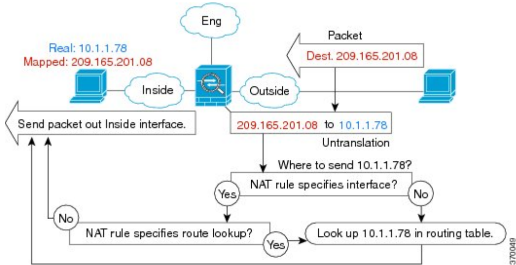
図 16: NATによるルーテッドモードでの出インターフェイスの選択
