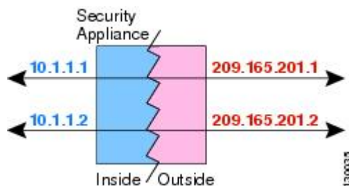
図 28:スタティック NAT
