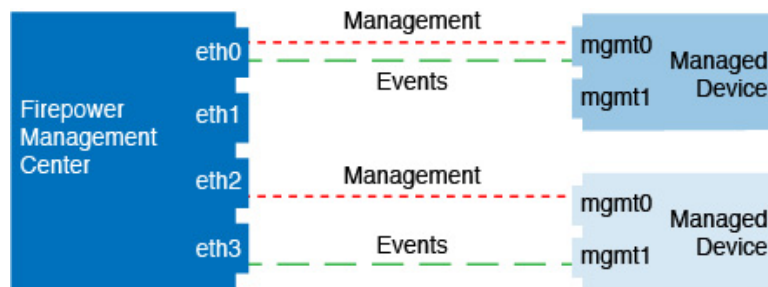
図 21: 管理インターフェイスとイベントインターフェイスを混在させて使用する場合
