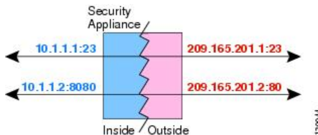
図 29:ポート変換を設定したスタティック NAT の一般的なシナリオ
