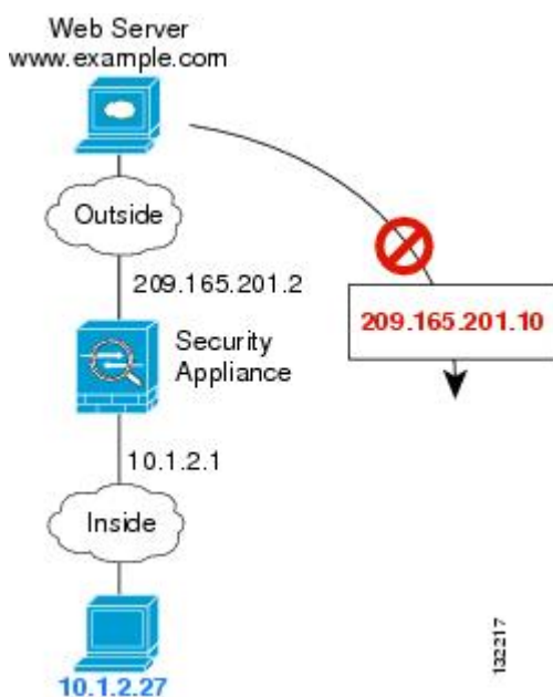
図 26: マッピングアドレスへの接続開始を試みているリモートホスト
