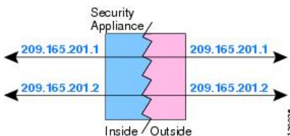
図 34: アイデンティティ NAT
