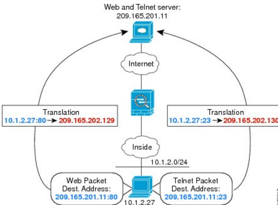
図 40:異なる宛先ポートを使用する手動 NAT
