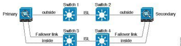
図 12: セキュアスイッチを使用した接続
