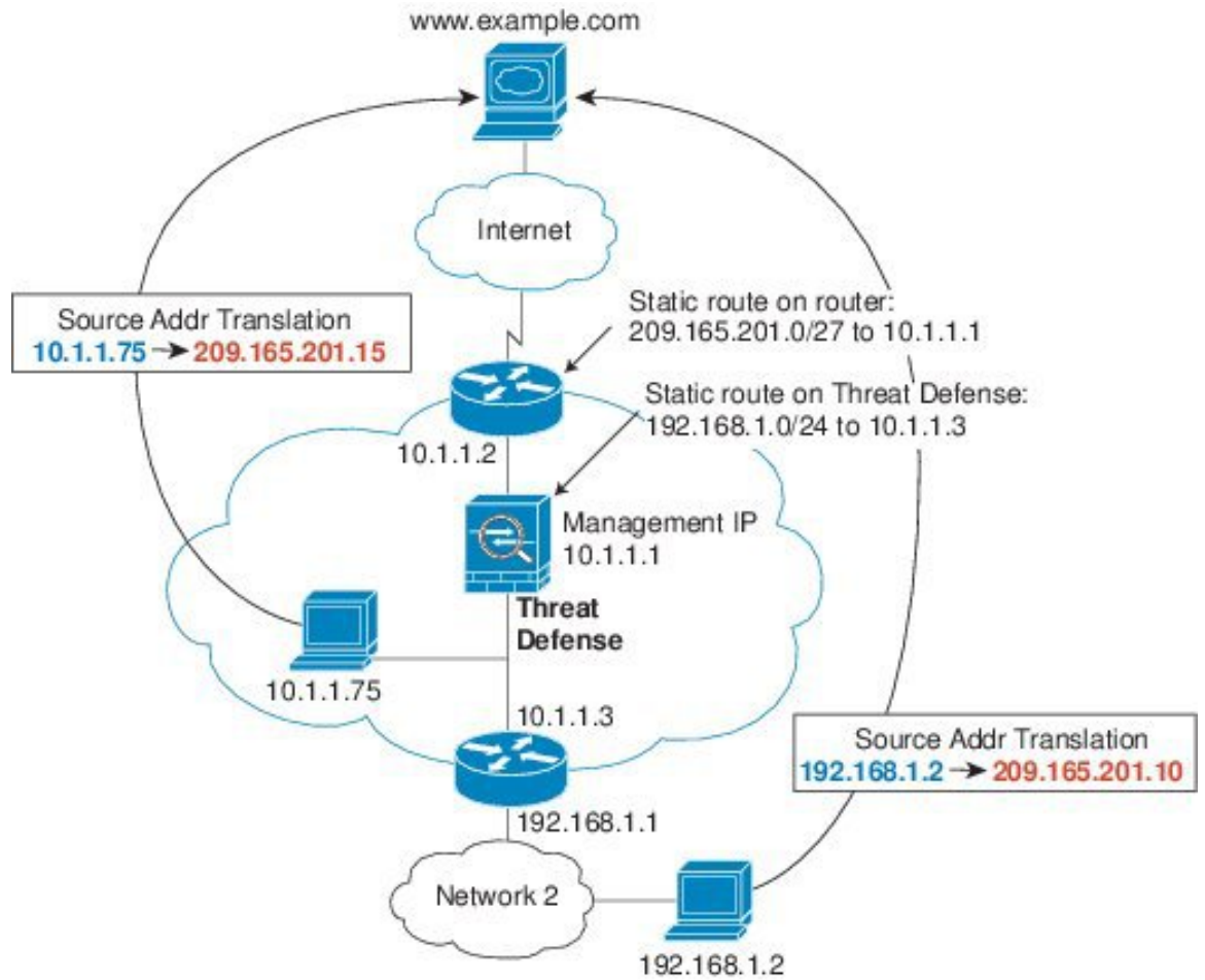
図 5: NAT の例 : ブリッジグループ内の NAT
