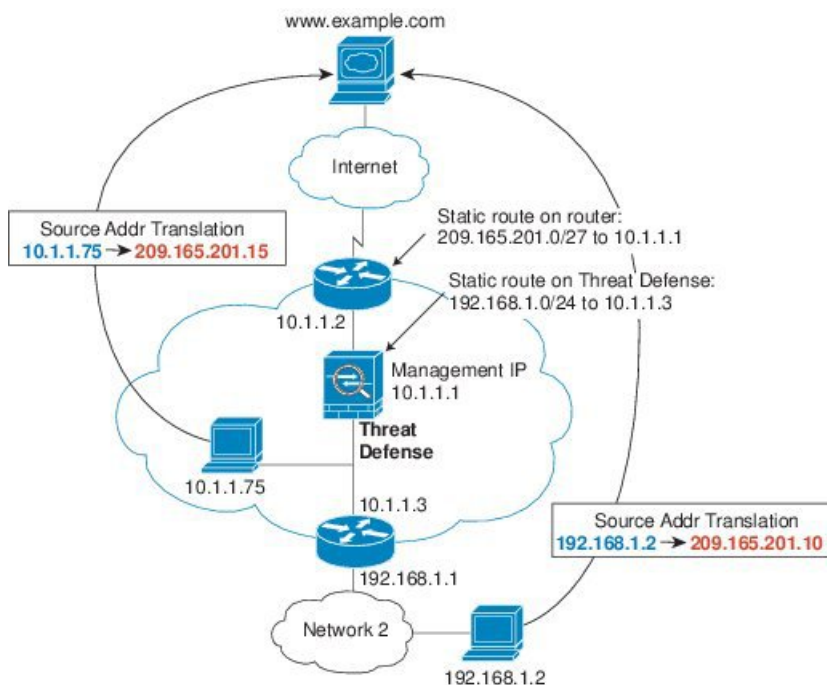
図 23: NAT の例 : トランスパレントモード
