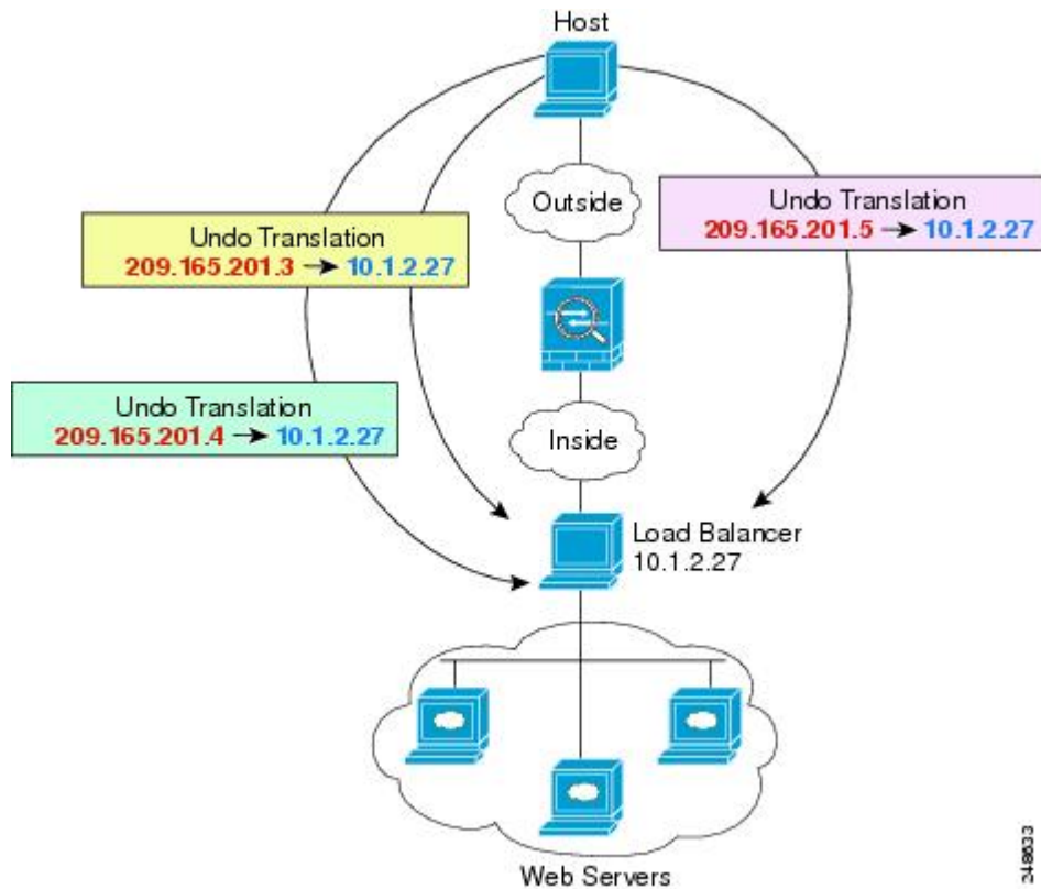
図 31: 一対多のスタティック NAT の例
