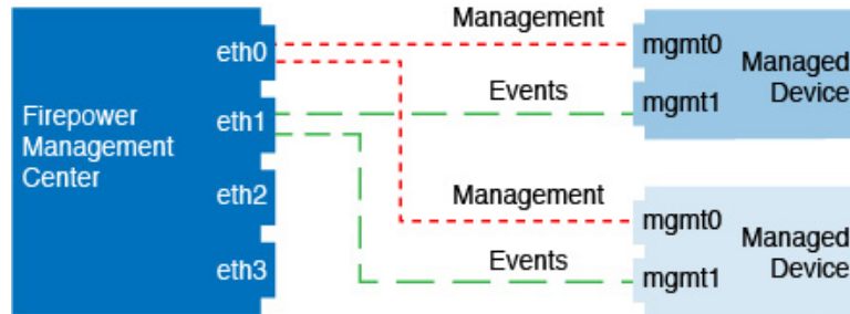
図 20: Firepower Management Center 上の個別のイベントインターフェイスと管理対象デバイスを使用する場合
