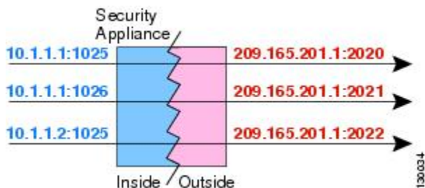
図 27: ダイナミック PAT
