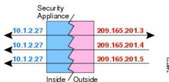
図 30: 一対多のスタティック NAT
