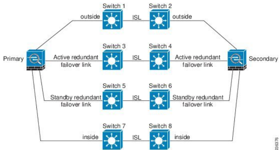
図 14: Inter-Switch Link (ISL) を使用した接続
