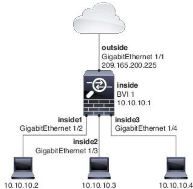
図 4: 内部ブリッジグループと外部ルーテッドインターフェイスを持つルーテッドファイアウォールネットワーク
