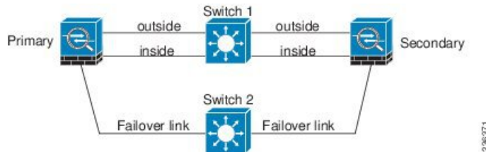
図 11: ケーブルを使用した接続
