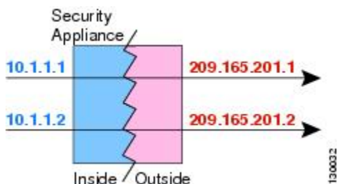
図 25: ダイナミック NAT
