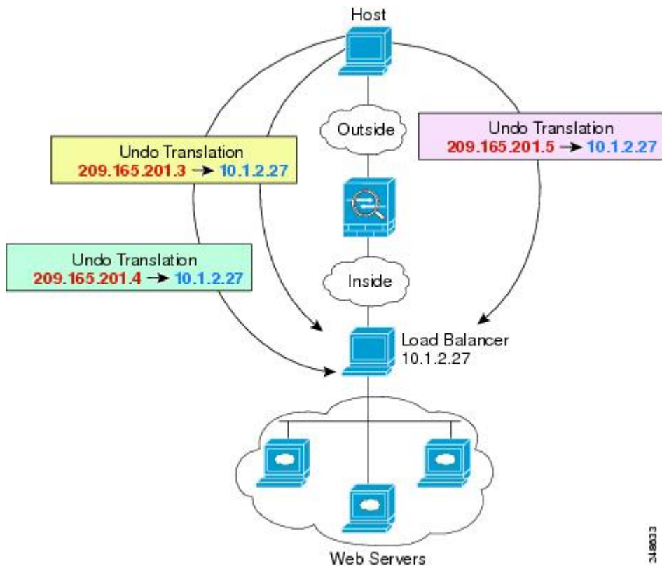
図 37: 内部ロードバランサのスタティック NAT (1 対多)
