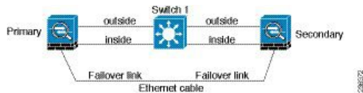
図 11: ケーブルを使用した接続
