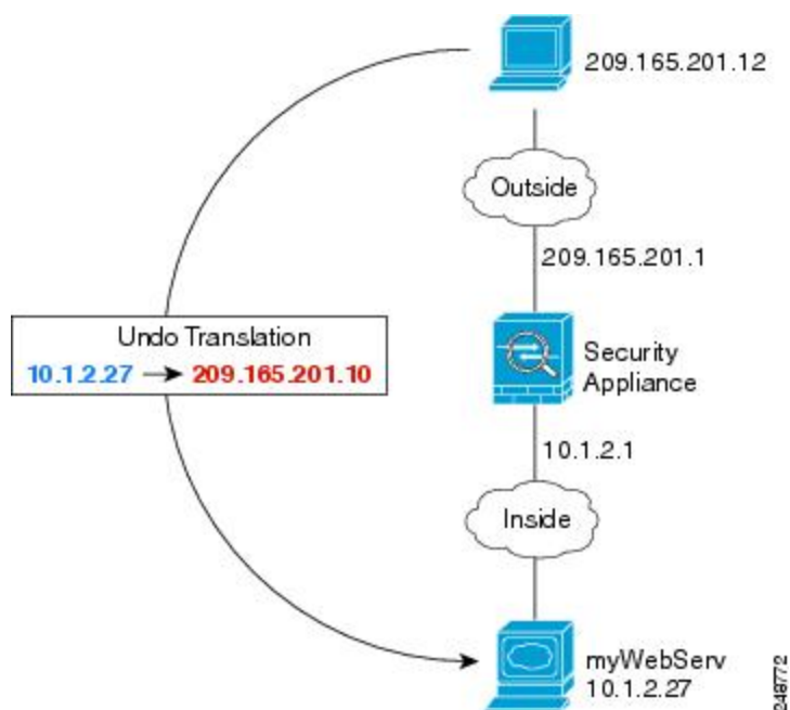
図 35: 内部 Web サーバのスタティック NAT
