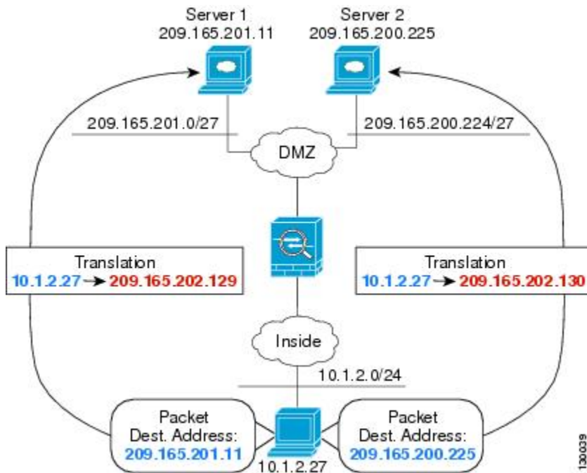
図 39:異なる宛先アドレスを使用する手動 NAT
