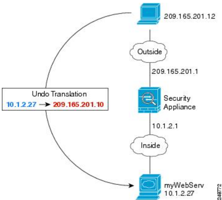
図 24: 内部 Web サーバのスタティック NAT
