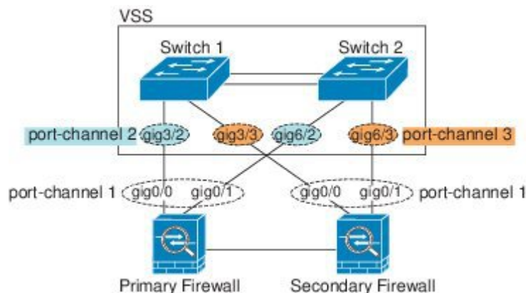
図 11: アクティブ/スタンバイ フェールオーバーと VSS/vPC
