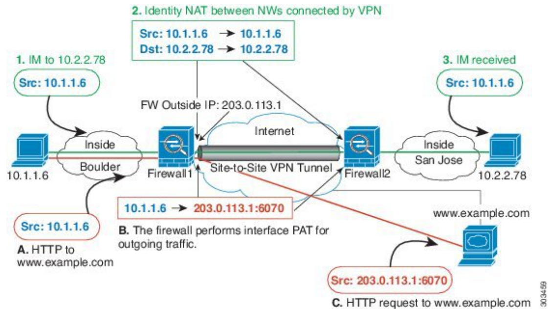
図 28: サイトツーサイトVPNのためのインターフェイスPATおよびアイデンティティNAT
