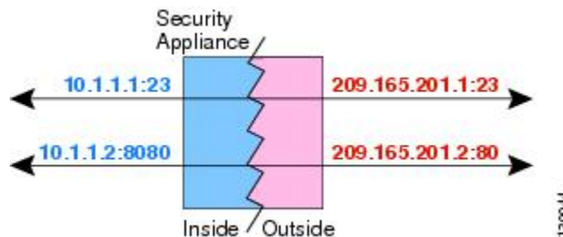
図 18:ポート変換を設定したスタティック NAT の一般的なシナリオ
