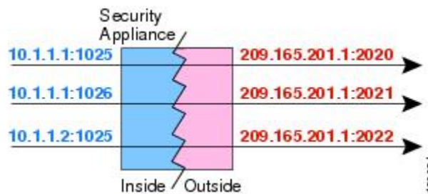
図 16: ダイナミック PAT
