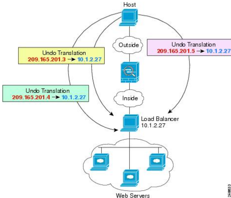
図 20:1 対多のスタティック NAT の例
