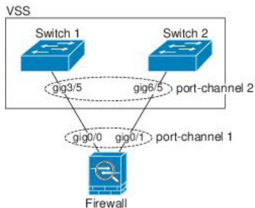
図 10: VSS/vPC への接続
