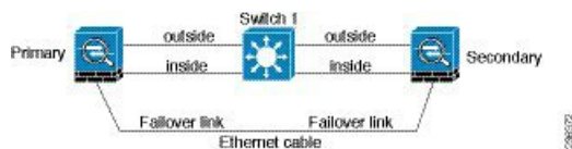
図 8: ケーブルを使用した接続
