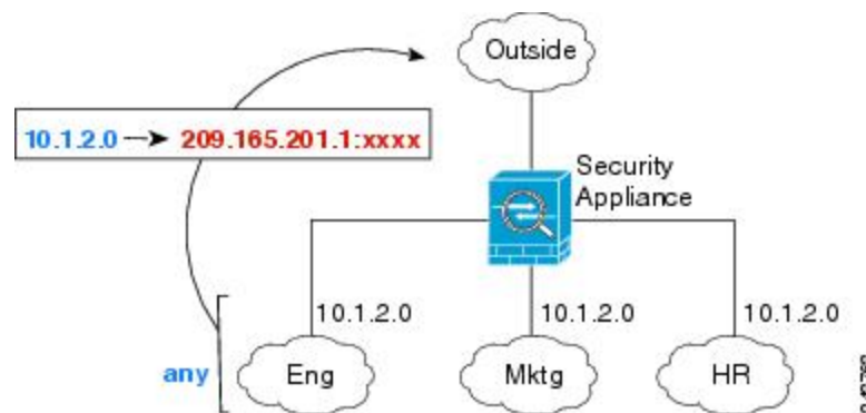
図 13: 任意のインターフェイスの指定
