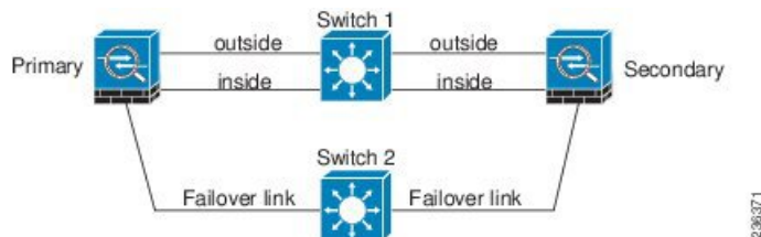
図 8: ケーブルを使用した接続
