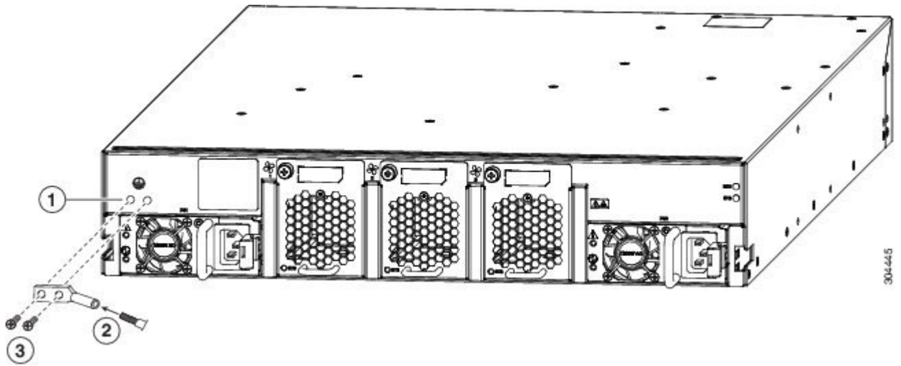
図 12: シャーシのアース接続
