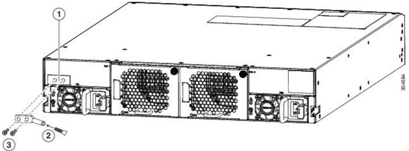
図 11: Cisco Nexus 9396 シャーシのアース接続
