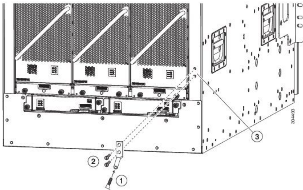
図 12: シャーシのアース接続
