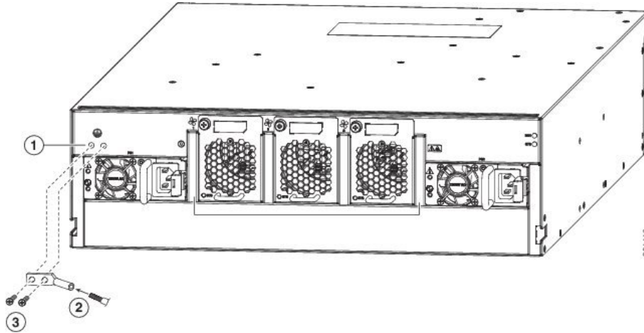
図 10: シャーシのアース接続
