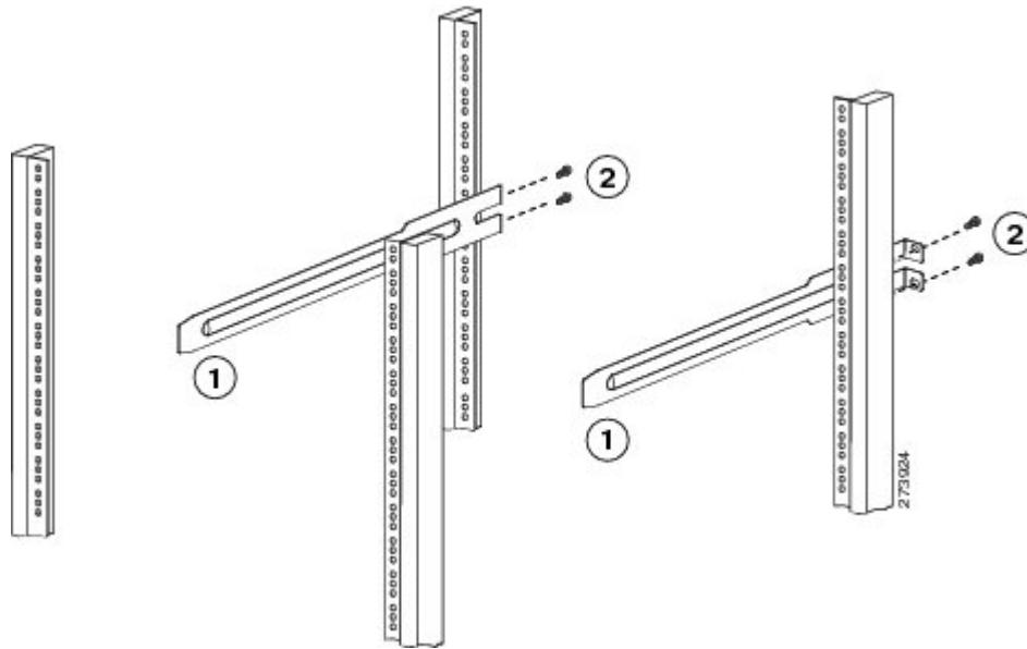
図 8: スライダ レールの取り付け
