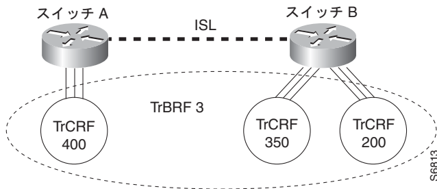
図 12-2 非分散型 TrCRF
