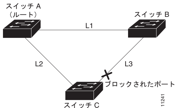
図 18-1 直接リンク障害が発生する前の UplinkFast の例
