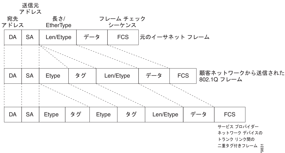
図 15-2 タグなし、802.1Q タグ付き、および、二重タグ付きイーサネット フレーム
