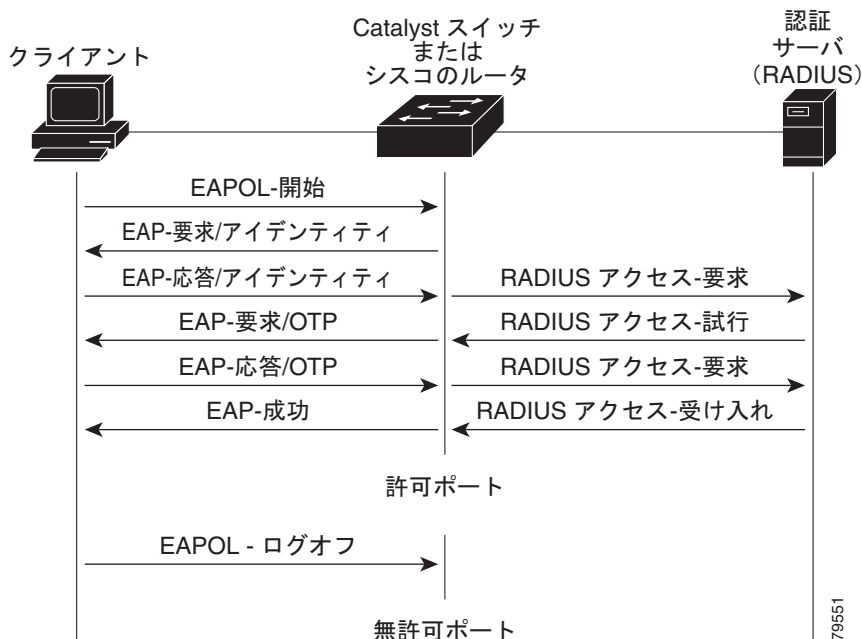
図 42-2 メッセージ交換
