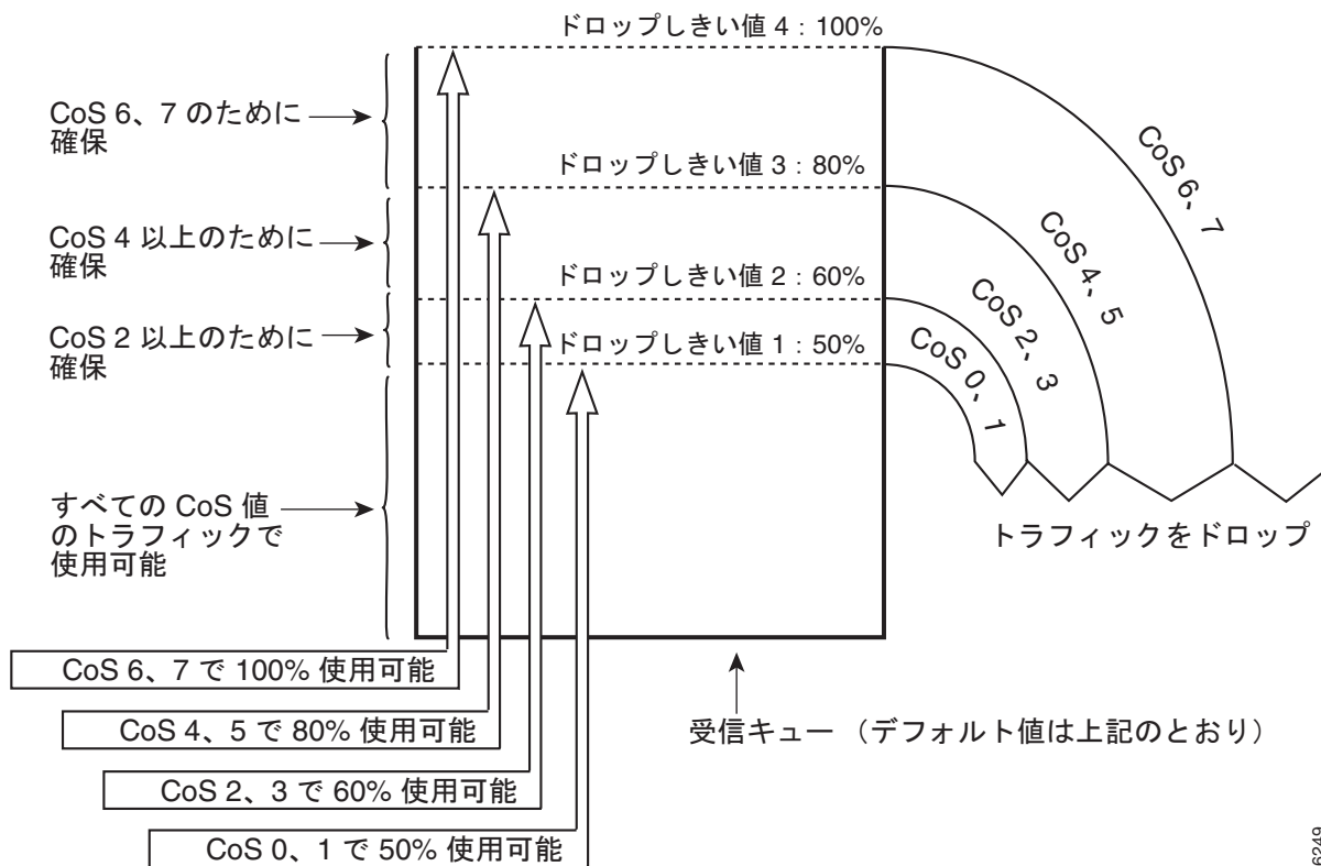
図 38-8 受信キューのドロップしきい値
