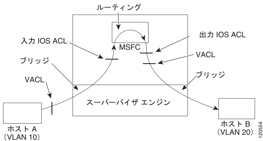
図 32-2 ルーティング対象パケットへの VACL の適用
