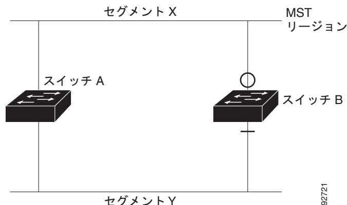
図 17-11 標準準拠および先行標準スイッチの相互運用
