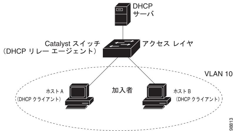
図 34-1 メトロポリタンイーサネットネットワークにおける DHCP リレー エージェント
