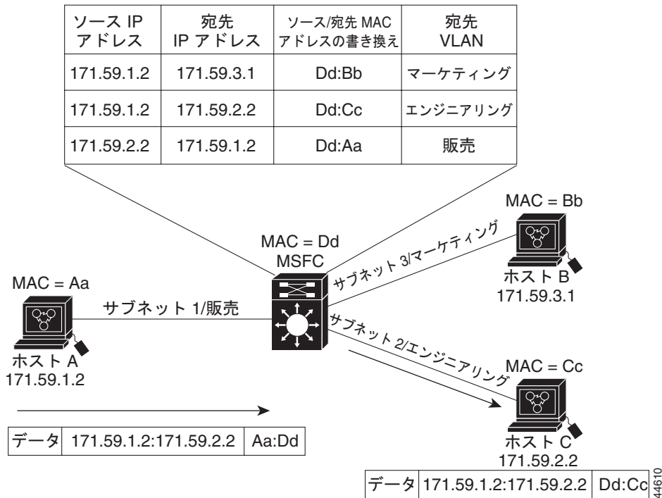
図 23-1 ハードウェア レイヤ 3 スイッチングのトポロジ例
