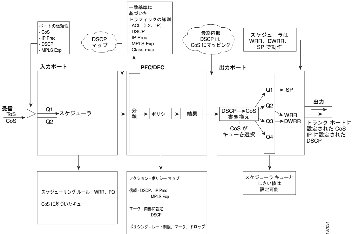
図 38-3 PFC QoS 機能とコンポーネントの概要
