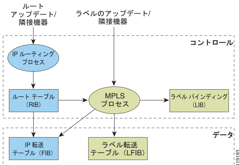
図 21-2 MPLS 転送、制御、データ プレーン
