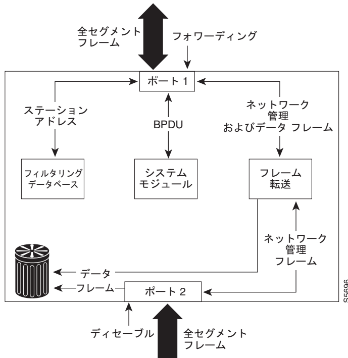
図 17-7 ディセーブル ステートのインターフェイス 2
