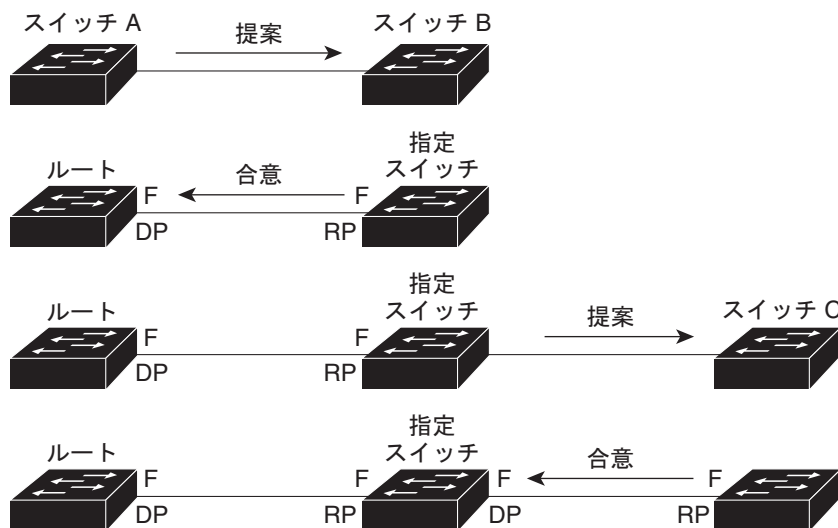
図 17-8 高速コンバージェンスの提案合意ハンドシェイク
