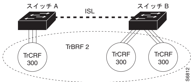
図 12-3 分散型 TrCRF
