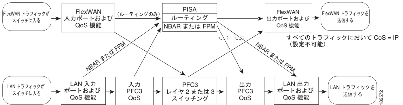
図 38-2 PFC3B でのトラフィック フローおよび PFC QoS 機能
