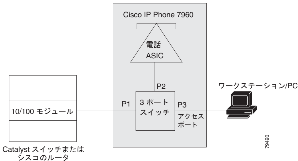
図 14-1 Cisco IP Phone とスイッチの接続
