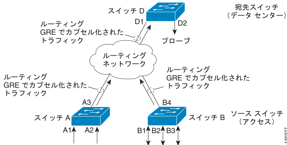
図 48-3 ERSPAN の設定
