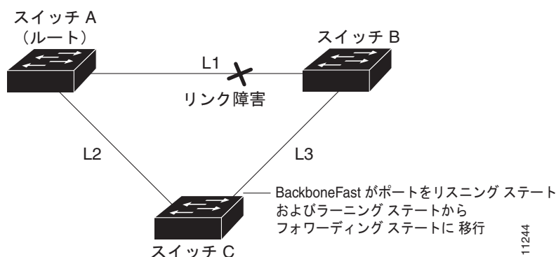
図 18-4 間接リンク障害が発生したあとの BackboneFast の例
