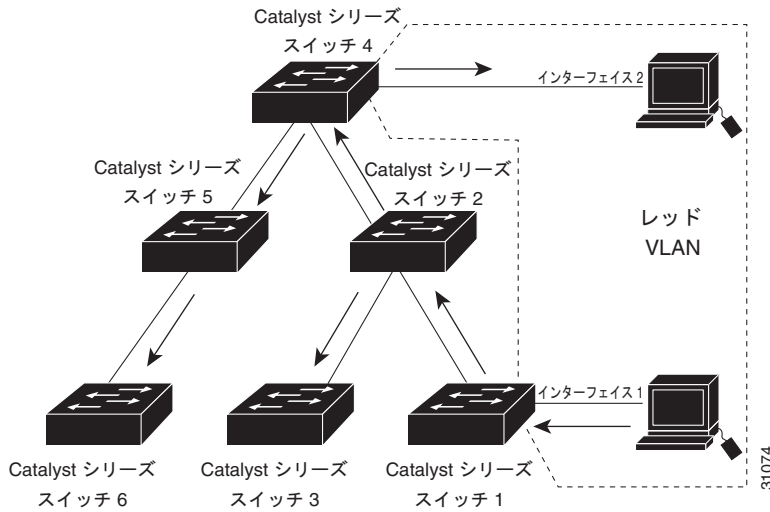
図 11-1 VTP プルーニングを使用しない場合のフラディング トラフィック
