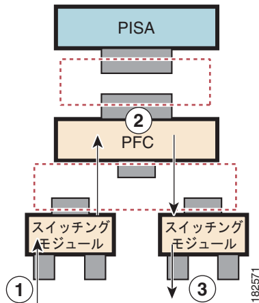
図 38-1 PFC QoS 機能による処理の概要
