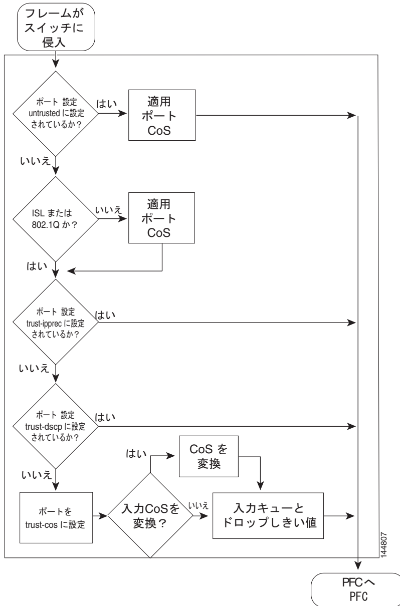
図 38-4 入力 LAN ポートの PFC QoS 機能
