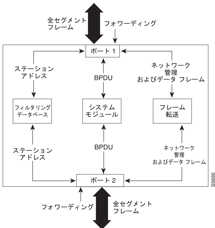
図 17-6 フォワーディング ステートのインターフェイス 2
