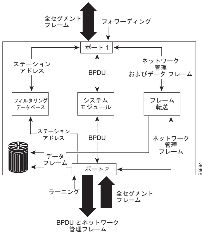
図 17-5 ラーニング ステートのインターフェイス 2
