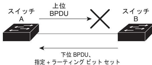
図 17-12 単一方向リンク障害の検出
