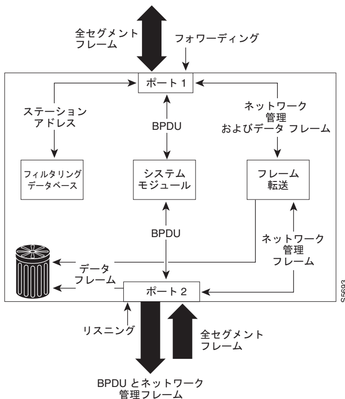
図 17-4 リスニング ステートのインターフェイス 2
