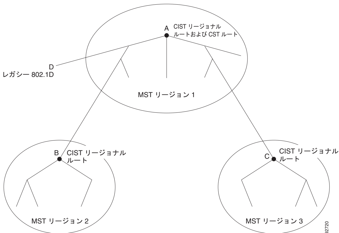
図 17-10 MST 領域、CIST リージョナルルート、および CST ルート
