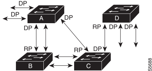
図 17-1 スパニング ツリー トポロジ
