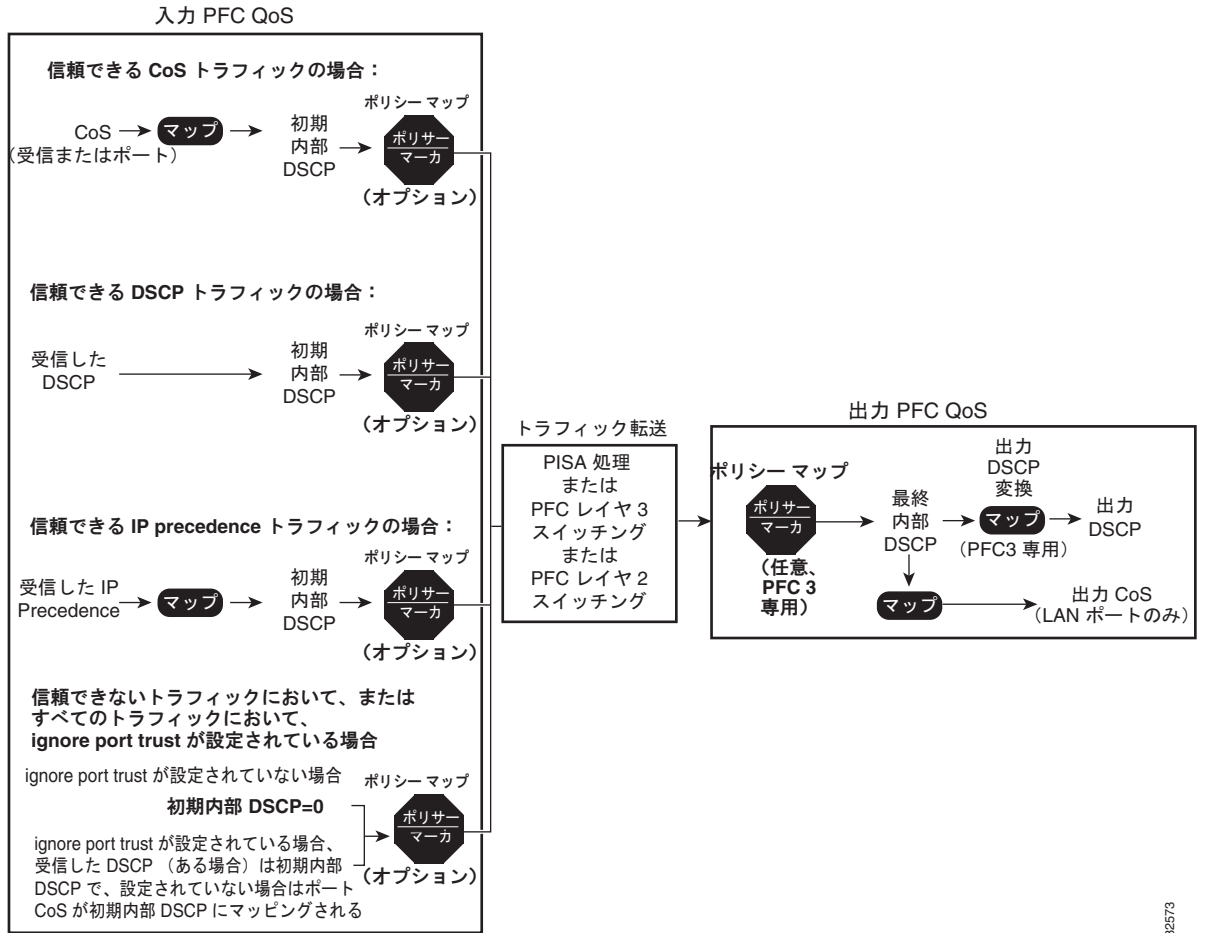
図 38-5 PFC3B の QoS 機能
