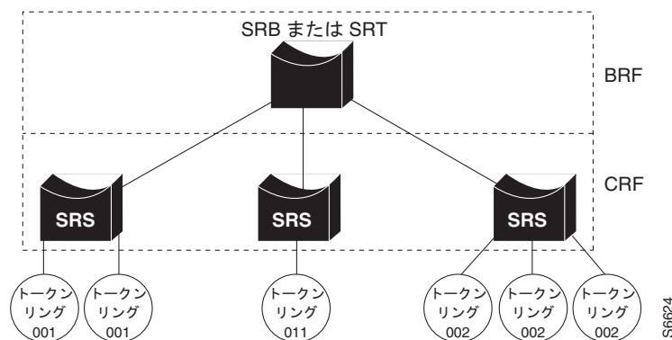
図 12-1 相互接続された TrBRF VLAN および TrCRF VLAN
