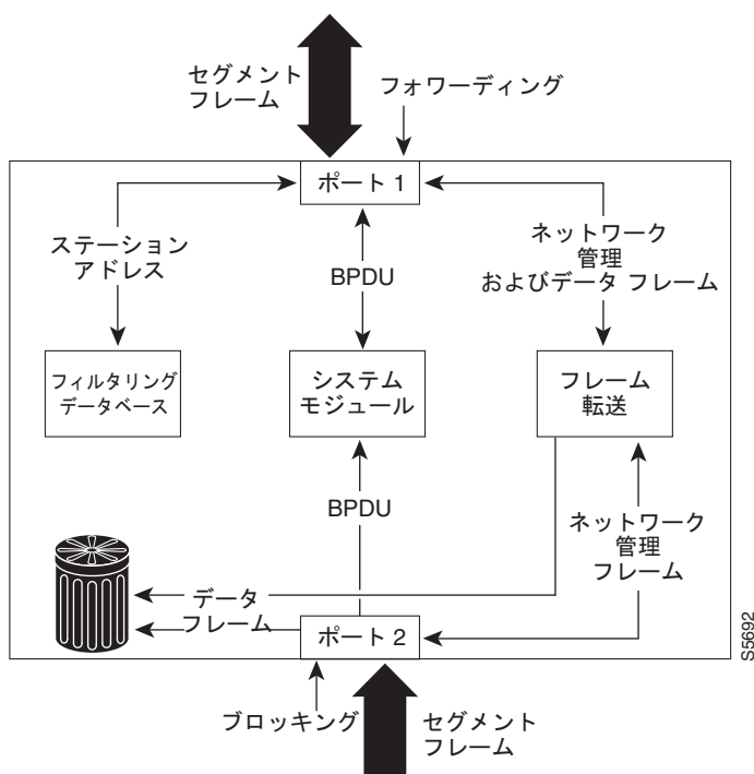
図 17-3 ブロッキング ステートのインターフェイス 2
