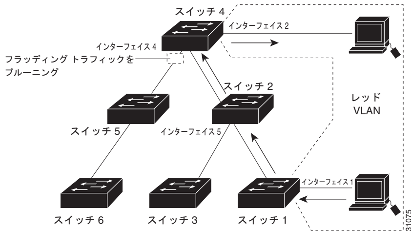
図 11-2 VTP プルーニングを使用した場合のフラディング トラフィック
