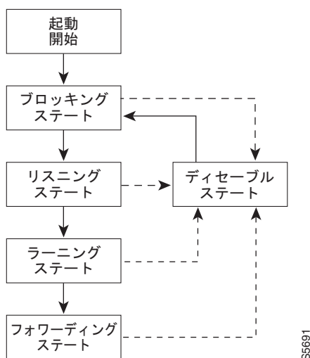
図 17-2 レイヤ 2 LAN インターフェイス ステート
