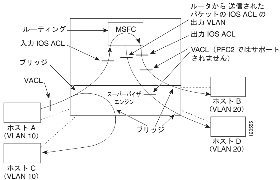
図 32-3 マルチキャスト パケットへの VACL の適用
