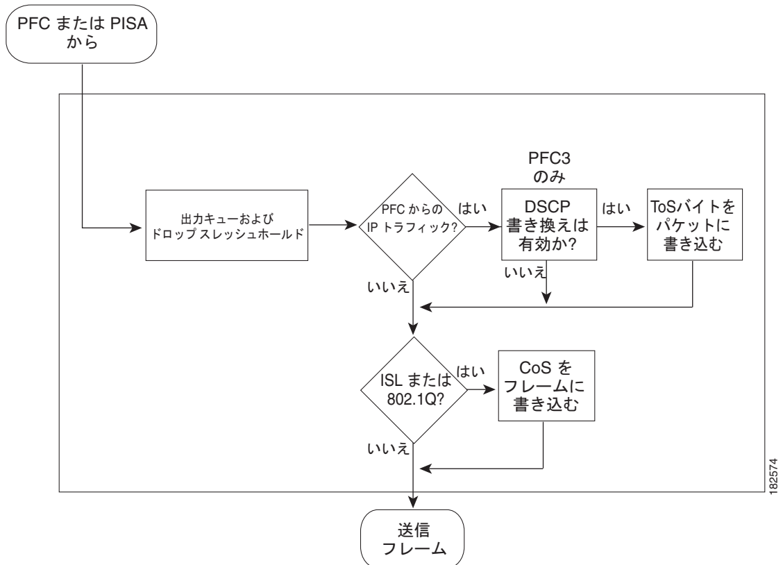
図 38-6 出力 LAN ポートでのスケジューリング、輻輳回避、およびマーキング
