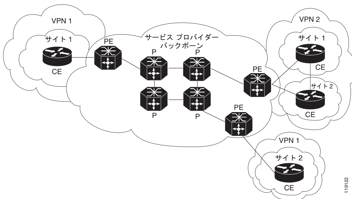
図 21-3 VPN およびサービス プロバイダー バックボーン
