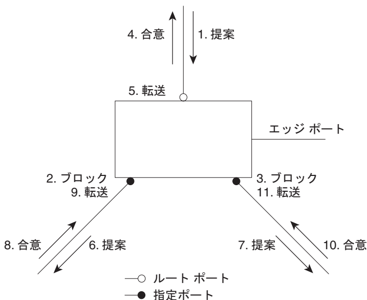
図 17-9 高速コンバージェンス時のイベント シーケンス
