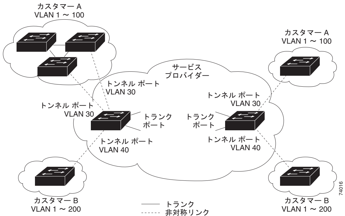
図 15-1 サービスプロバイダーネットワークにおける IEEE 802.1Q トンネルポート
