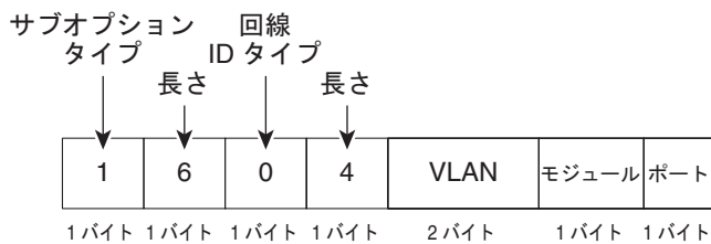
図 34-2 サブオプションの packets 形式
