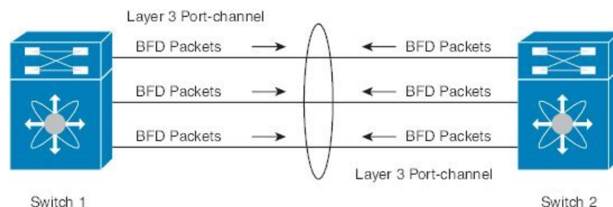
図 42: マイクロ BFD ポートチャネルでのセッション
