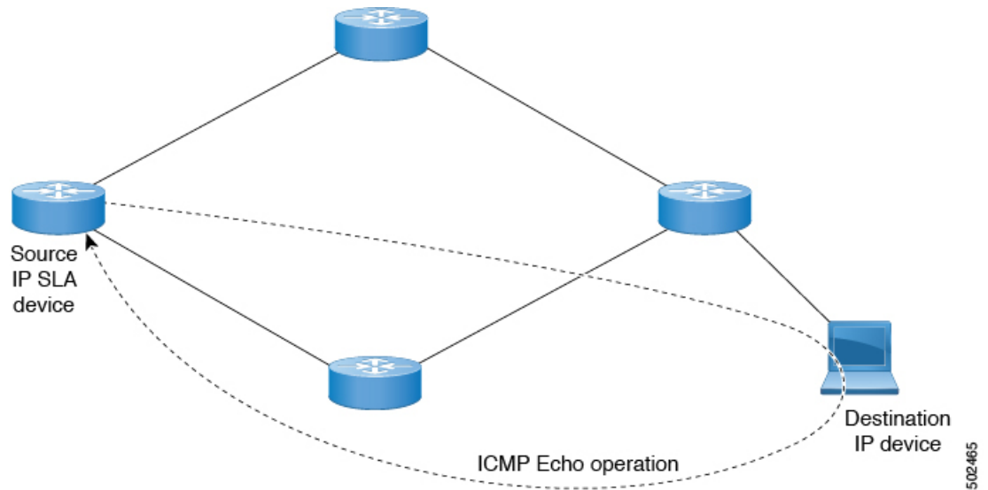
図 59: ICMP エコー動作の例
