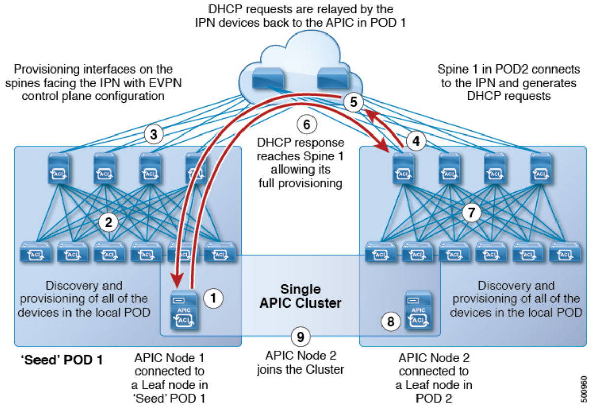
図 11: マルチポッドのプロビジョニング
