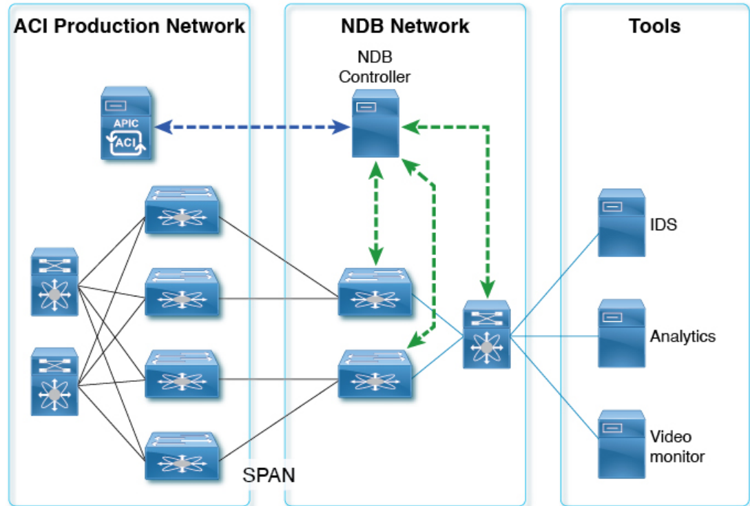
図 10: NDB MPLS ヘッダストリップソリューション
