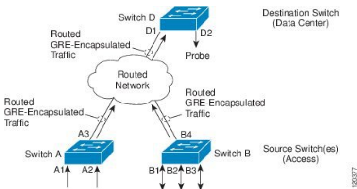
図 1: ERSPAN の設定
