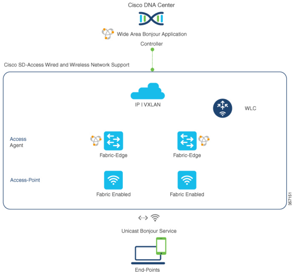
図 41 : Cisco SD-Access ネットワーク設計
