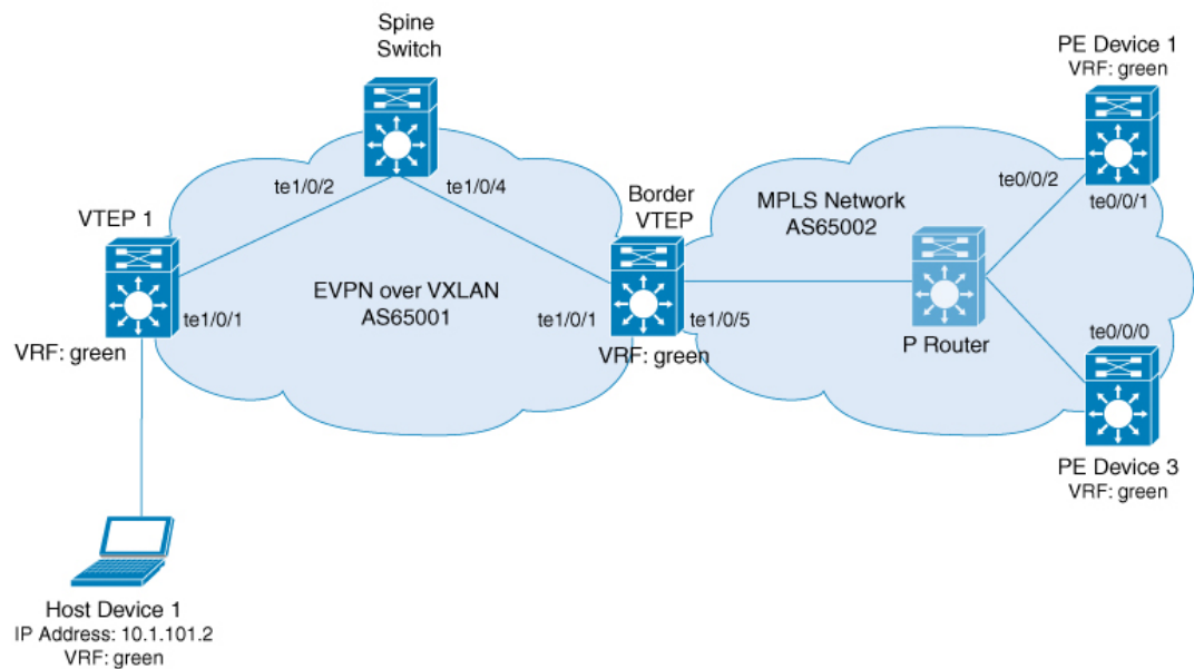
図 32: eBGP を介した MPLS レイヤ 3 VPN とのレイヤ 3 外部接続
