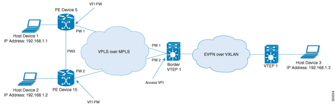
図 30: アクセス VFI を介した VPLS ネットワークとのレイヤ 2 外部接続
