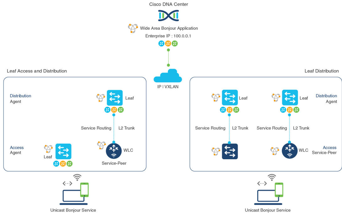
図 51: BGP EVPN VXLAN を介した Wide Area Bonjour の導入モデル
