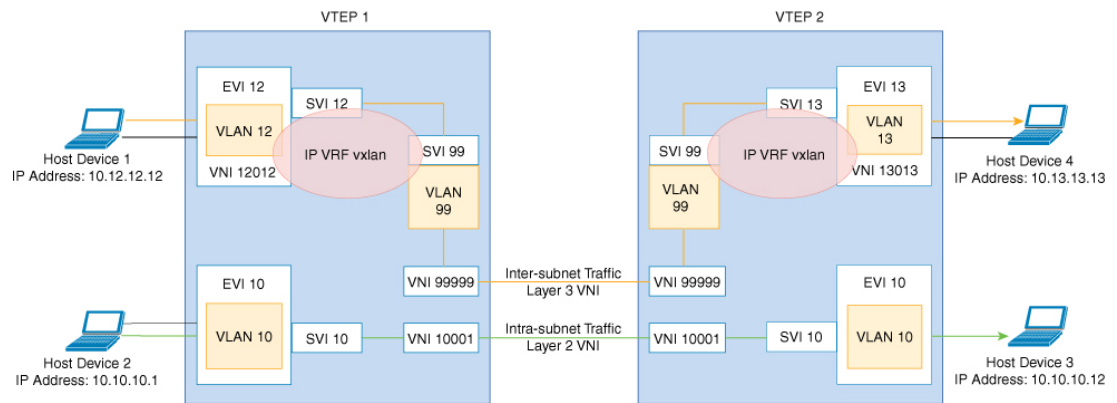
図 34: レイヤ2とレイヤ3のVNIを介したEVPN VXLANネットワークでのトラフィックの移動
