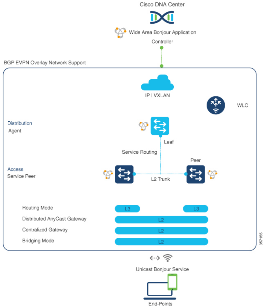
図 44: L2スイッチをアップストリーム BGP EVPN リーフスイッチに接続する mDNS エンドポイント
