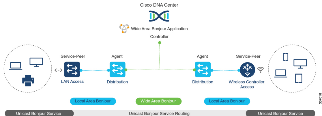
図 37: Cisco Wide Area Bonjour ソリューション
