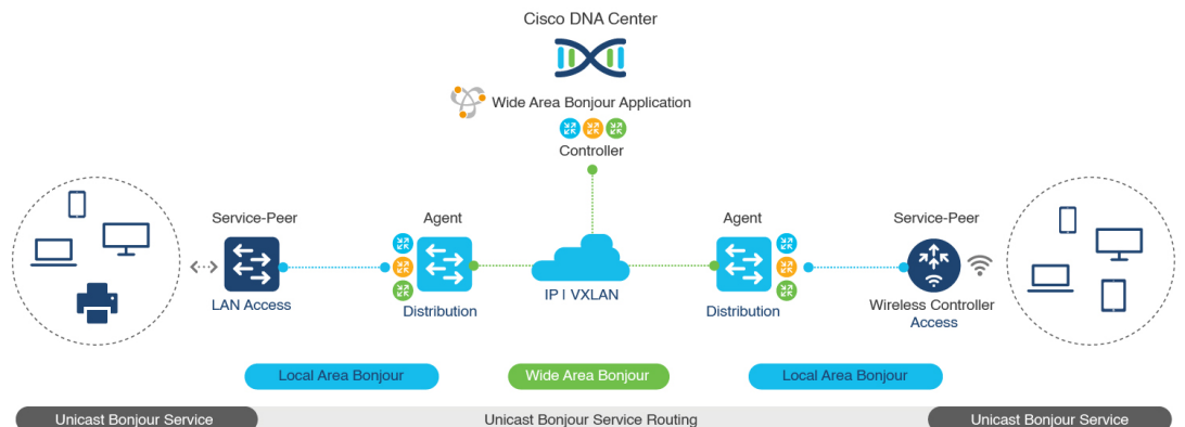
図 43: BGP EVPN 対応エンタープライズネットワークのオーバーレイ Bonjour サービス
