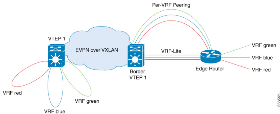
図 27: VRF-Lite を使用したレイヤ 3 外部接続
