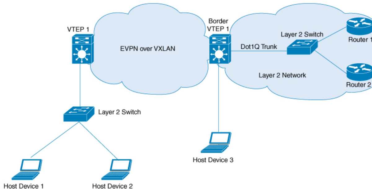
図 29: IEEE 802.1Q ネットワークとのレイヤ 2 外部接続
