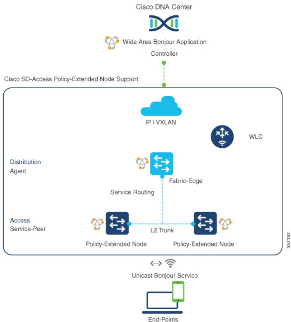
図 42: ファブリック対応ポリシー拡張ノード
