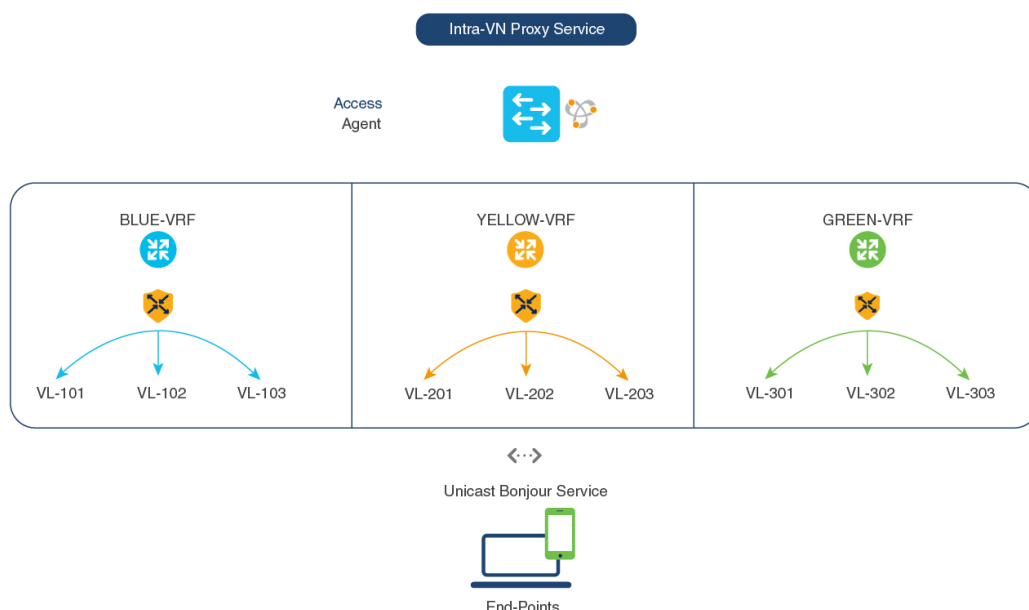
図 56: VN 間サービスプロキシ
