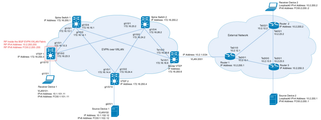
図 23：RPがBGP EVPN VXLANファブリック内にある場合のPIM-SMでのTRM
