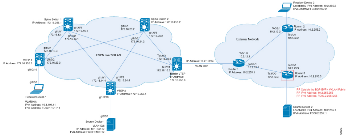
図 24：RP が BGP EVPN VXLAN ファブリックの外部にある場合の PIM-SM での TRM
