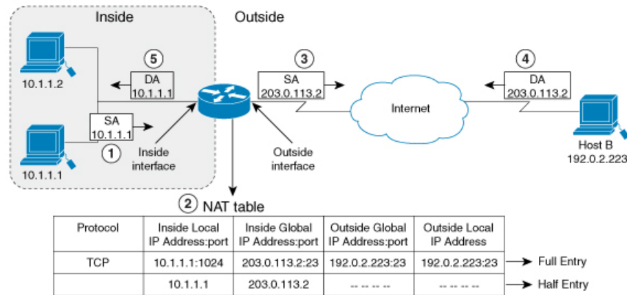
図 2: NAT 内部送信元変換
