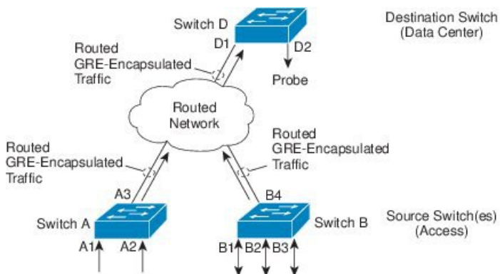
図 8: ERSPAN の設定
